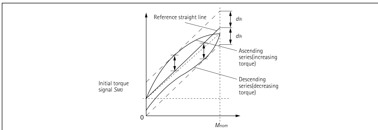
図5 ヒステリシスを含む直線性 d_{lh}
