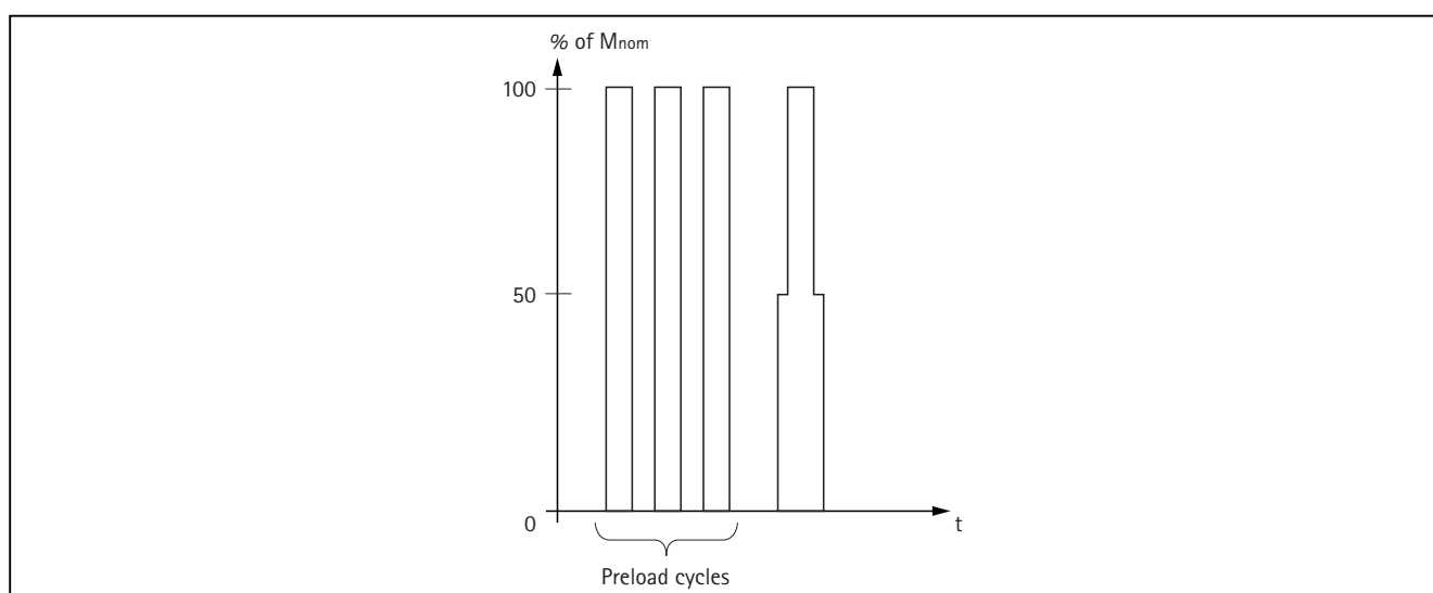
図9 DIN 1319に定義されている校正負荷サイクルの例 (ページ9の参照図)
