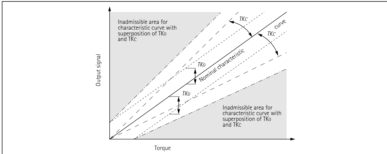
図2 感度に対する温度影響 ( TK_c ) およびゼロ点に対する温度影響 ( TK_o )
