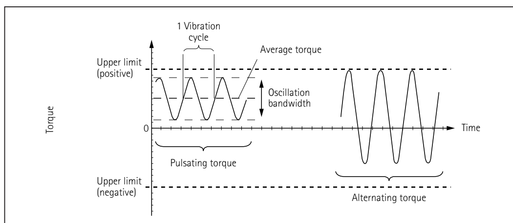
図7 振動振幅（Oscillation bandwidth）に関する用語
