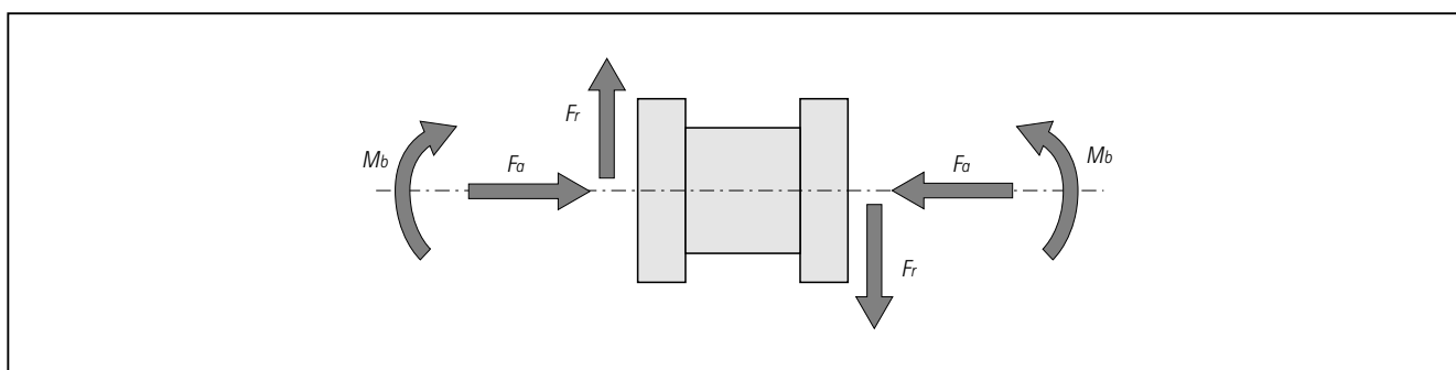
図8 寄生負荷 (parasitic loads): 軸方向力 F_a , 横力 F_r , 曲げモーメント M_b
