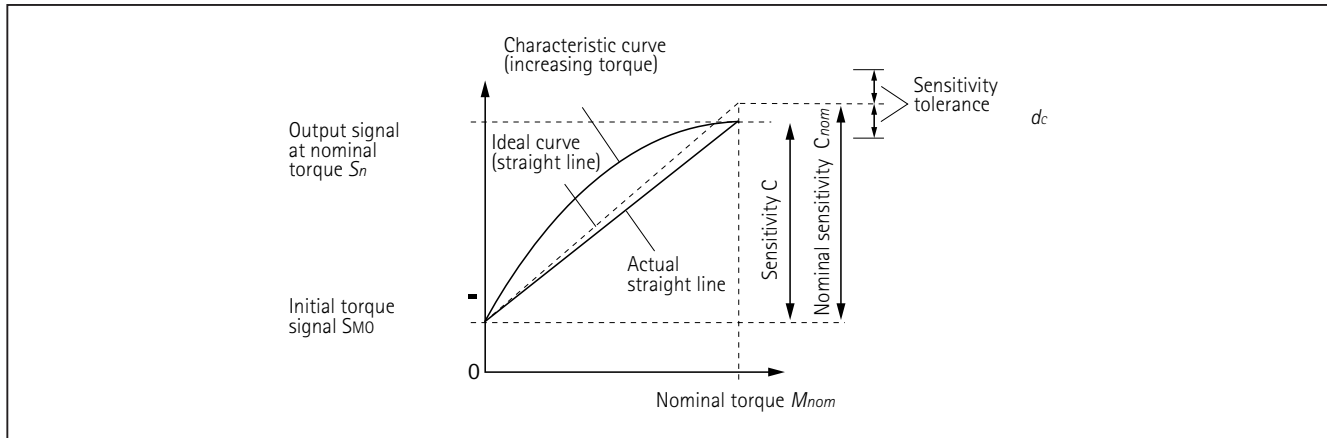
図1 感度と公称トルクの関係
