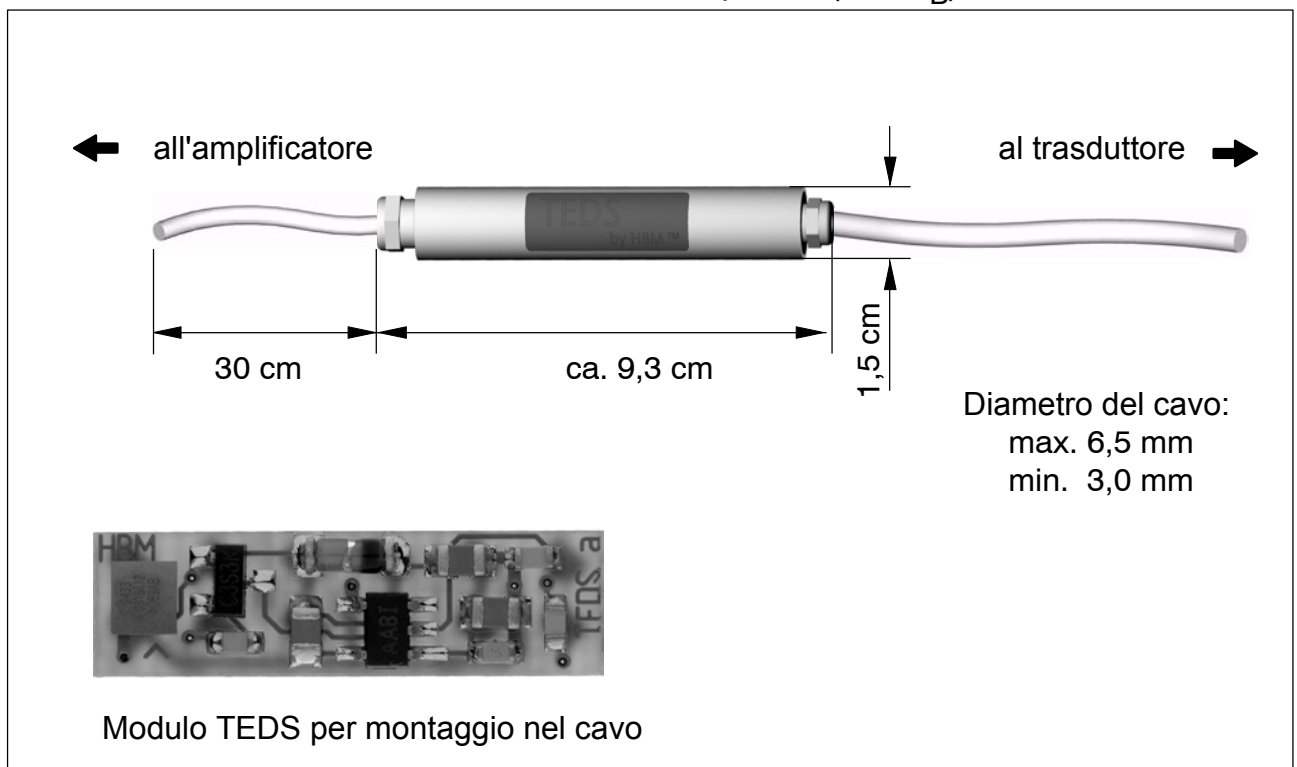
Fig. 3.3: Dimensioni del modulo TEDS già montato
