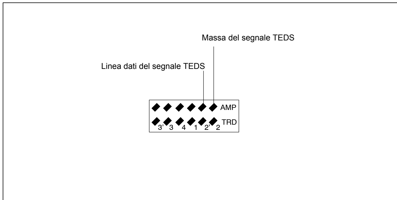
Fig. 3.4: Connessione all'amplificatore di misura con due fili separati
