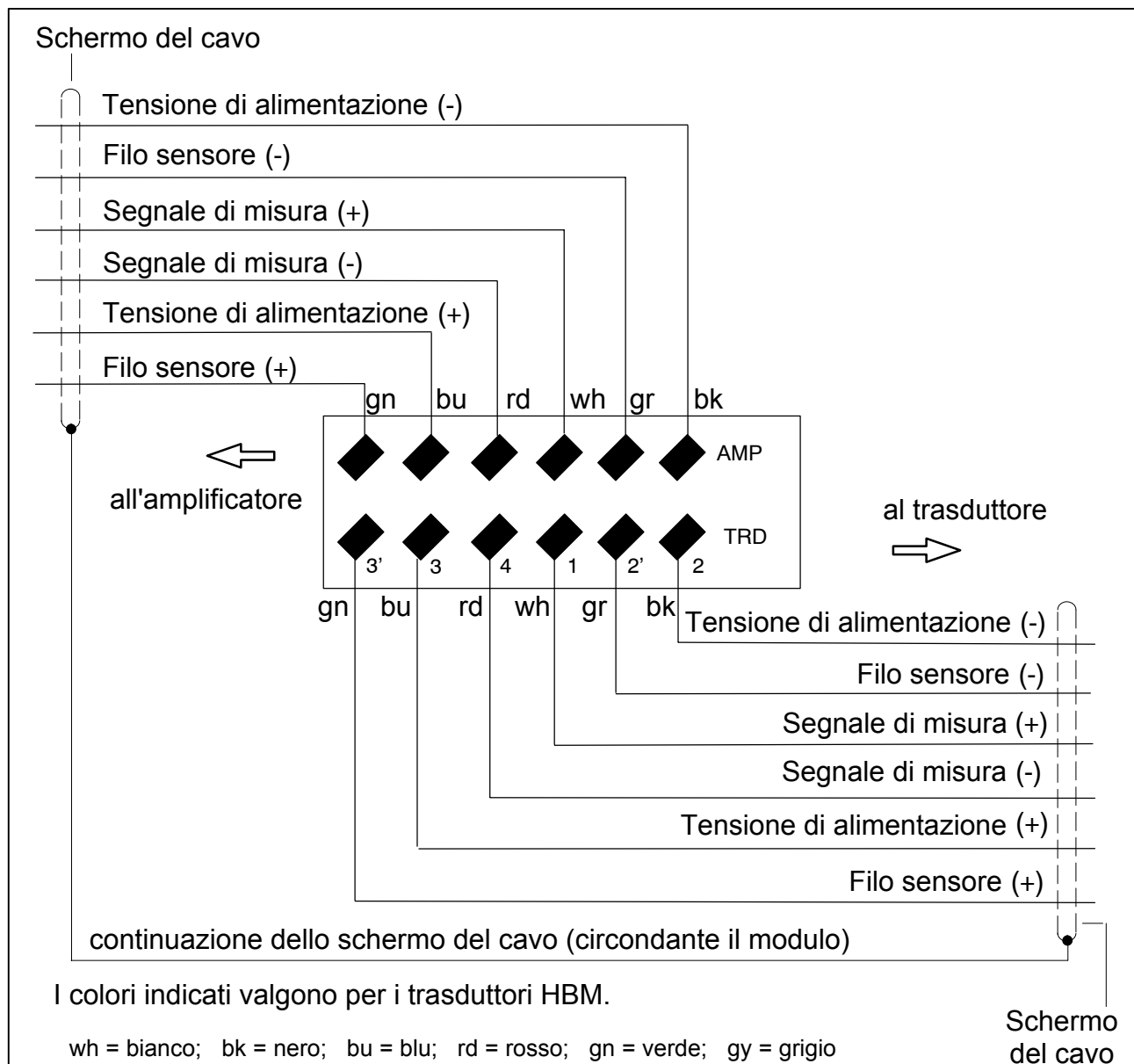
Fig. 3.2: Modulo 1-TEDS-BOARD-S
