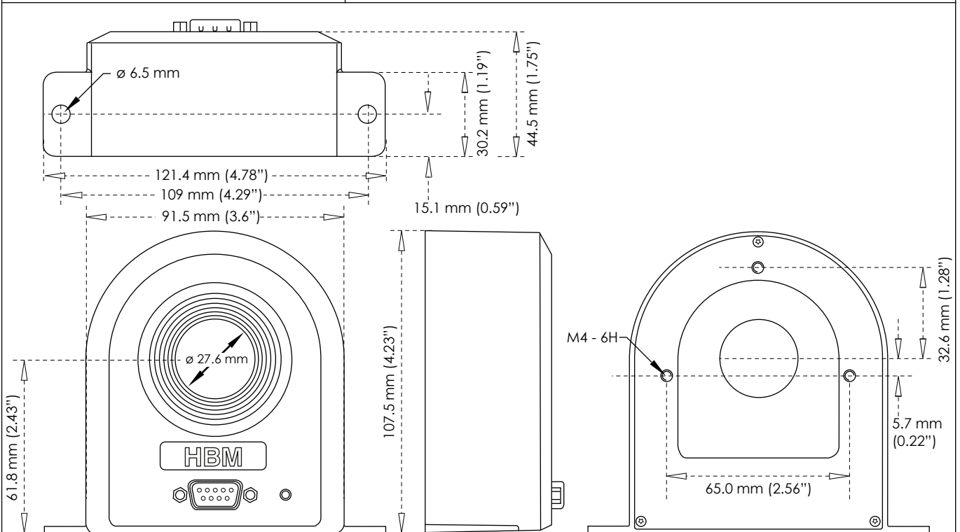
그림 1.5: CTS50/200ID/400ID/600ID 치수
