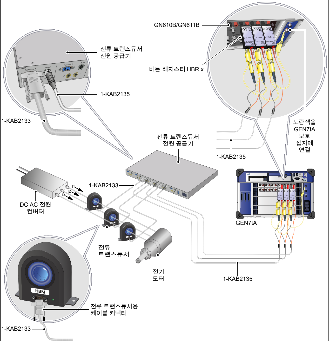
그림 1.9: 전류 트랜스듀서 연결도
