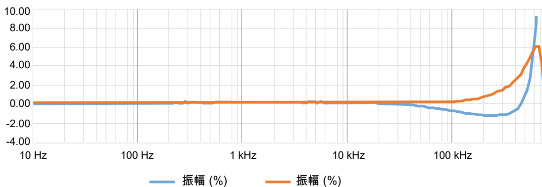
図 1.3: 周波数特性
