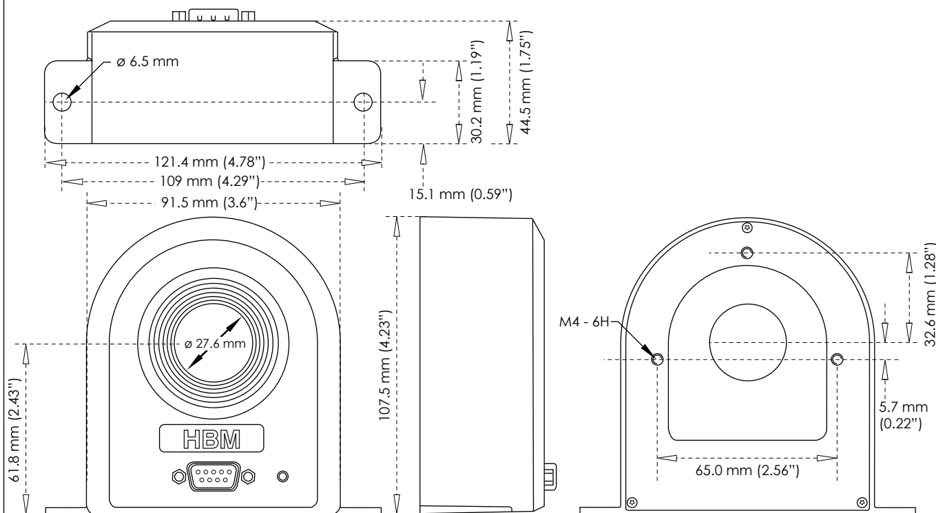
図 1.5: CTS50/200ID/400ID/600ID の寸法
