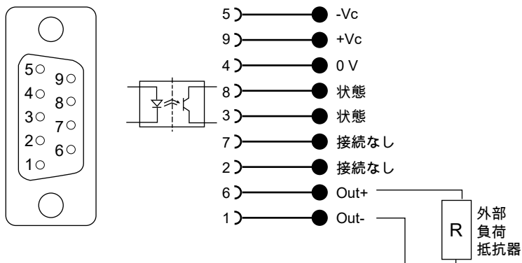
図 1.4: 標準 D-SUB 9 電流出力
