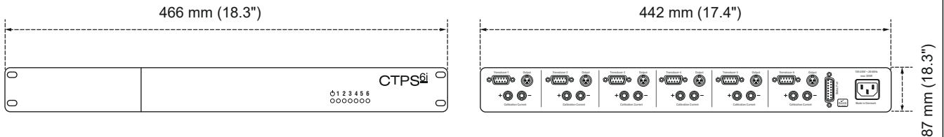
그림 1.7: 치수
