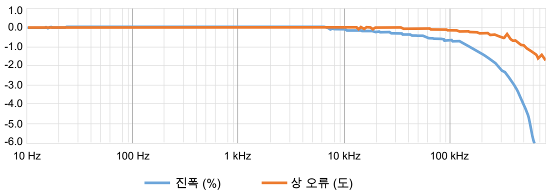
그림 1.3: 주파수 특성
