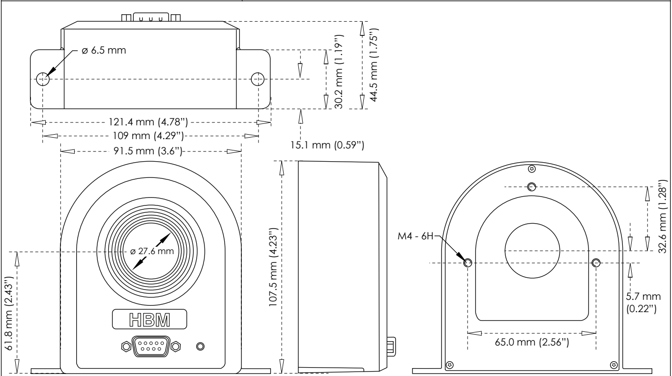
그림 1.5: CTS50/200ID/400ID/600ID 치수
