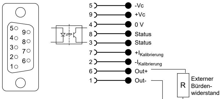
Abbildung 1.4: Stromausgang am 9-poligen D-SUB-Standardstecker
