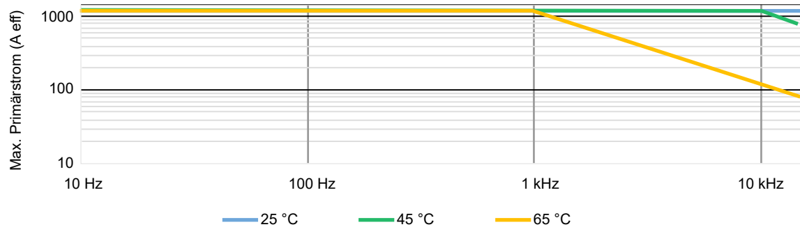
Abbildung 1.2: Herabsetzung der Nennwerte durch Frequenz und Umgebungstemperatur
