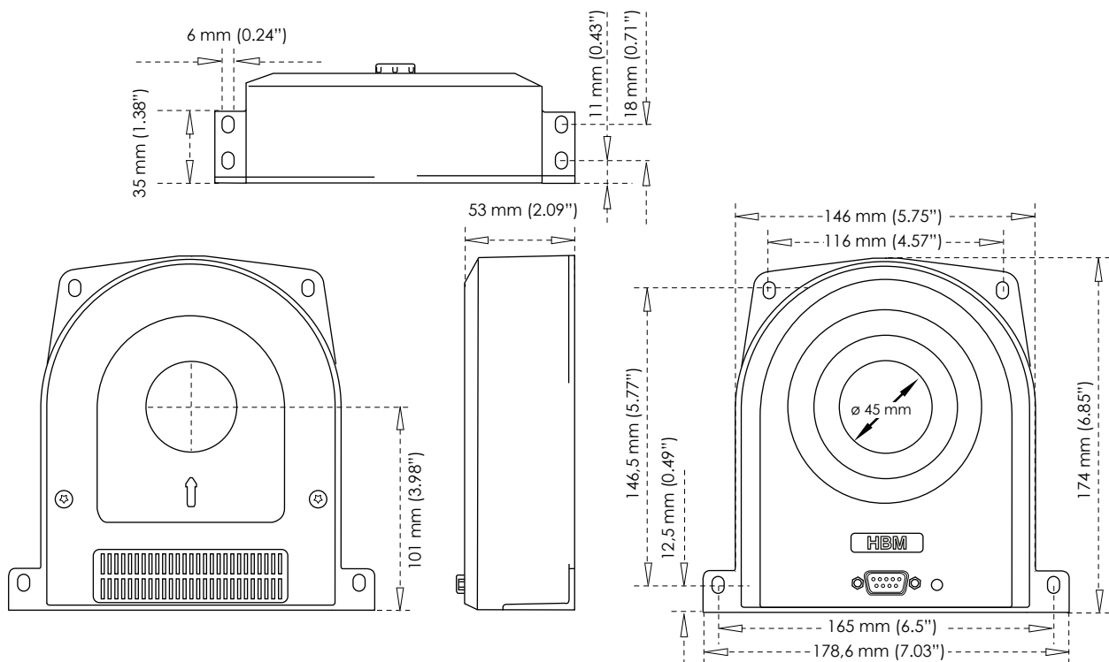
Abbildung 1.5: Abmessungen CTM1200ID/CTM1200ID-CD3000
