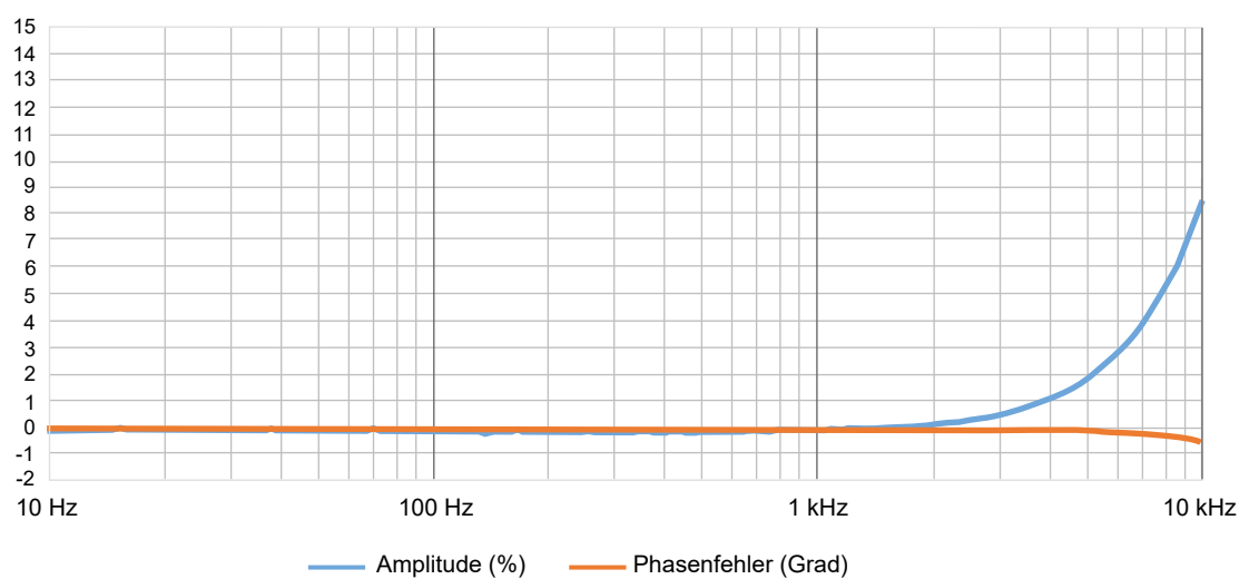
Abbildung 1.3: Frequenzkennlinie
