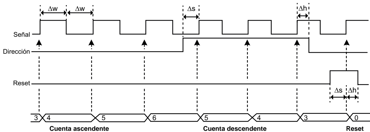
Figura 30: Reloj unidireccional y bidireccional
