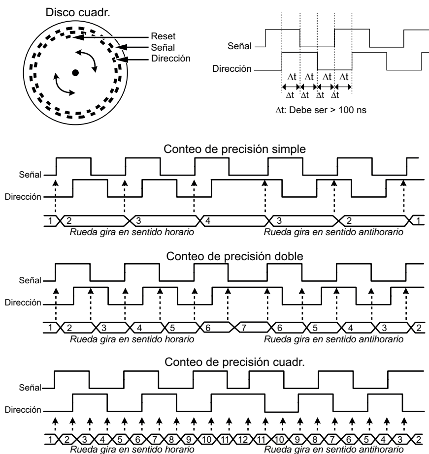
Figura 31: Modos de conteo bidireccional en cuadratura
