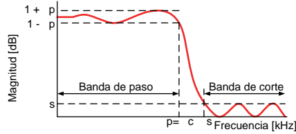
Figura 24: Filtro Elíptico IIR digital
