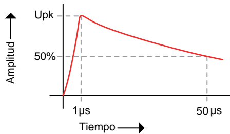
Figura 9: Ejemplo de impulso de 1,2/50 μs
