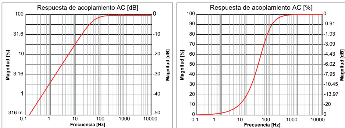
Figura 4: Representación de la respuesta de acoplamiento AC
