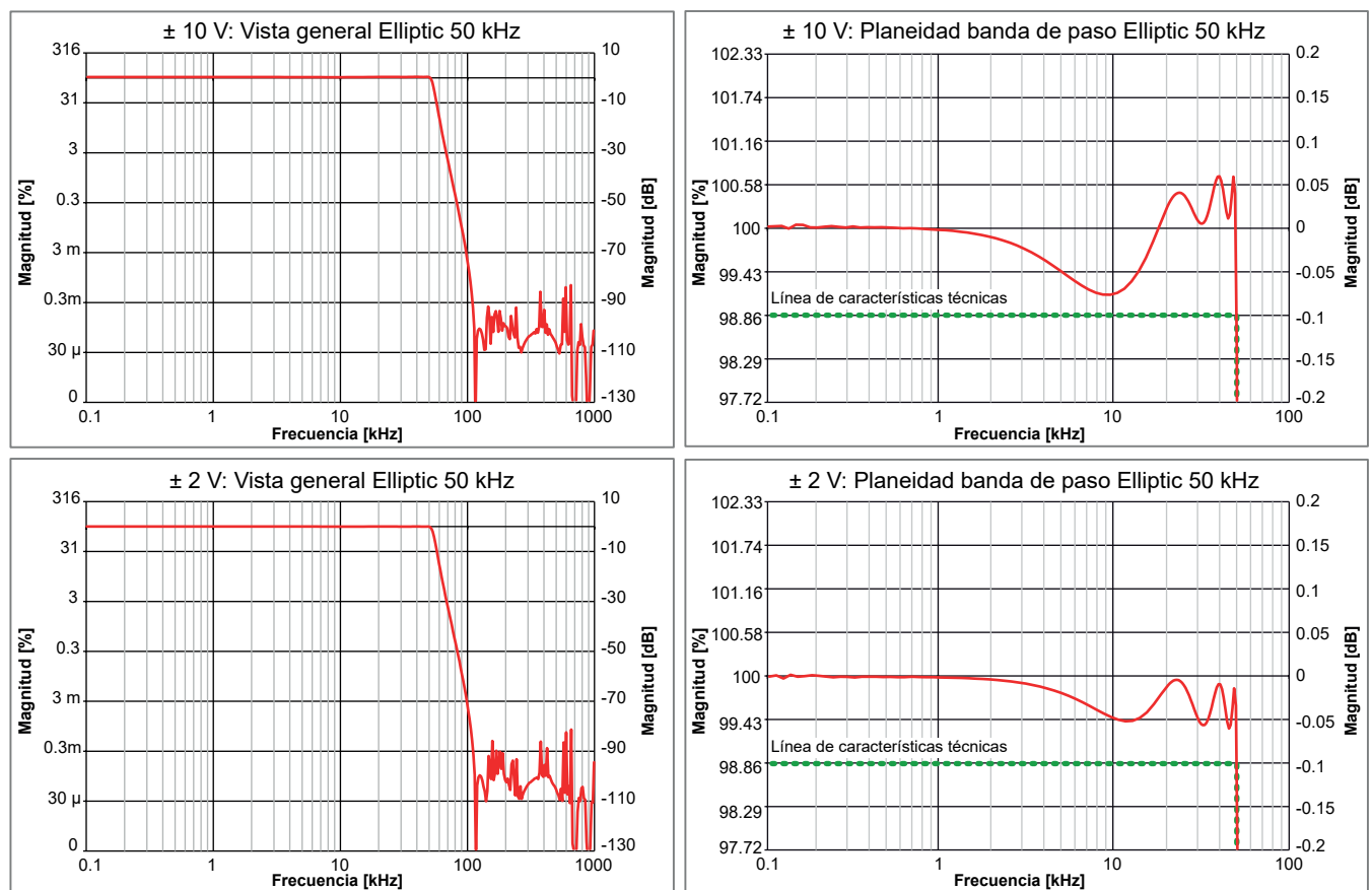
Figura 27: Ejemplos de filtros Elíptico IIR
