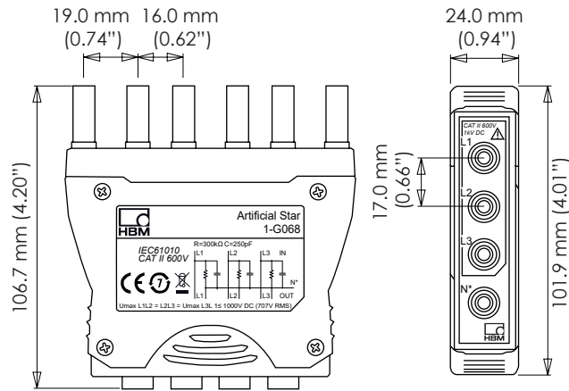
Figura 40: Adaptador de estrella artificial
