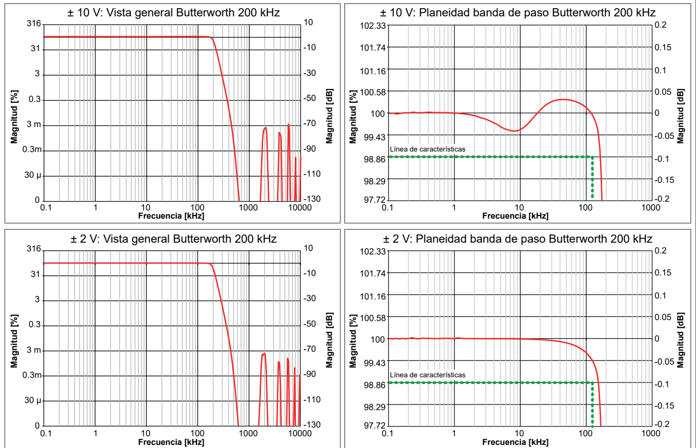
Figura 21: Ejemplos representativos de Butterworth IIR
