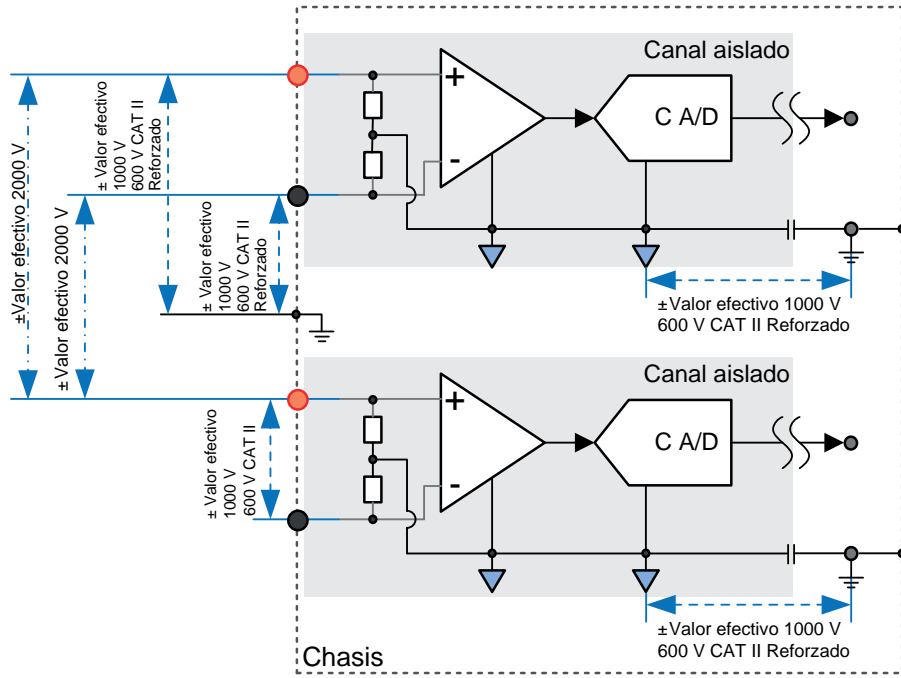
Figura 8: Vista del aislamiento de la tarjeta de 1kV
