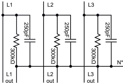
Figura 39: Diagrama de conexiones eléctricas
