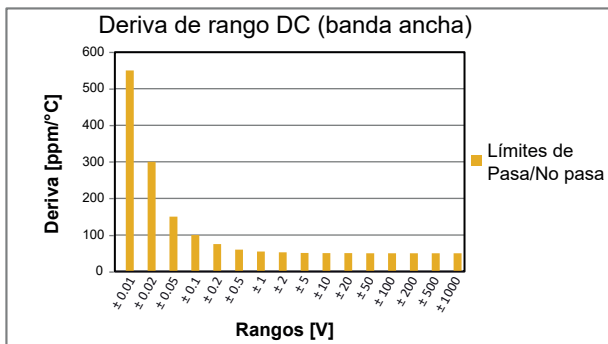
Figura 6: Especificaciones de tensión banda ancha
