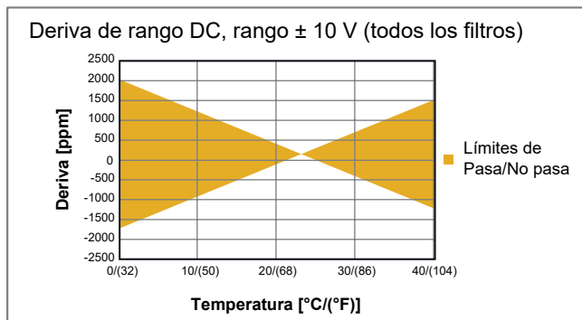
Figura 7: Especificaciones de tensión con todos los filtros usados
