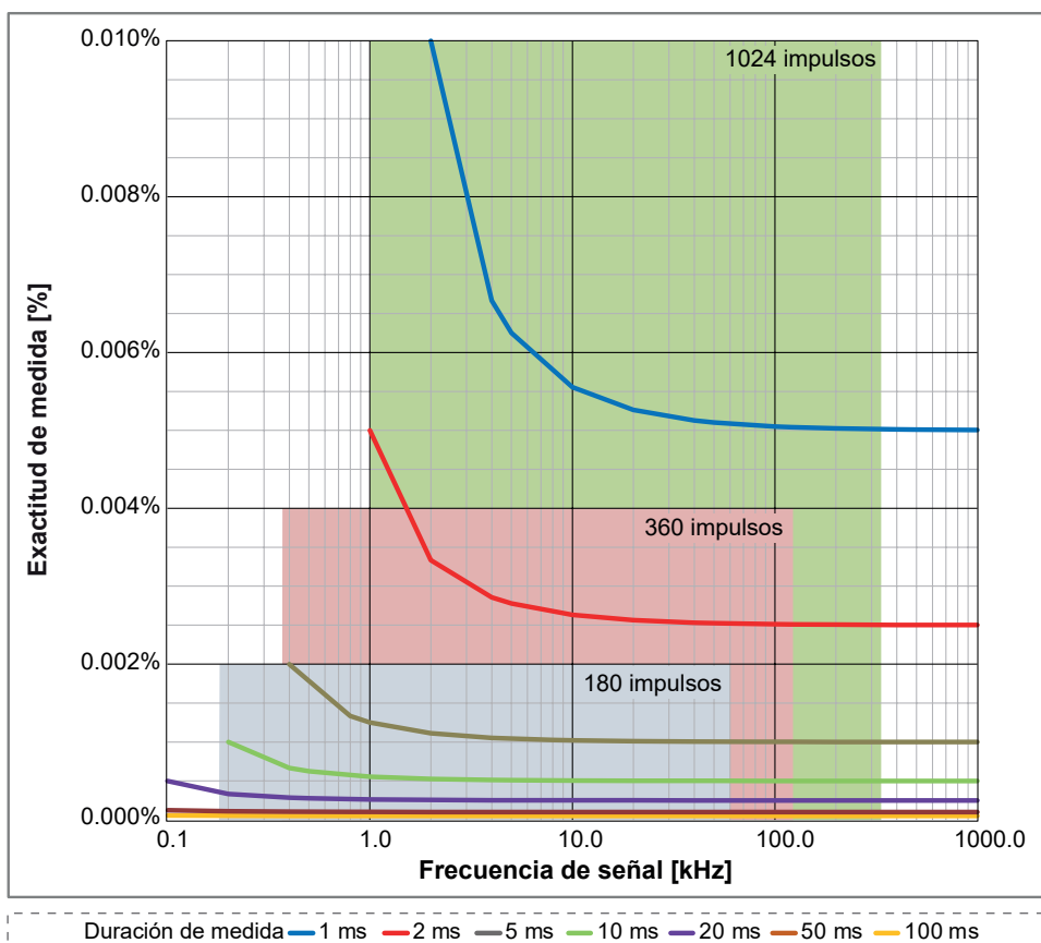
Figura 35: Rango operativo de transductor de velocidad vs. inexactitud y duración de medida
