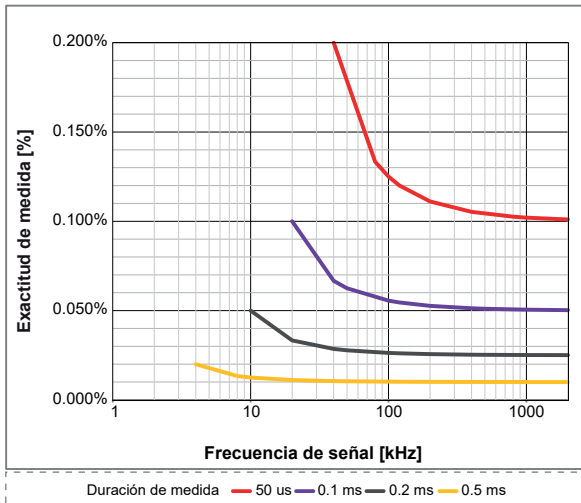
Figura 33: Inexactitud máx. de temporizador
