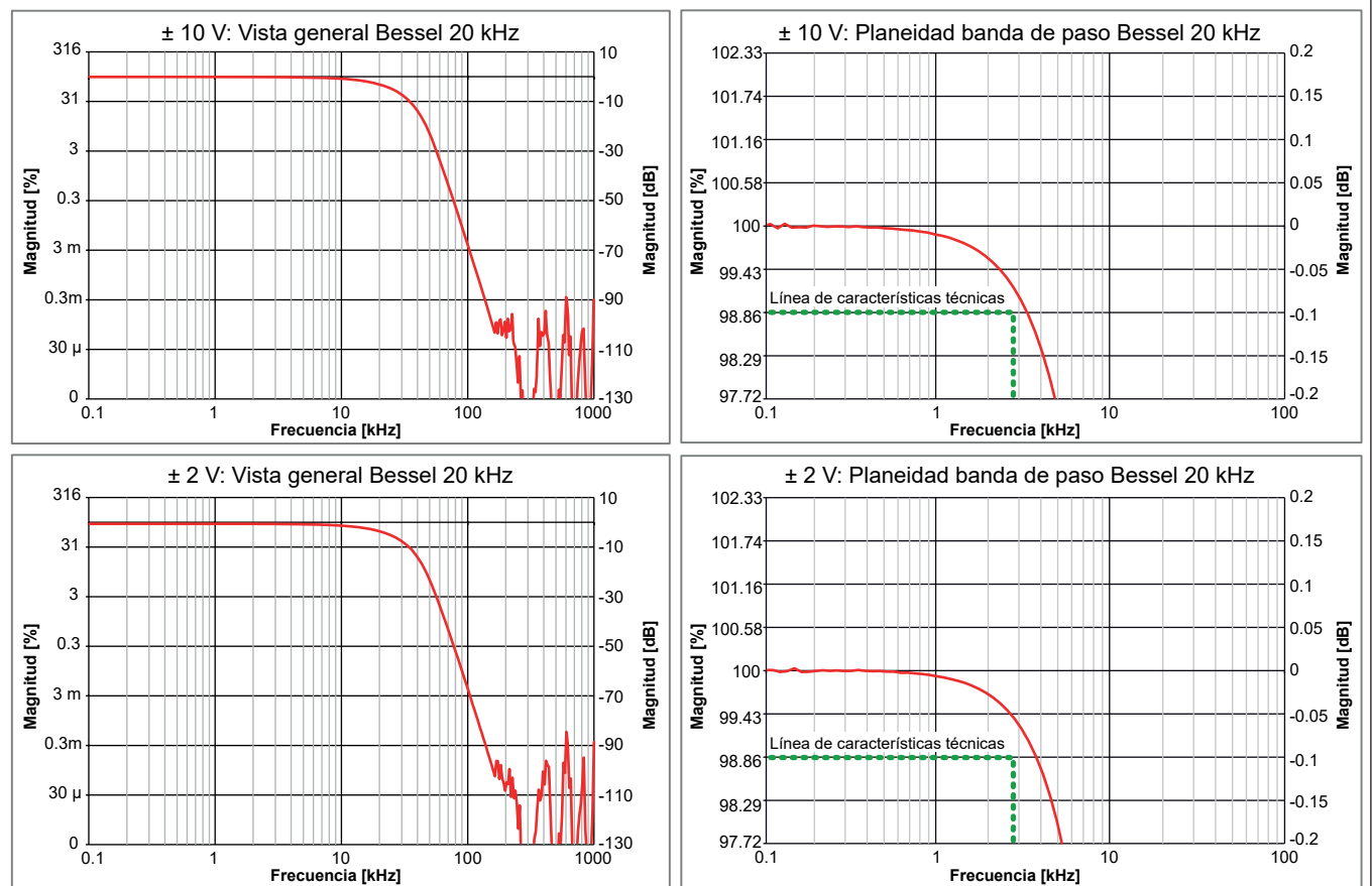
Figura 19: Ejemplos de filtros Bessel IIR
