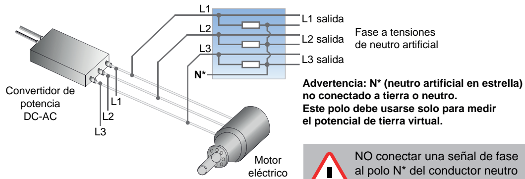
Figura 41: Representación de la utilización del adaptador de estrella artificial con tres fases
