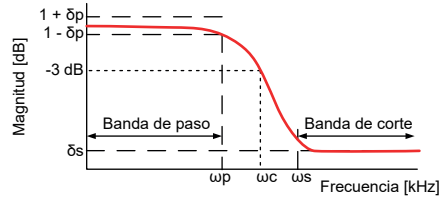
Figura 14: Filtro Butterworth
