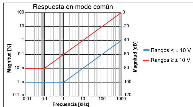
Figura 5: Representación de la respuesta en modo común
