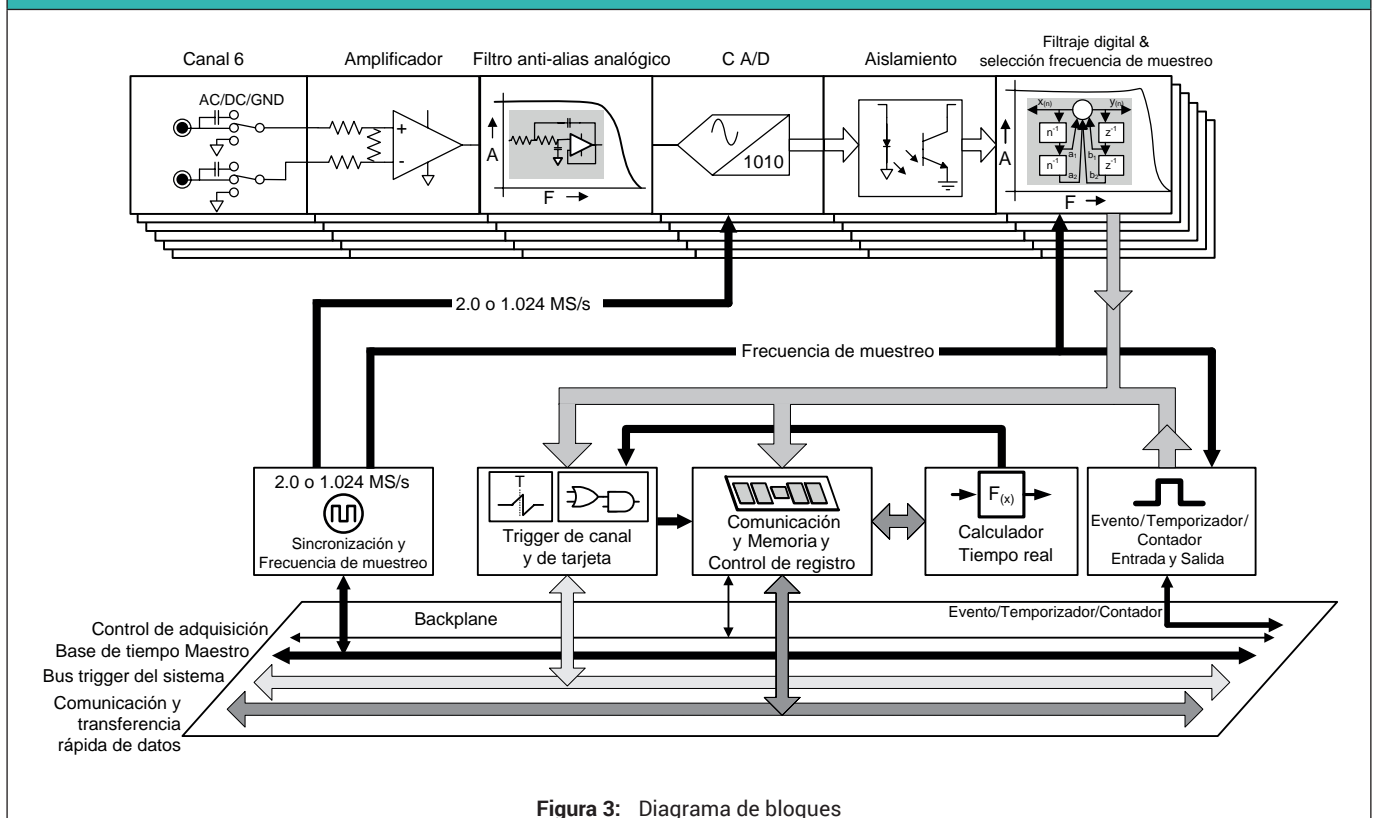
Figura 3: Diagrama de bloques
