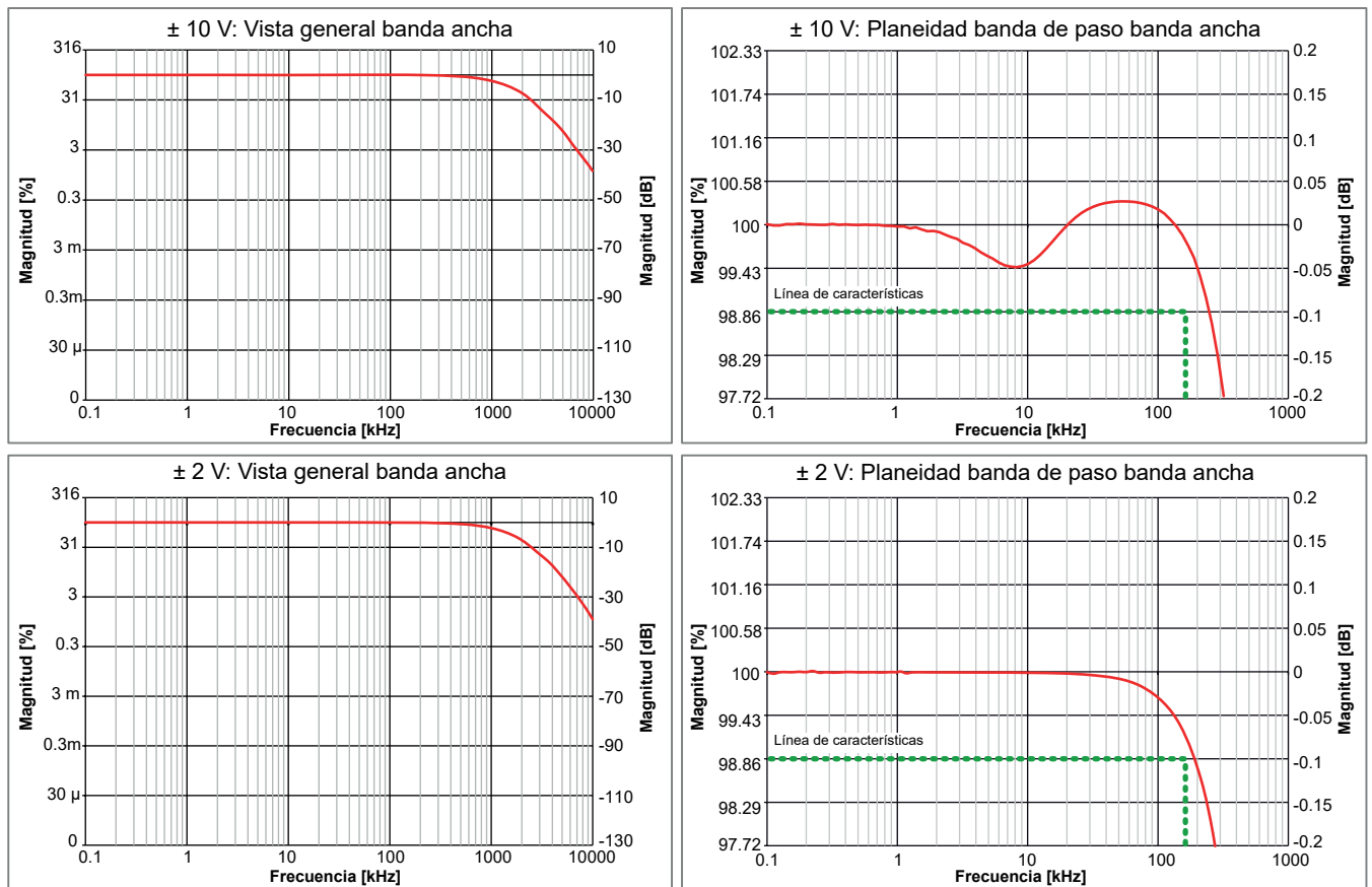
Figura 11: Ejemplos representativos de filtros de banda ancha
