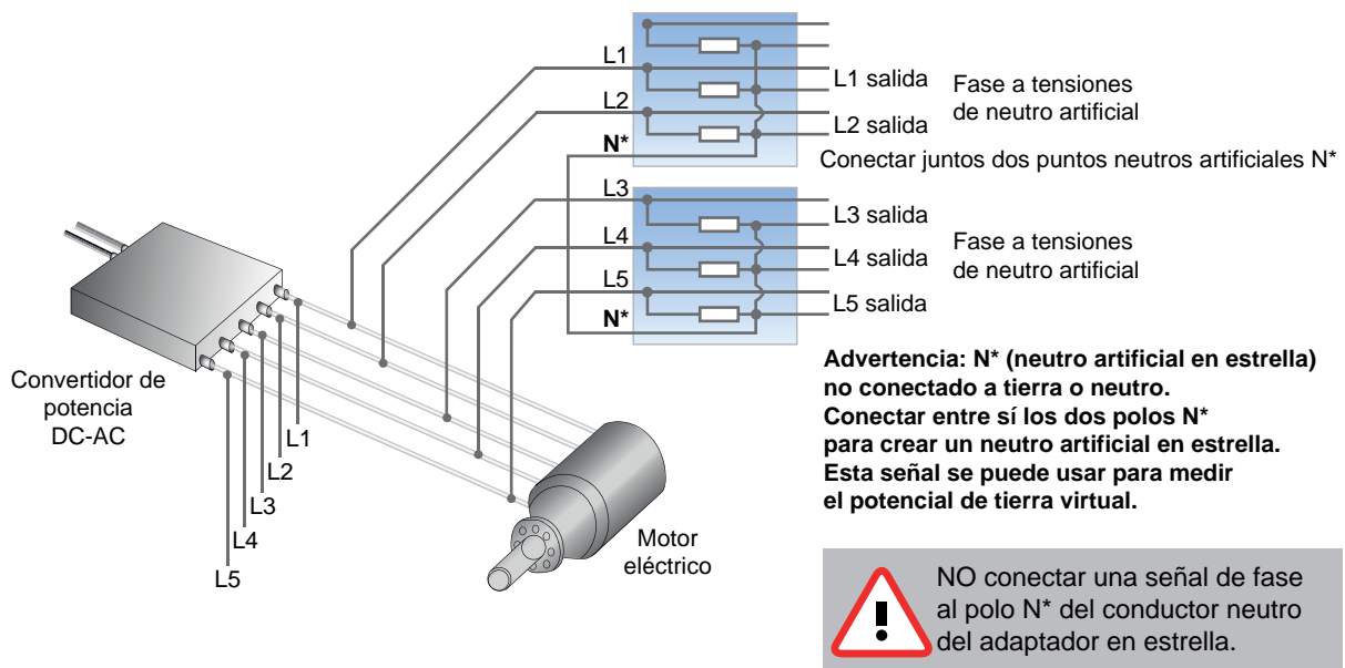
Figura 42: Representación de la utilización del adaptador de estrella artificial con 5 fases o más
