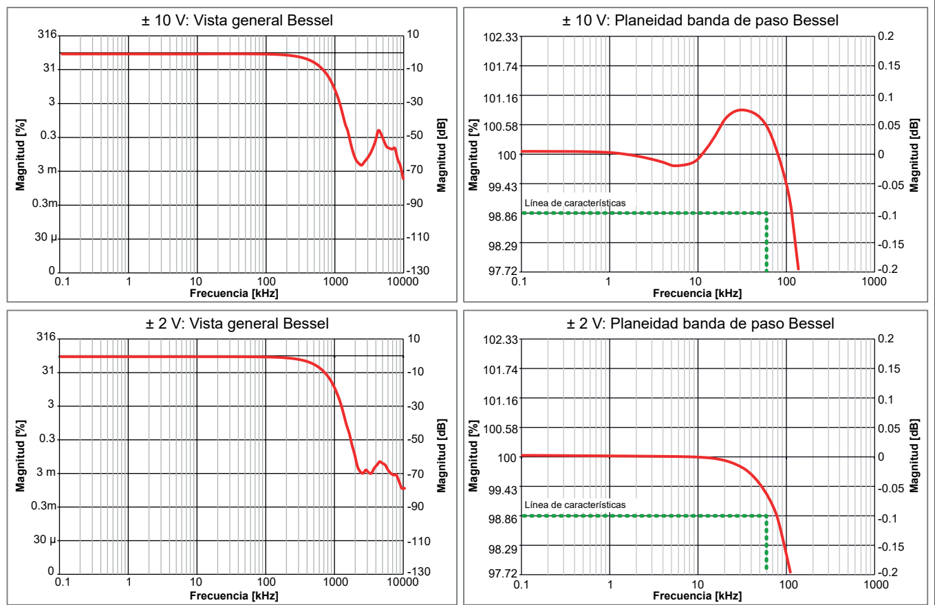
Figura 13: Ejemplos representativos Bessel
