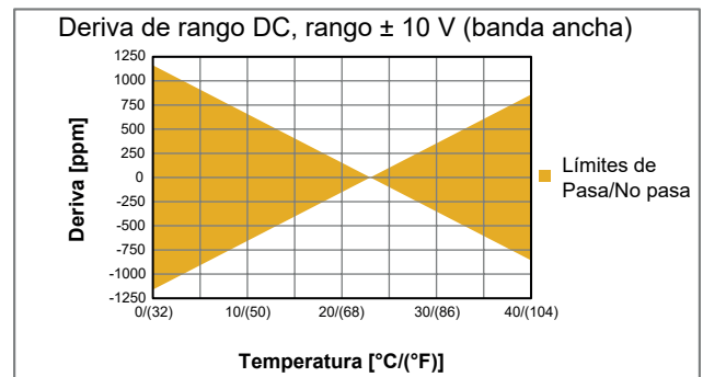
Figura 6: Especificaciones de tensión banda ancha
