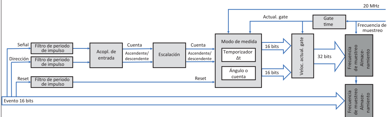
Figura 29: Diagrama de bloques Temporizador/Contador
