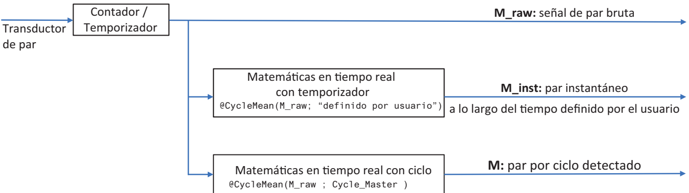
Figura 36: Cálculos simultáneos de par exacto y par dinámico
