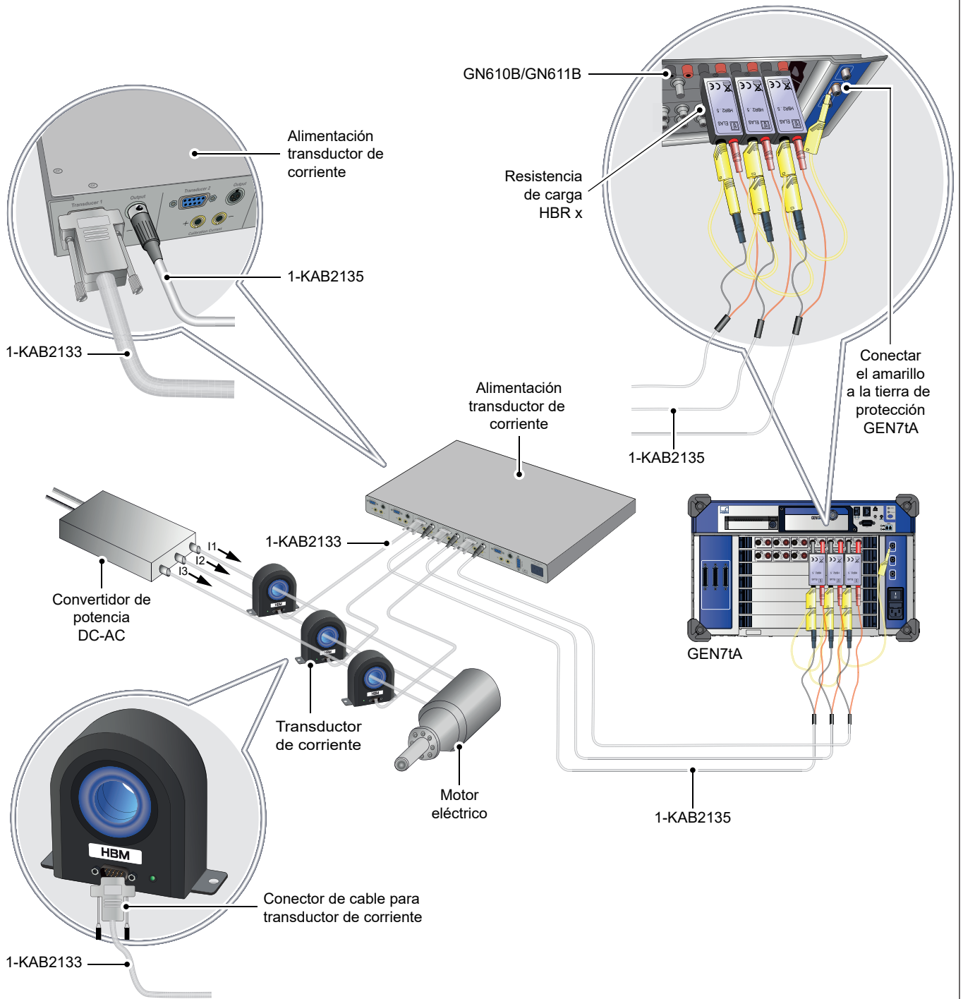
Figura 43: Diagrama de conexiones del transformador de corriente
