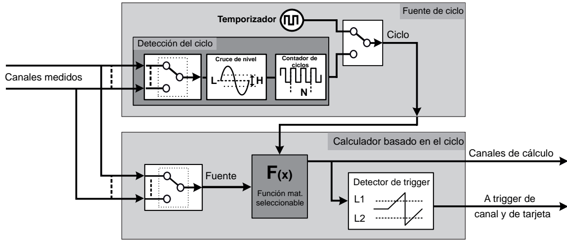
Figura 37: Calculadores en tiempo real basados en el ciclo
