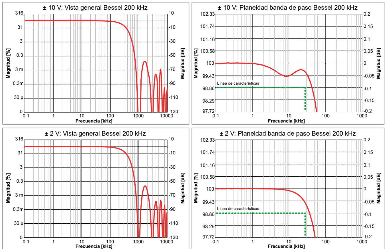
Figura 17: Ejemplos de filtros Bessel IIR
