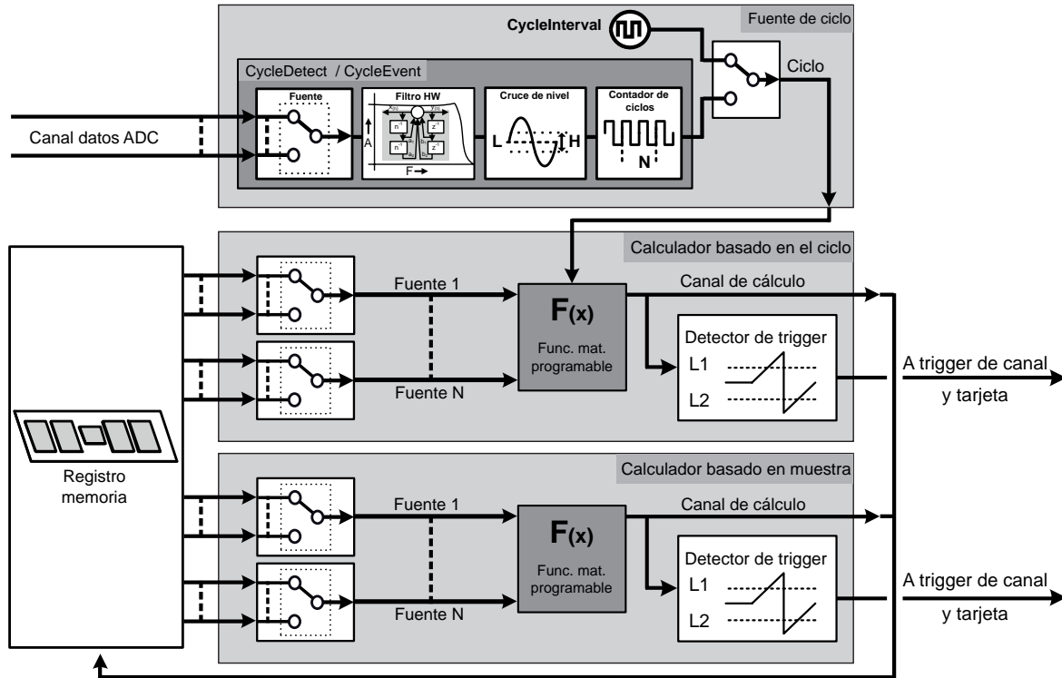
Figura 38: Calculadores en tiempo real asociados a base de datos de fórmulas (RT-FDB)
