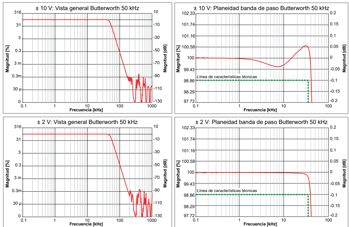
Figura 23: Ejemplos representativos de Butterworth IIR
