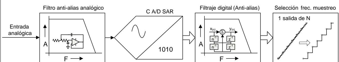
Figura 10: Diagrama de bloques de filtros anti-alias analógicos y digitales combinados
