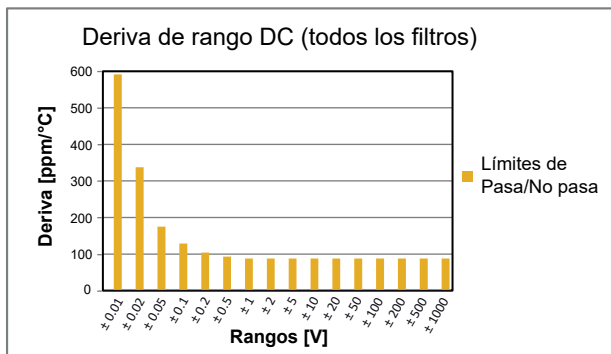
Figura 7: Especificaciones de tensión con todos los filtros usados
