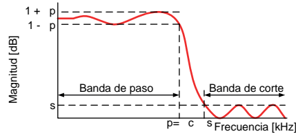
Figura 26: Filtro Elíptico IIR digital
