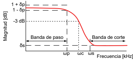
Figura 12: Filtro Bessel
