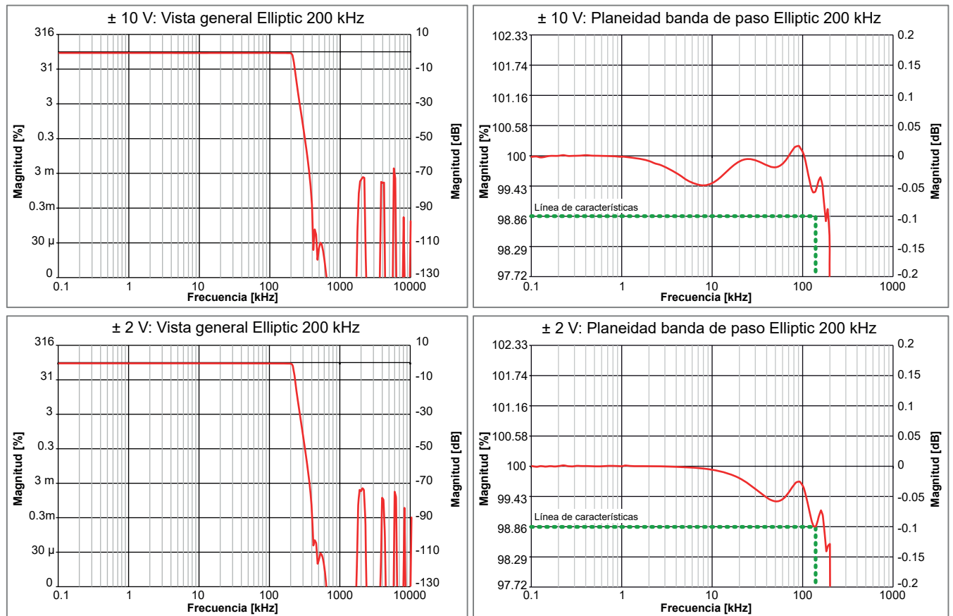
Figura 25: Ejemplos de filtros Elíptico IIR
