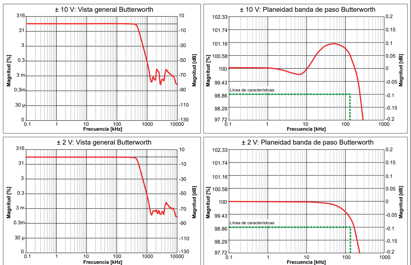
Figura 15: Ejemplos representativos de filtros Butterworth
