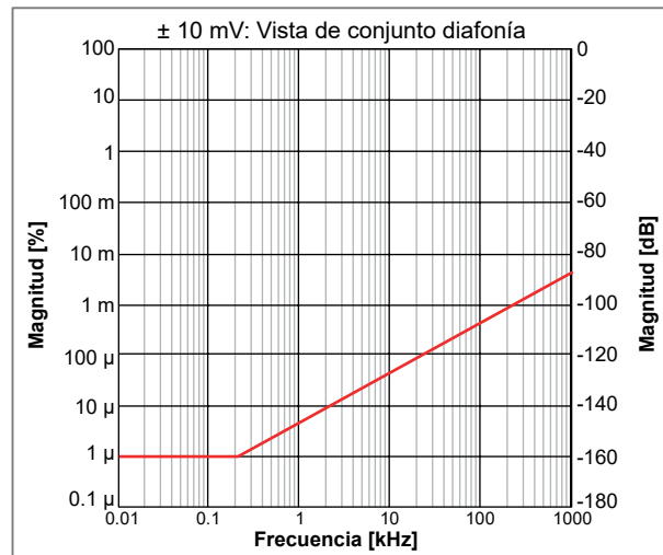
Figura 28: Representación de la diafonía canal a canal
