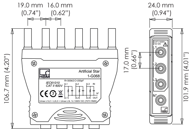
그림 40: 인공 스타 어댑터
