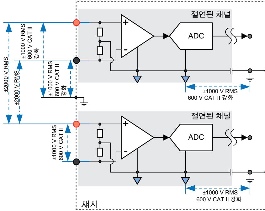
그림 8: 절연 1kV 데이터 수집 카드 개요
