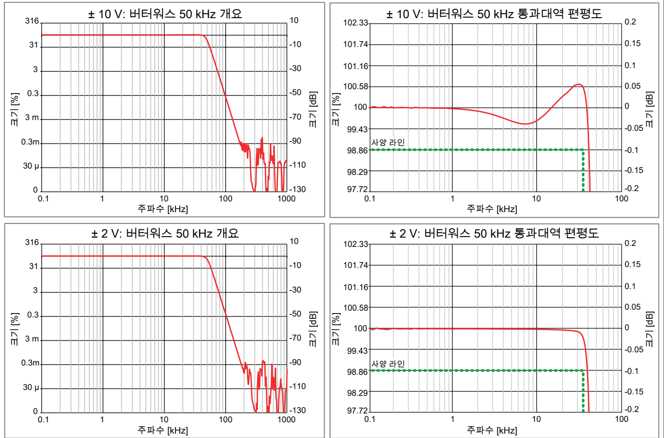
그림 23: 대표적 버터워스 IIR 예시
