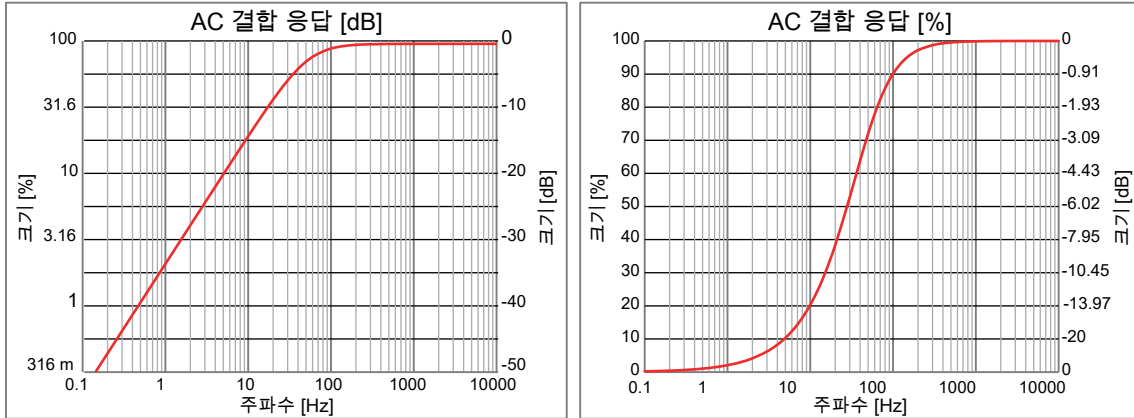
그림 4: 대표적인 AC 결합 응답
