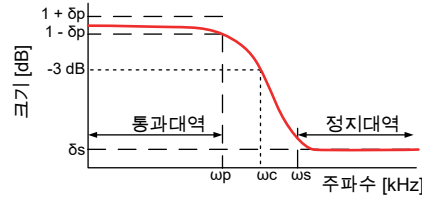
그림 14: 버터워스 필터
