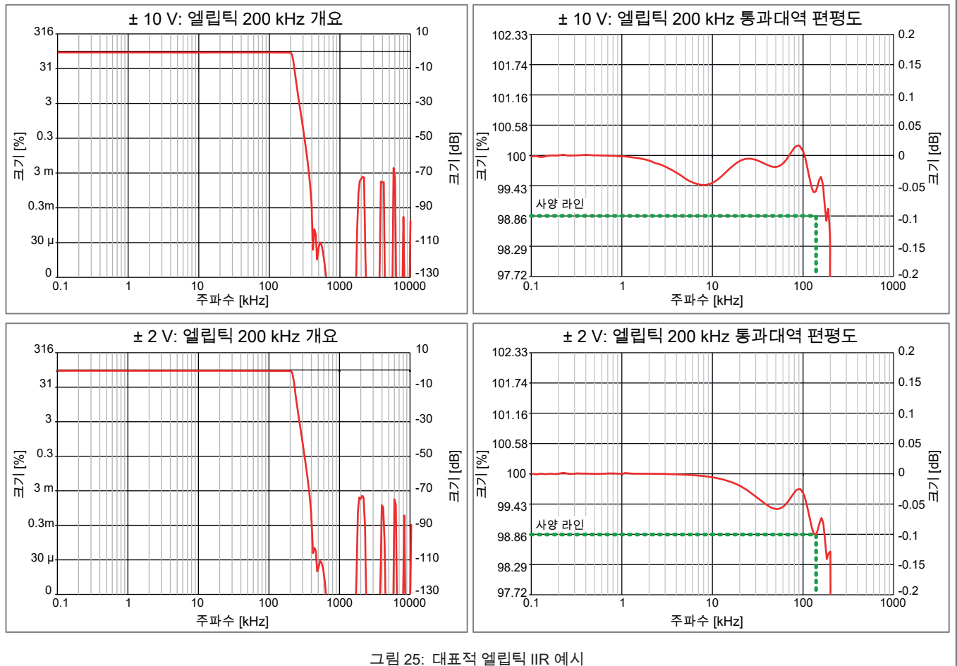
그림 25: 대표적 엘리틱 IIR 예시
