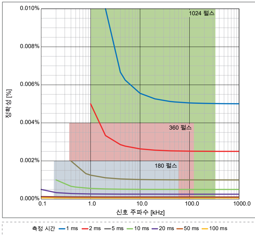
그림 35: RPM 센서 작동 범위 대 부정확 및 측정 시간
