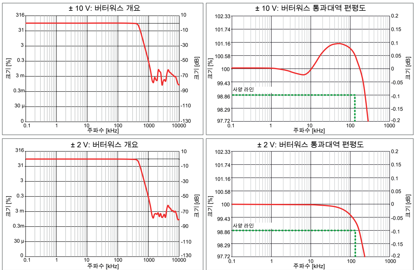
그림 15: 대표적 버터워스 예시
