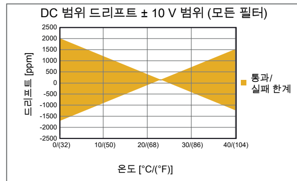
그림 7: 사용된 모든 필터 전압 사양
