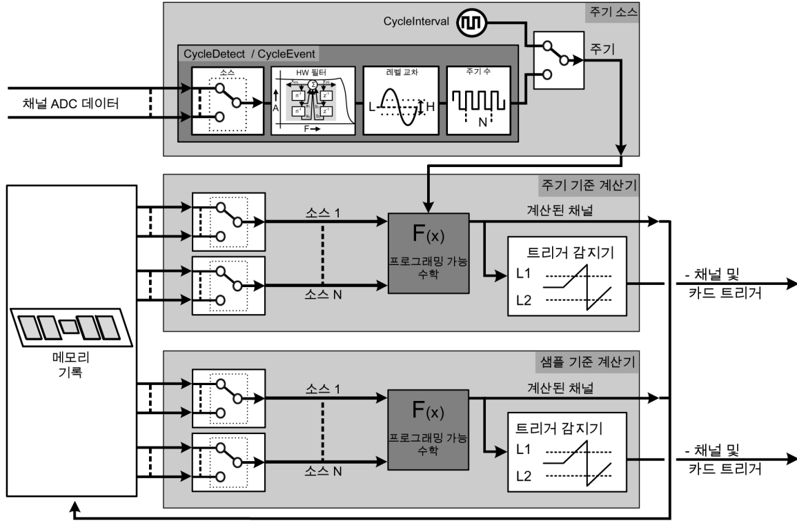
그림 38: 실시간 포물라 데이터베이스(formula database) (RT-FDB) 계산기
