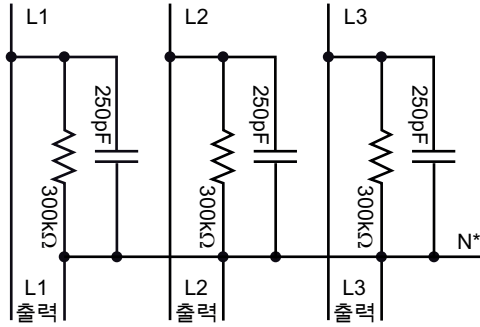
그림 39: 전기 회로도
