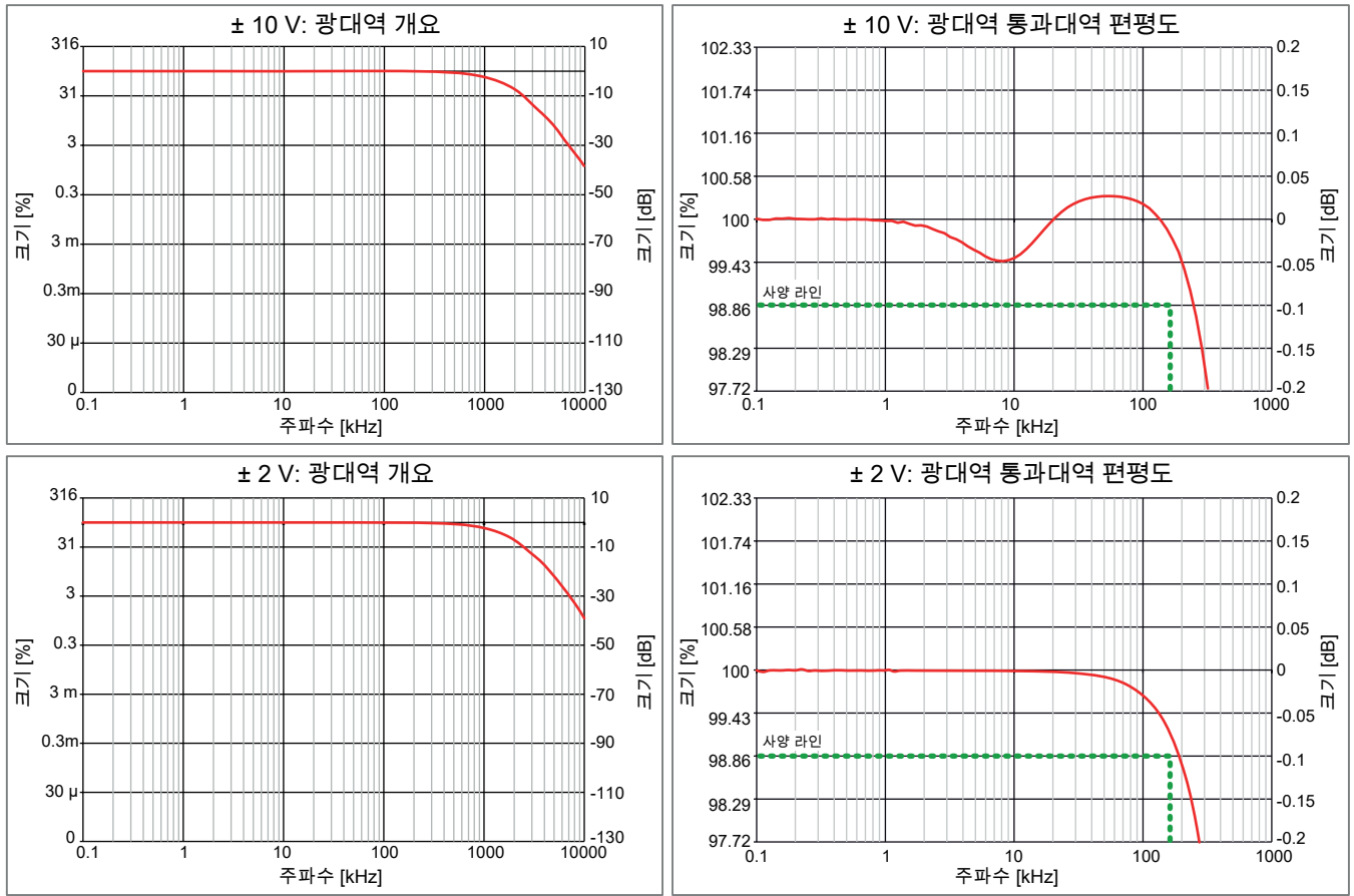
그림 11: 대표적 광대역 예시
