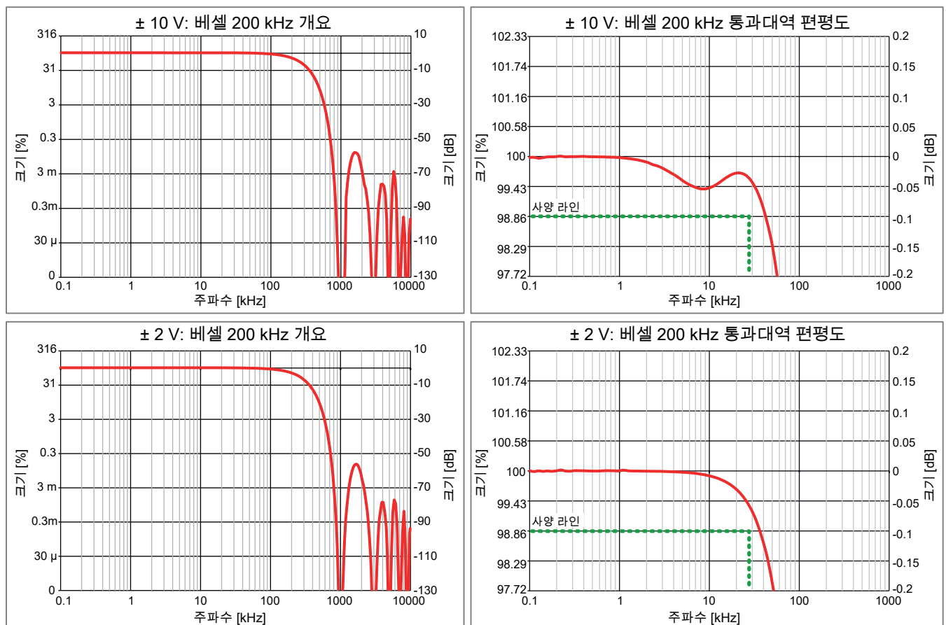
그림 17: 대표적 베셀 IIR 예시
