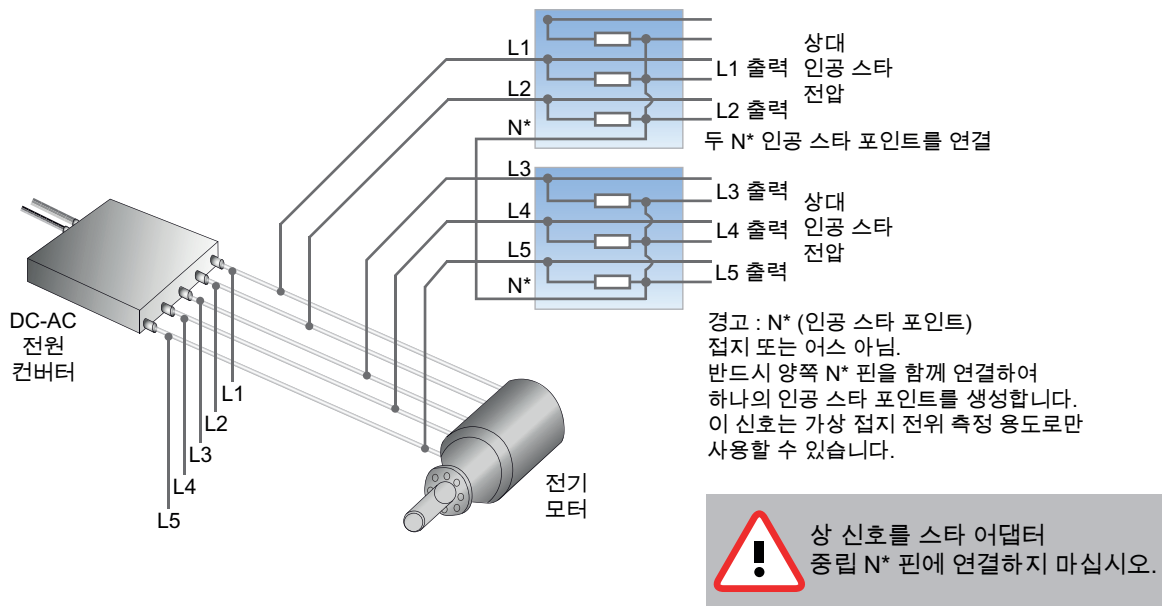
그림 42: 이중 스타 어댑터의 5 상 이상 대표적 사용
