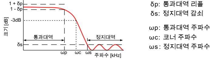
그림 18: 디지털 베셀 IIR 필터
