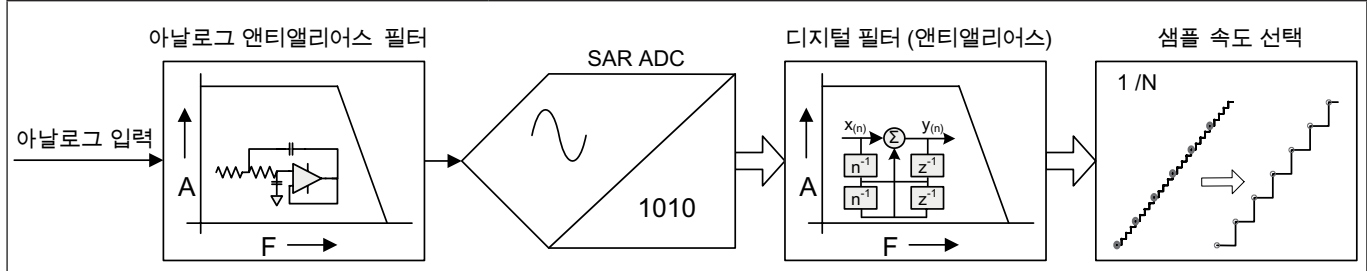
그림 10: 결합된 아날로그 및 디지털 앤티앨리어스 필터 블록도
