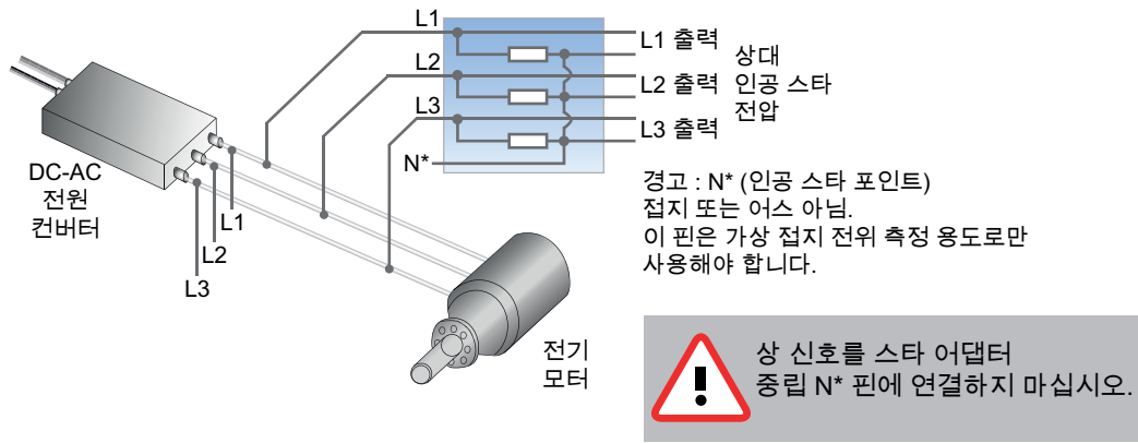
그림 41: 인공 스타 어댑터의 3 상 대표적 사용
