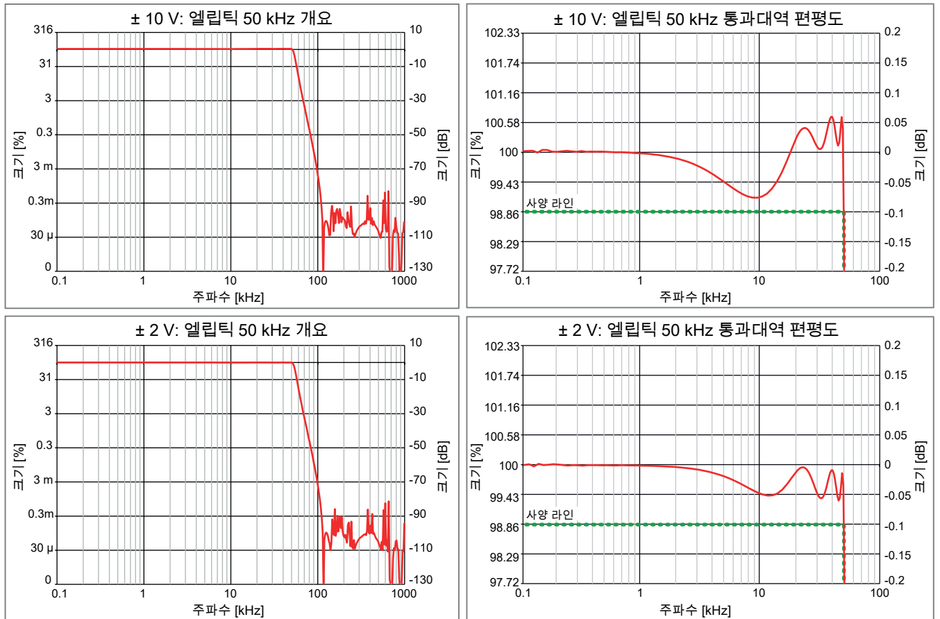
그림 27: 대표적 엘리틱 IIR 예시
