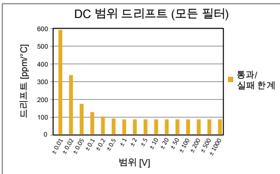
그림 7: 사용된 모든 필터 전압 사양
