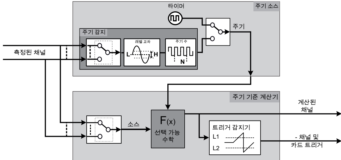
그림 37: 실시간 주기 기준 계산기
