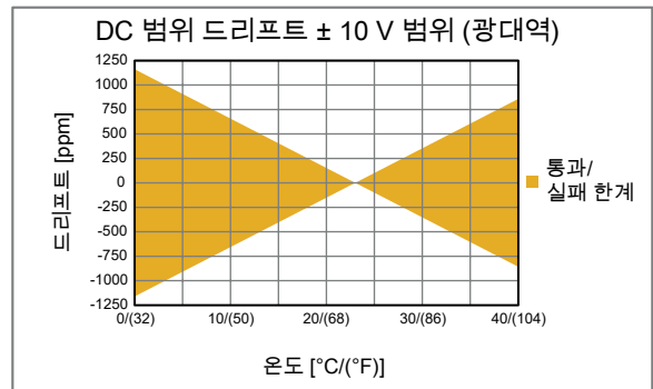
그림 6: 광대역 전압 사양
