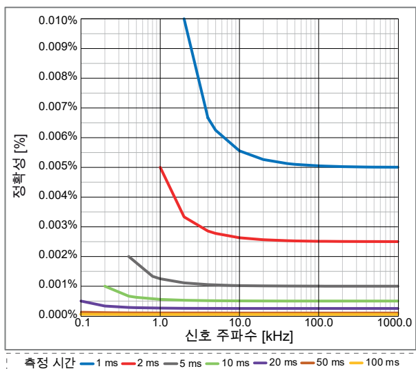
그림 33: 최대 타이머 부정확
