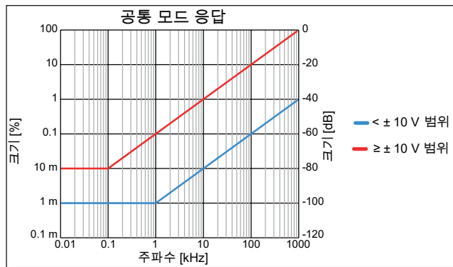
그림 5: 대표적 공통 모드 응답
