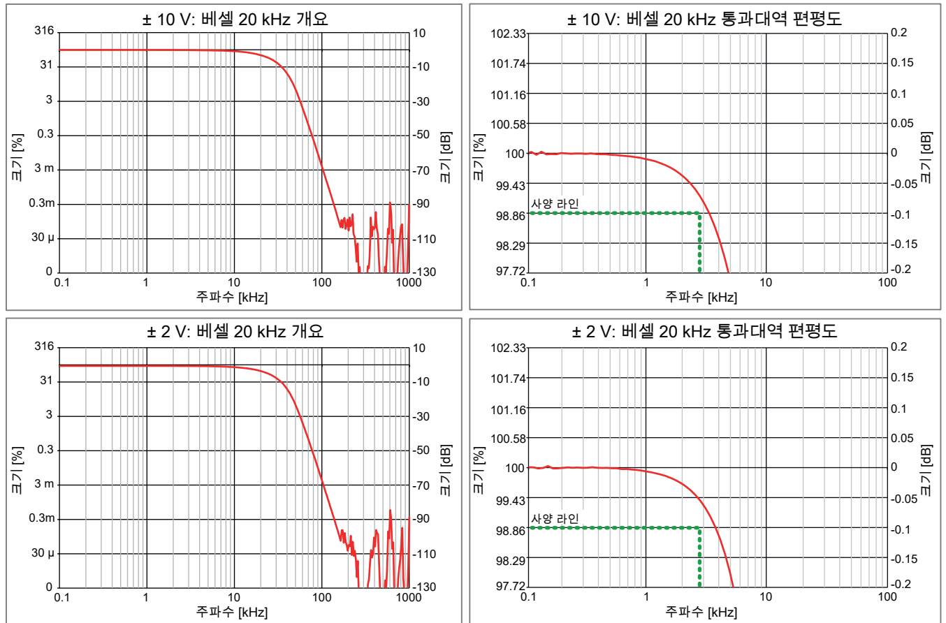
그림 19: 대표적 베셀 IIR 예시
