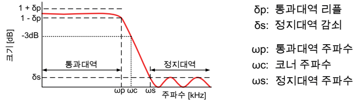
그림 22: 디지털 버터워스 IIR 필터
