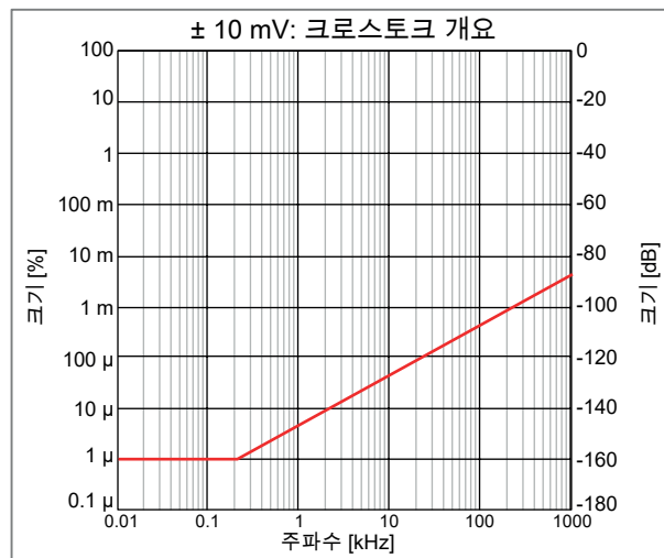
그림 28: 대표적 채널 대 채널 크로스토크
