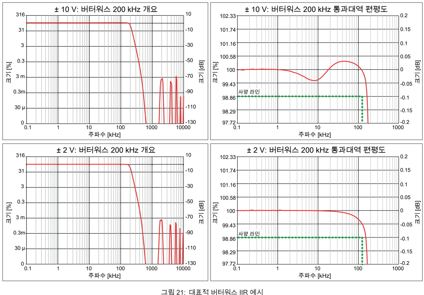
그림 21: 대표적 버터워스 IIR 예시
