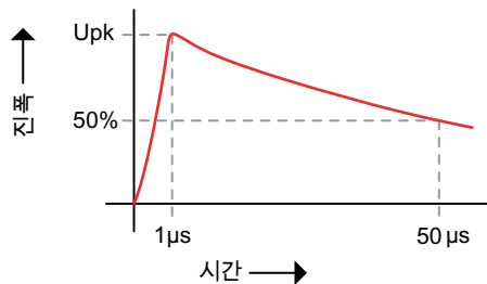
그림 9: 1.2/50 μs 임펄스 예
