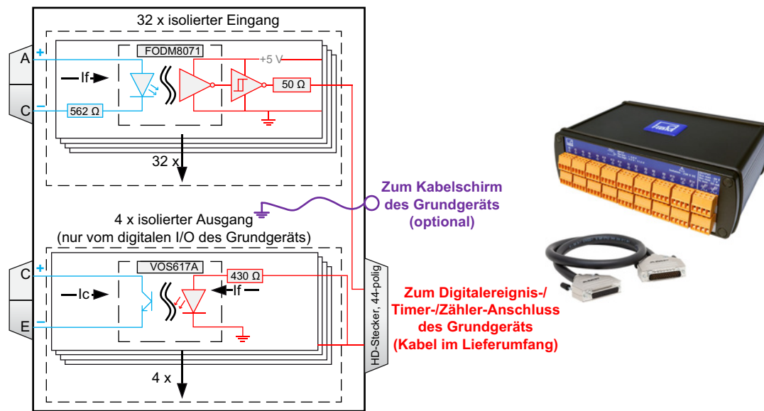
Abbildung 1.33: Blockschaltbild und Abbildung
