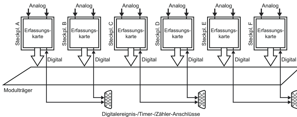
Abbildung 1.13: Blockschaltbild Digitalereignis/Timer/Zähler
