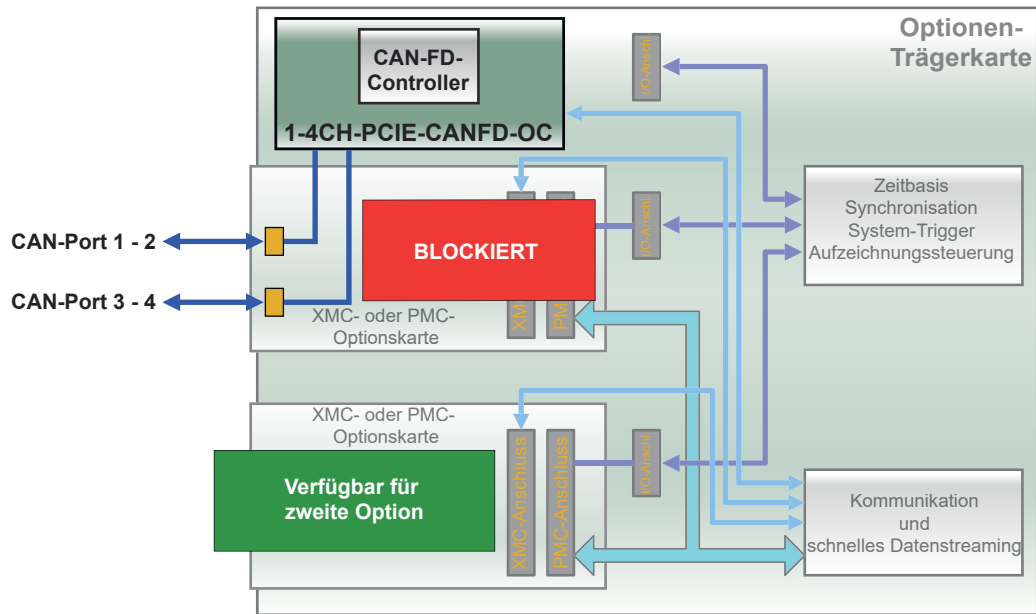
Abbildung 1.25: Blockschaltbild von 1-4C-PCIE-CAN FD-OC (erfordert G081)
