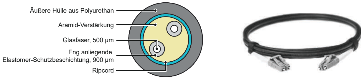
Abbildung 1.31: Schematische Darstellung und Abbildung
