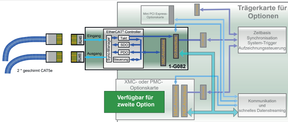
Abbildung 1.24: Blockschaltbild der EtherCAT®-Karte
