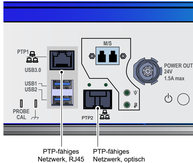
Abbildung 1.8: Schnittstelle zu 1-Gigabit-Netzwerk, elektrisch und optisch
