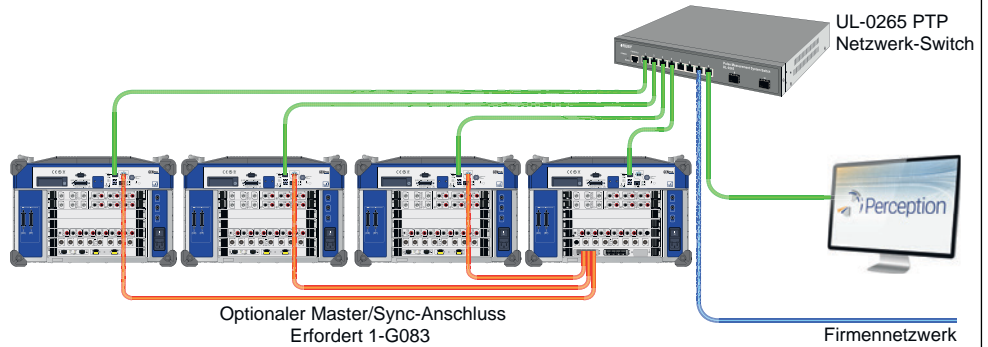
Abbildung 1.4: Mehrere Grundgeräte
