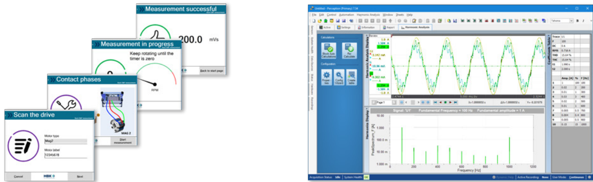
Abbildung 1.43: Beispiele für Perception CSI: BackEMF (links) Analyse von Oberschwingungen (rechts)
