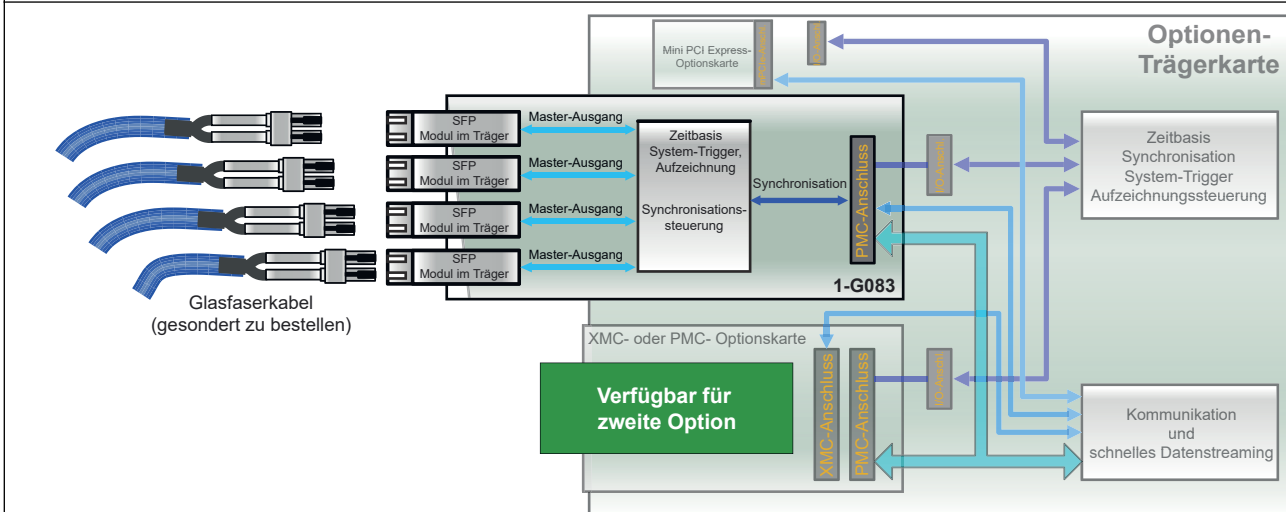
Abbildung 1.23: Blockschnittbild der Master-Ausgangskarte (erfordert G081)
