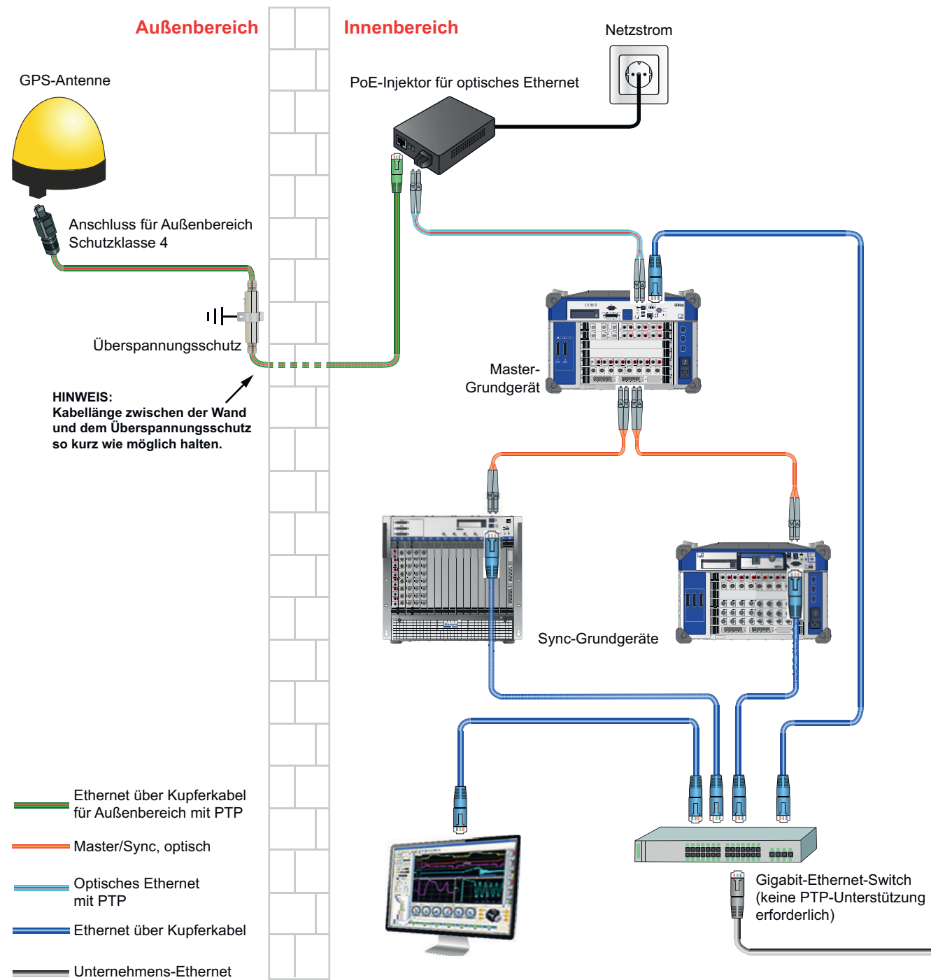
Abbildung 1.36: GPS-Konfiguration für kabelgebundenes Grundgerät mit angeschlossenen Sync-Grundgeräten in einem Master/Sync-System
