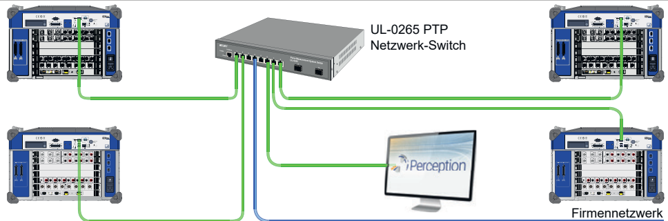
Abbildung 1.5: Mehrere Grundgeräte (verteilt)
