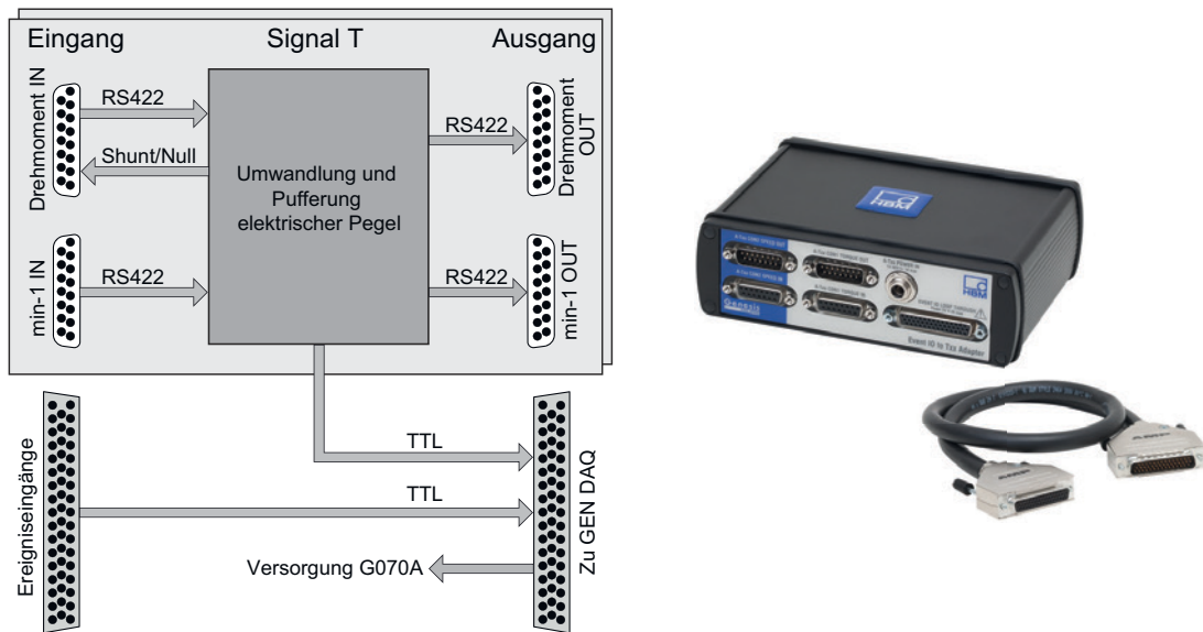
Abbildung 1.32: Blockschaltbild und Abbildung
