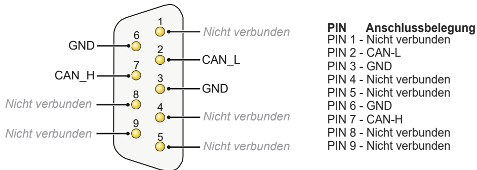
Abbildung 1.28: D-Sub-Anschlussbelegung
