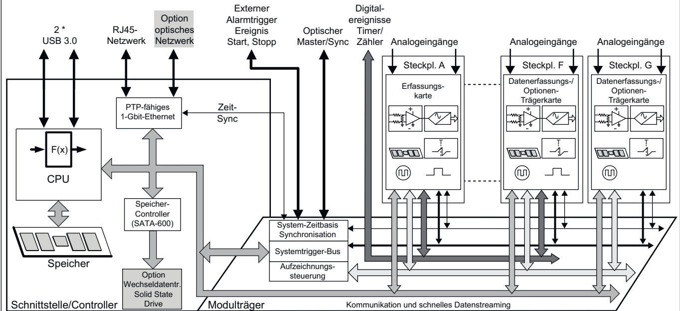
Abbildung 1.6: Blockschaltbild
