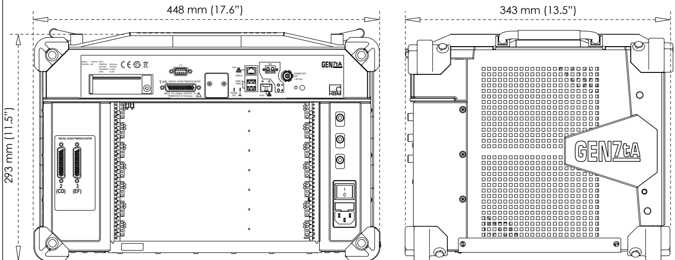
Abbildung 1.18: Abmessungen des GEN7tA
