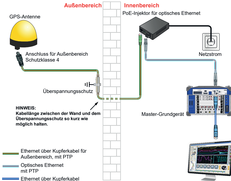
Abbildung 1.35: Beispielkonfiguration der GPS-Zeitsynchronisation
