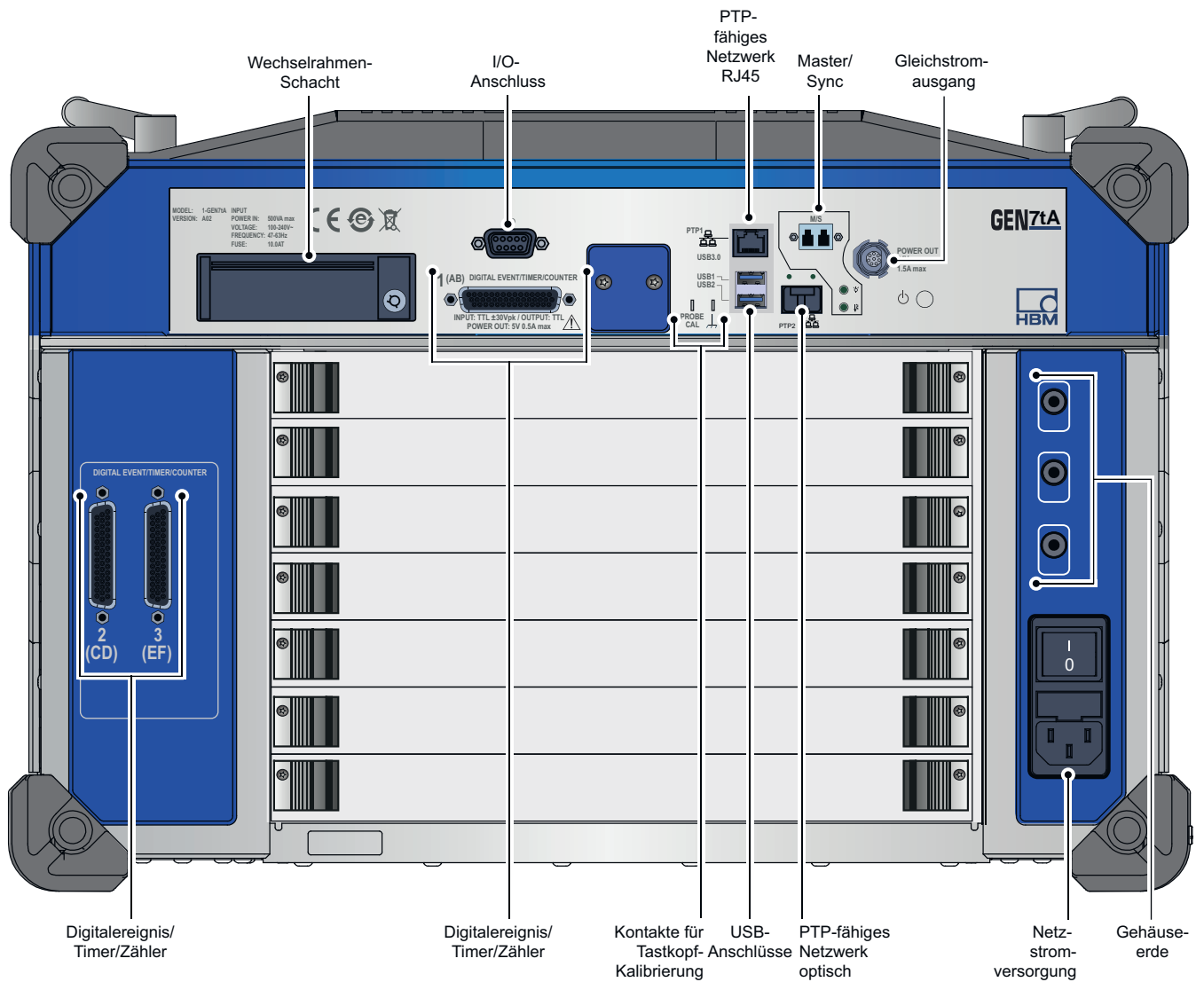
Abbildung 1.7: Anschlussübersicht
