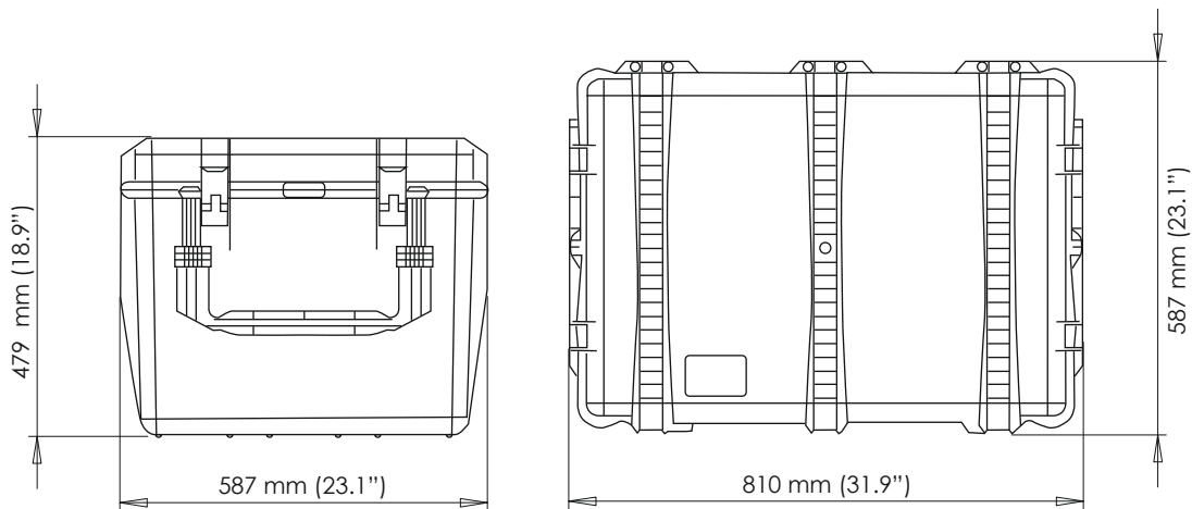
Abbildung 1.38: Wiederverwendbarer Hartschalen-Transportkoffer mit Rädern und Transportgriff
