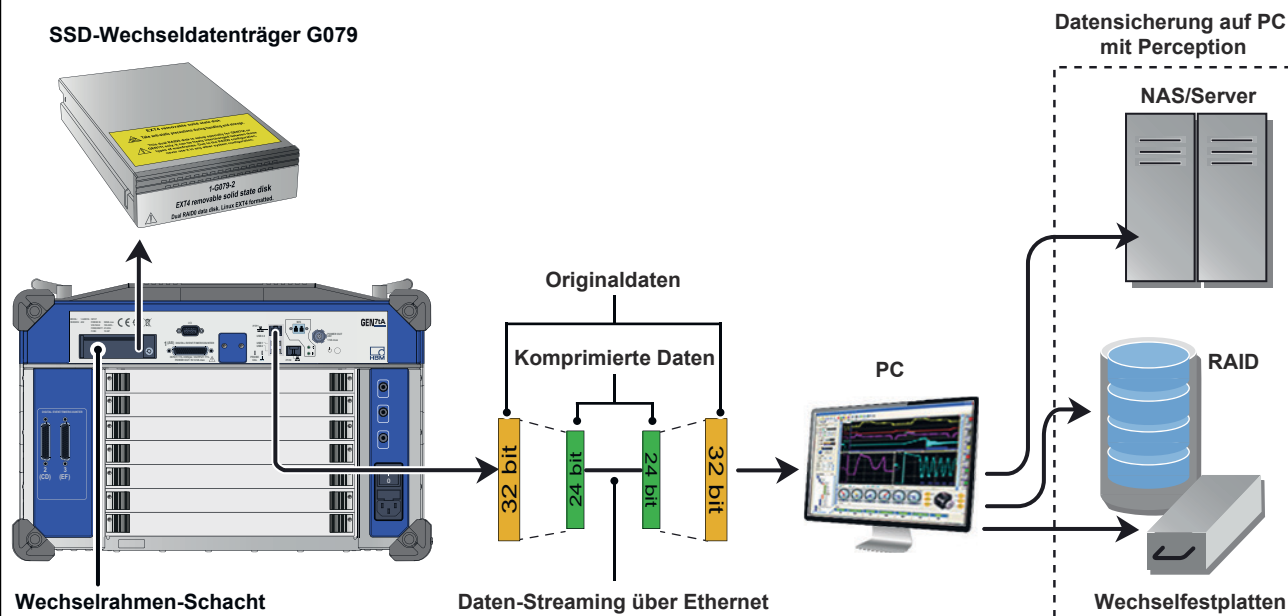
Abbildung 1.9: Kontinuierliches Streaming – Übersicht
