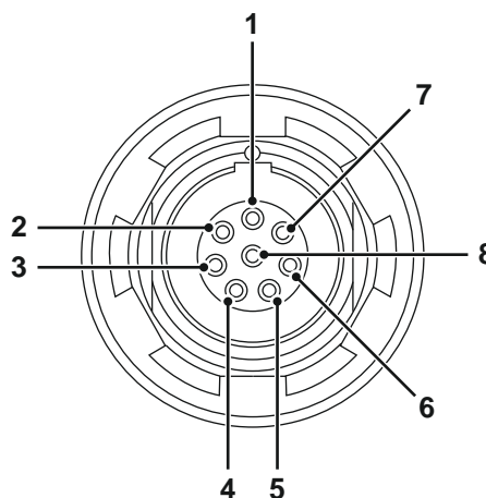
Abbildung 1.16: Anschluss des Gleichstromausgangs
