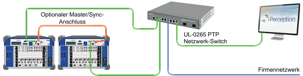
Abbildung 1.3: Zwei Grundgeräte
