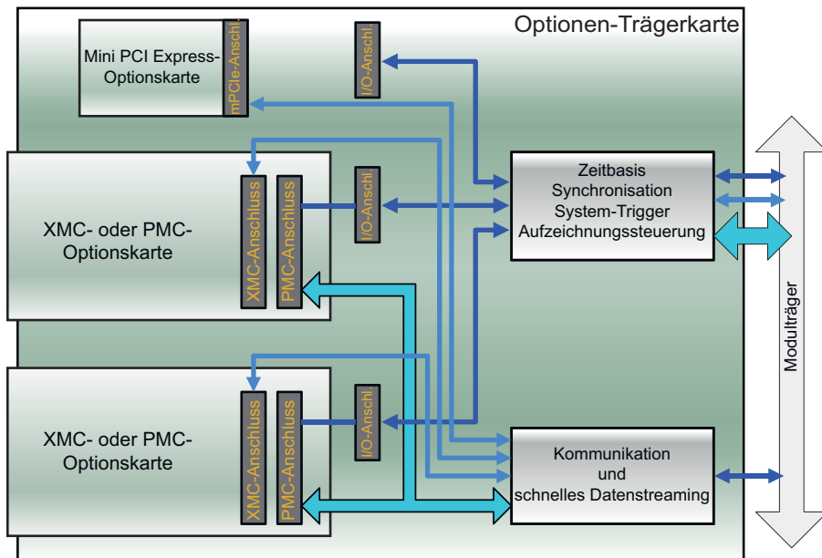
Abbildung 1.21: Blockschaltbild der Optionen-Trägerkarte
