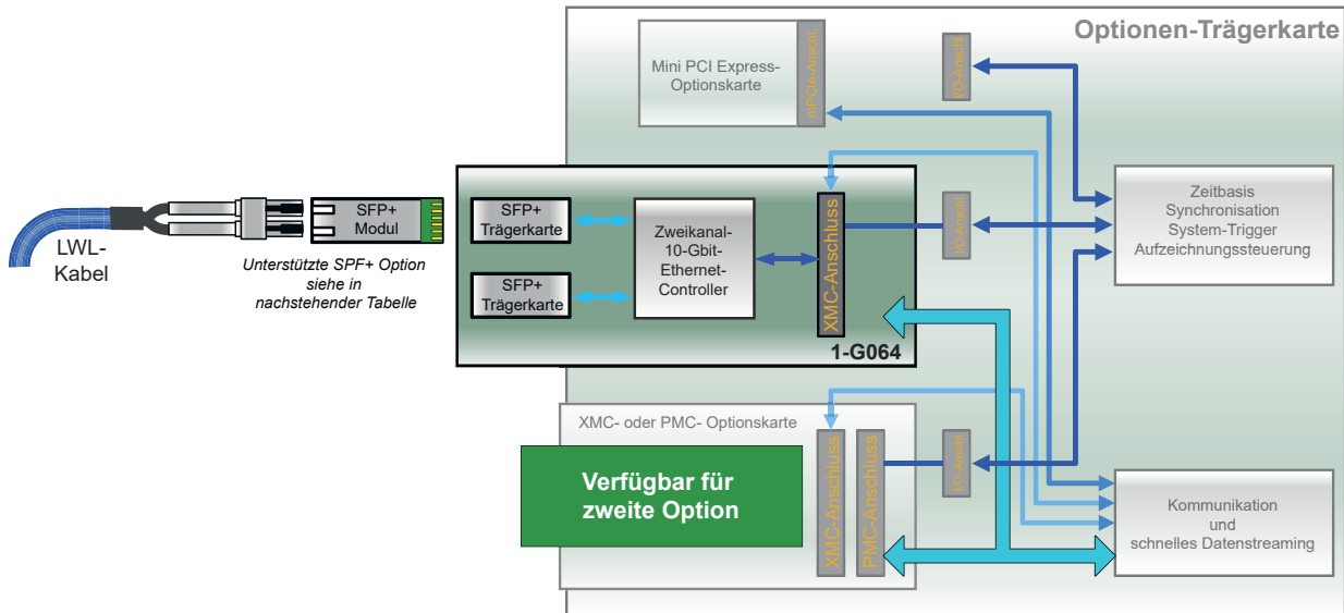
Abbildung 1.22: Blockschaltbild der Karte für 10-Gigabit-Ethernet, optisch (erfordert G081)
