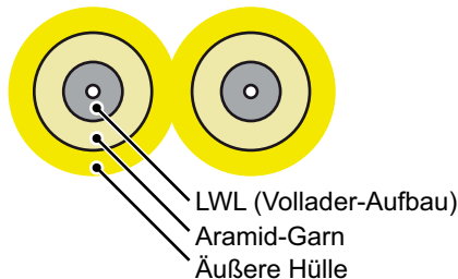
Abbildung 1.30: Schematische Darstellung und Abbildung
