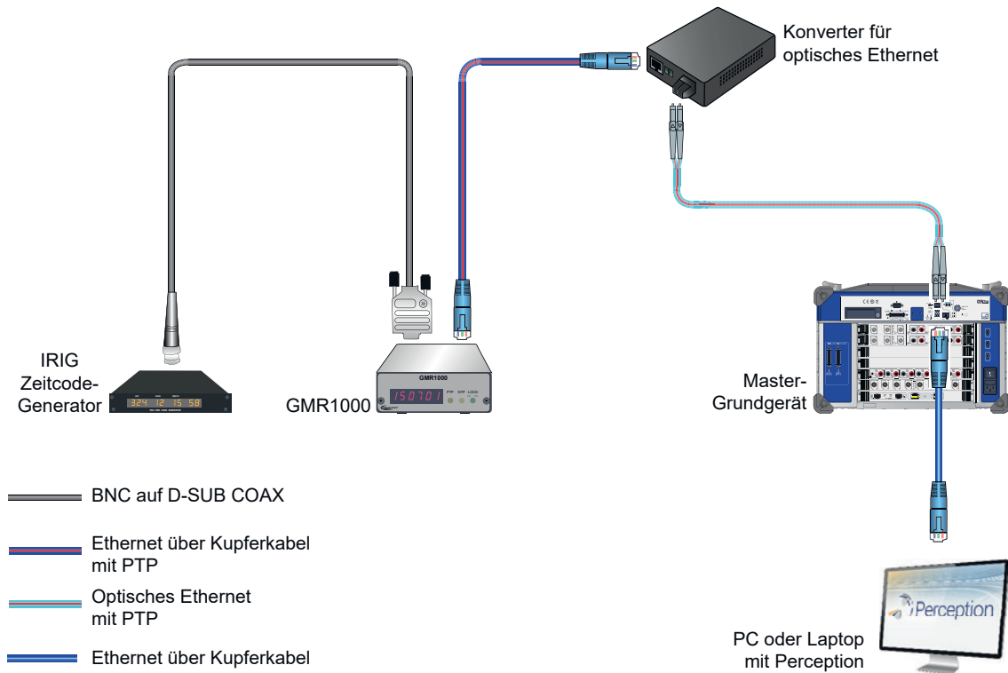
Abbildung 1.34: Beispielkonfiguration der IRIG-Zeitsynchronisation
