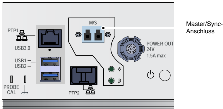
Abbildung 1.10: Master/Sync-Anschluss
