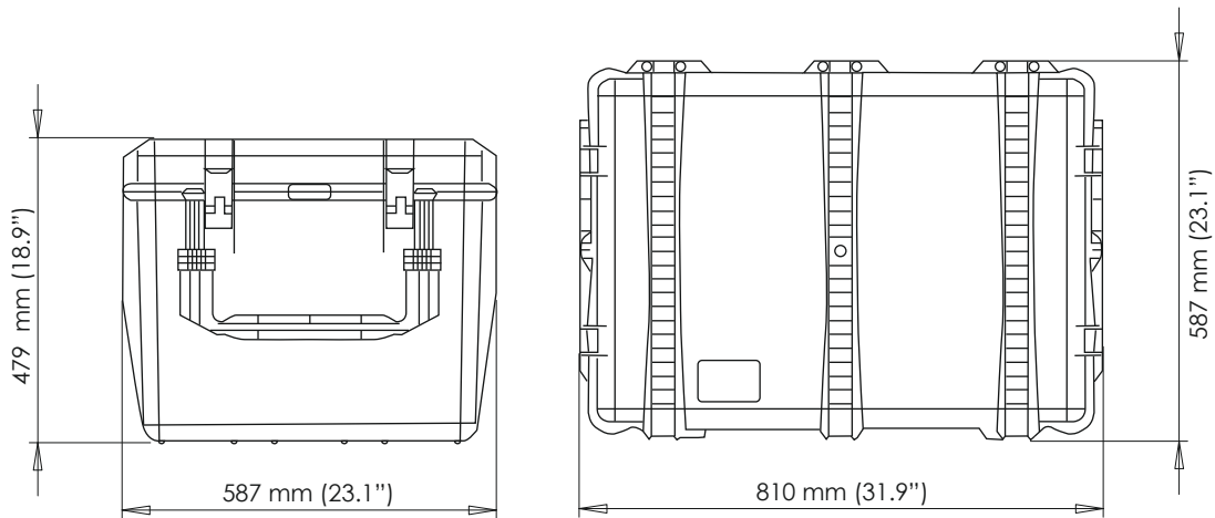
그림 1.38: 재활용 가능 하드커버 배송 케이스(휠 및 운송 핸들 포함)
