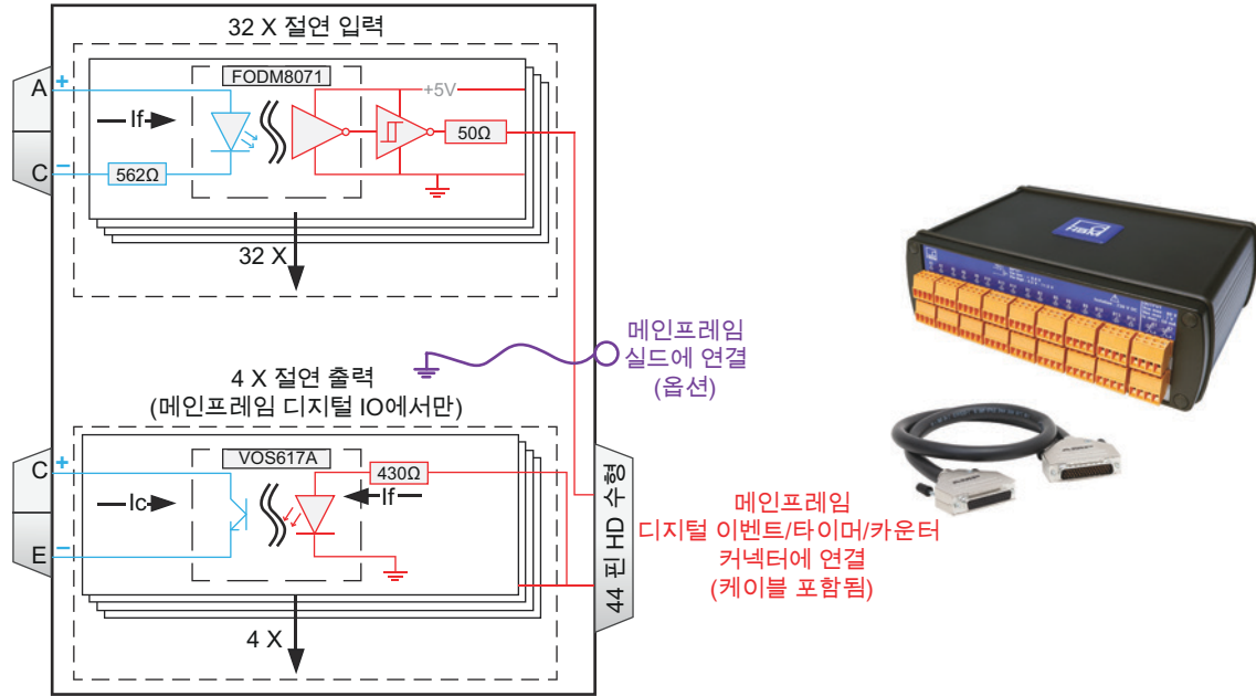
그림 1.33: 블록도 및 이미지
