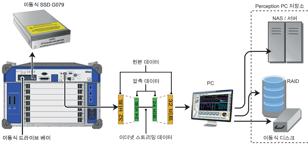
그림 1.9: 연속 스트리밍 개요
