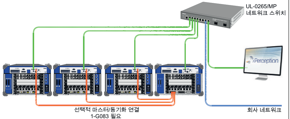
그림 1.4: 멀티 메인프레임
