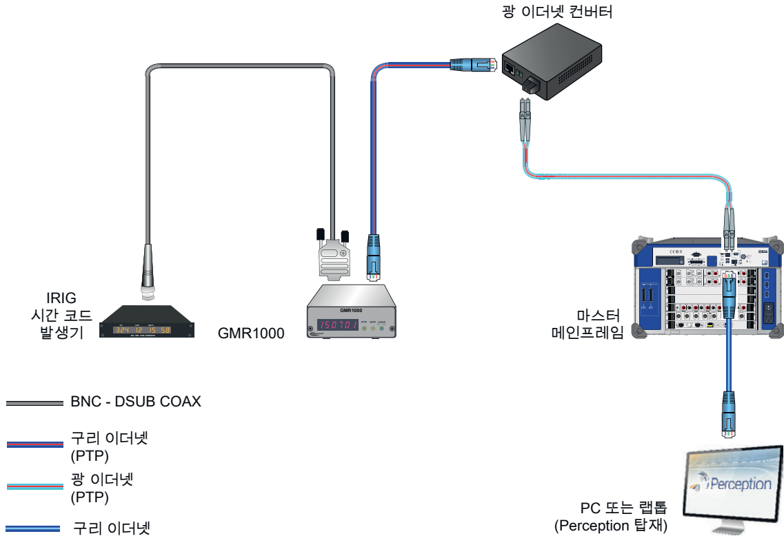
그림 1.34: 예제 설정 IRIG 시간 동기화
