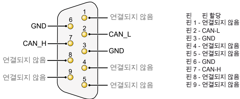
그림 1.28: 핀 할당 D-Sub
