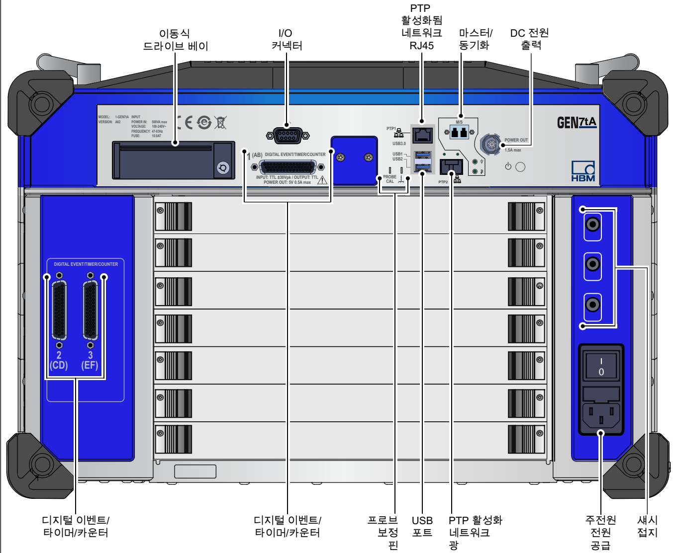
그림 1.7: 연결 개요
