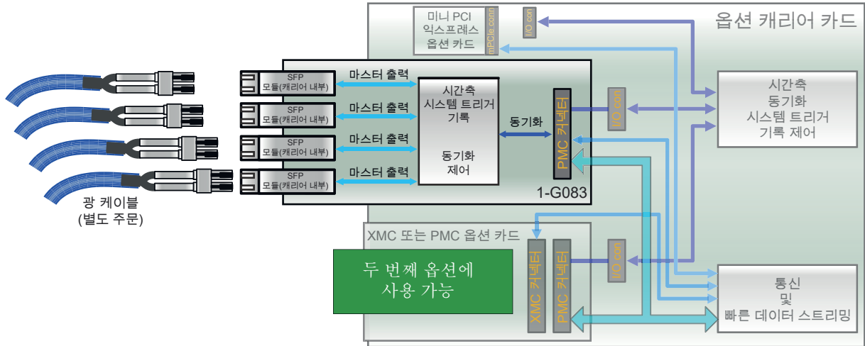
그림 1.23: 블록도 마스터 출력 카드 (G081 필요)
