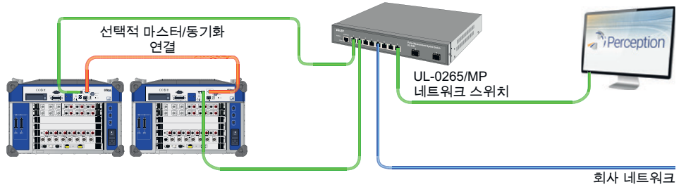
그림 1.3: 듀얼 메인프레임
