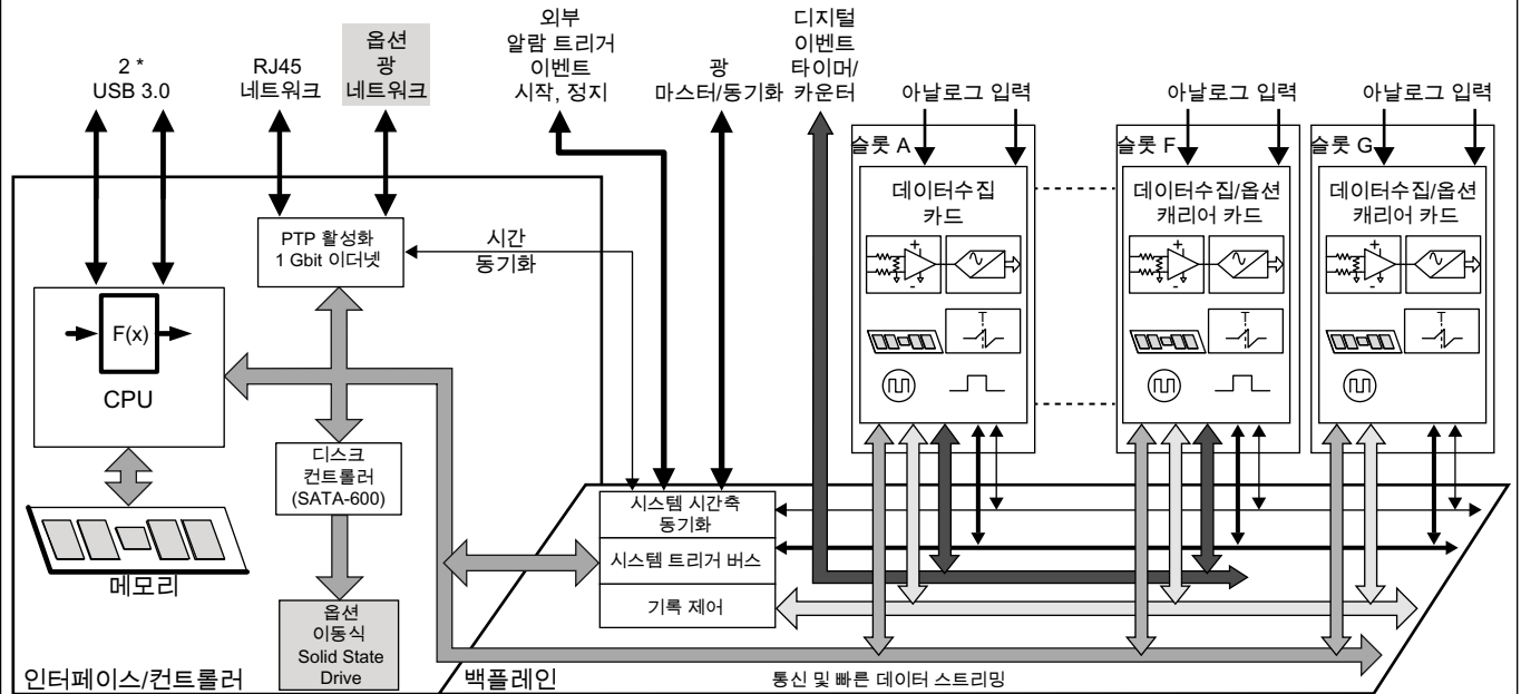
그림 1.6: 블록도
