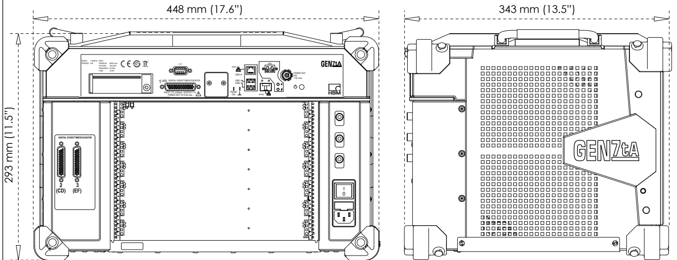
그림 1.18: GEN7tA 치수
