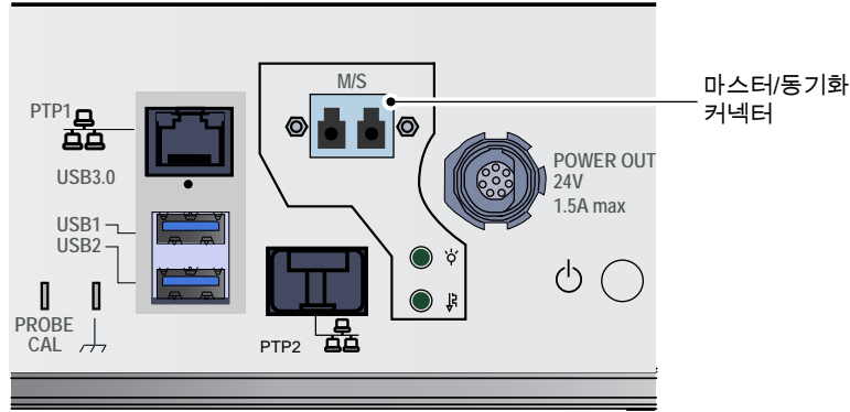
그림 1.10: 마스터/동기화 커넥터
