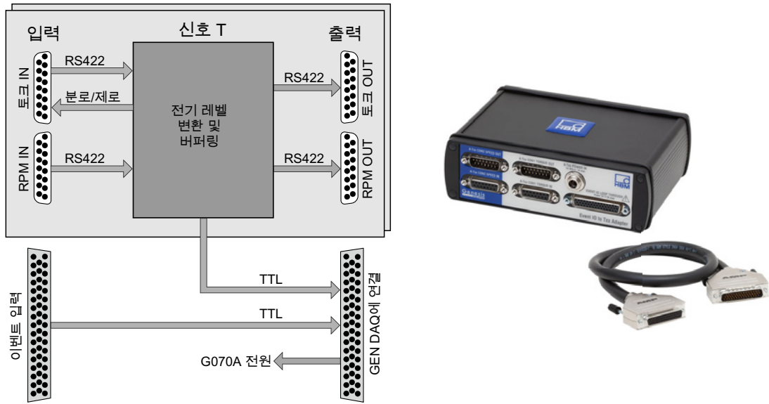
그림 1.32: 블록도 및 이미지
