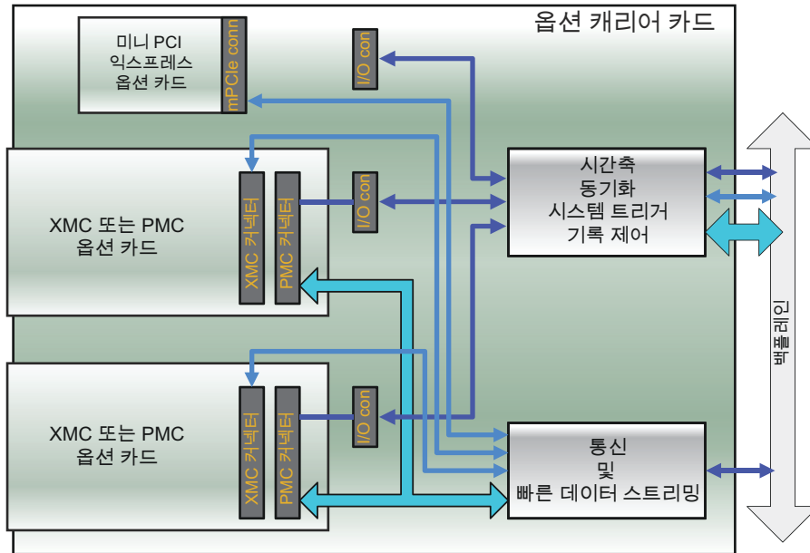
그림 1.21: 블록도 옵션 캐리어 카드
