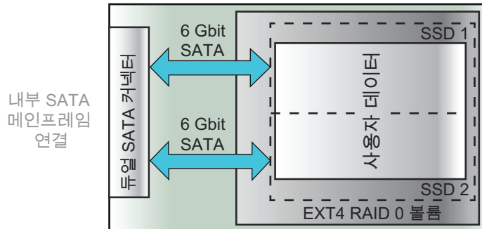
그림 1.20: 블록도 드라이브
