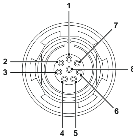
그림 1.16: 커넥터 전원 출력
