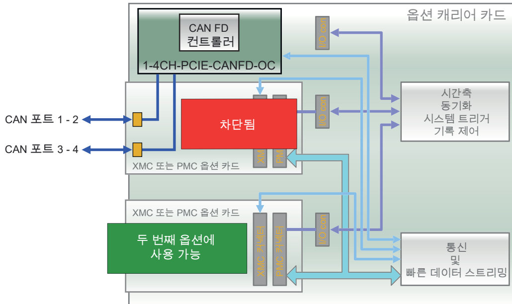
그림 1.25: 블록도 1-4C-PCIE-CAN FD-OC (G081 필요)
