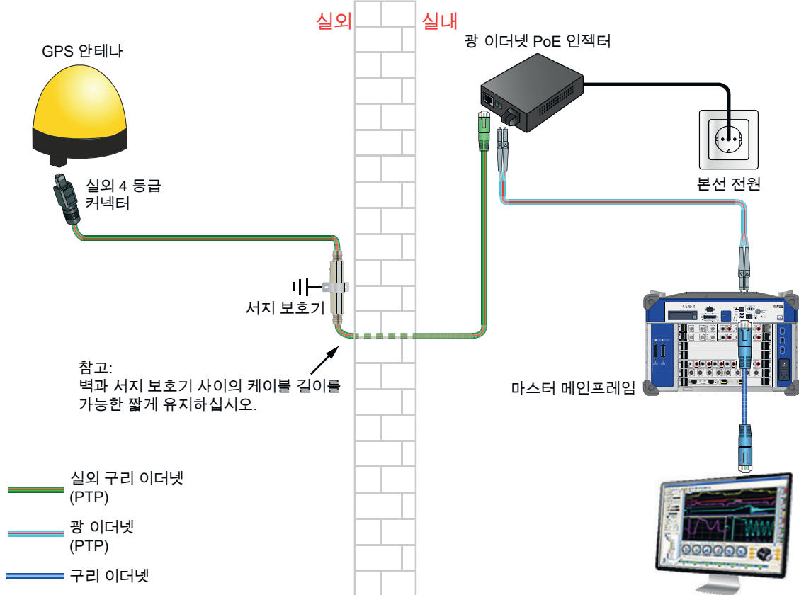
그림 1.35: 예제 설정 GPS 시간 동기화
