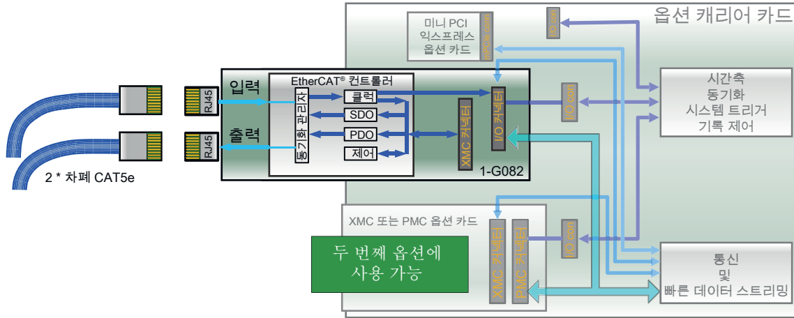
그림 1.24: 블록도 EtherCAT® 카드
