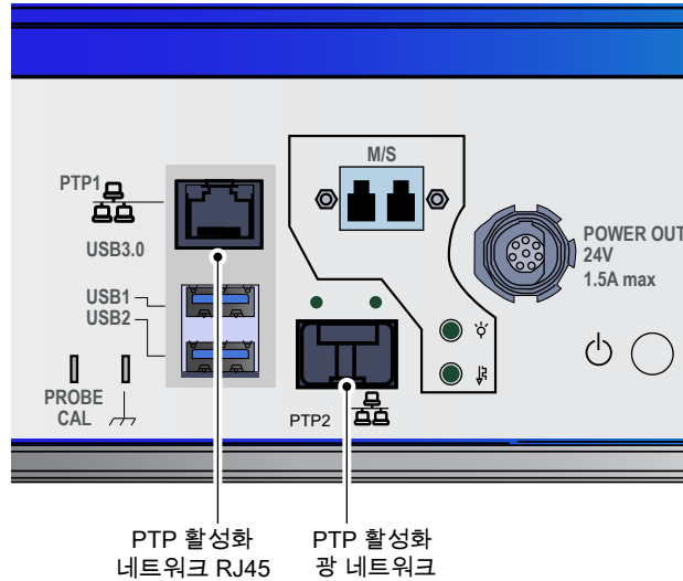
그림 1.8: 전기 및 광 1 Gbit 네트워크 인터페이스
