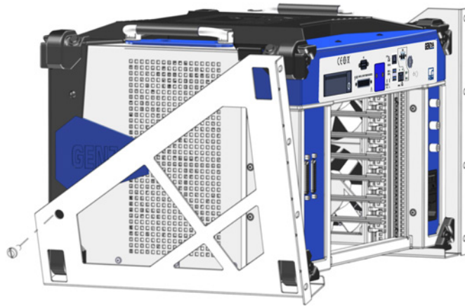
그림 1.37: GEN7tA 랙 장착 키트
