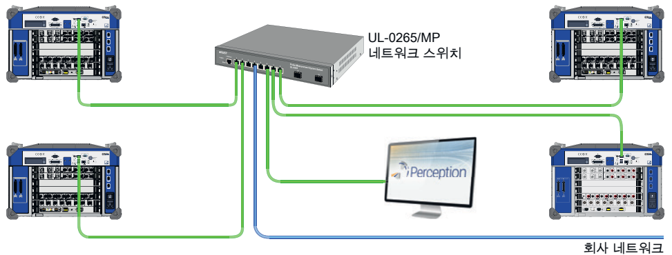
그림 1.5: 멀티 메인프레임 (분산)
