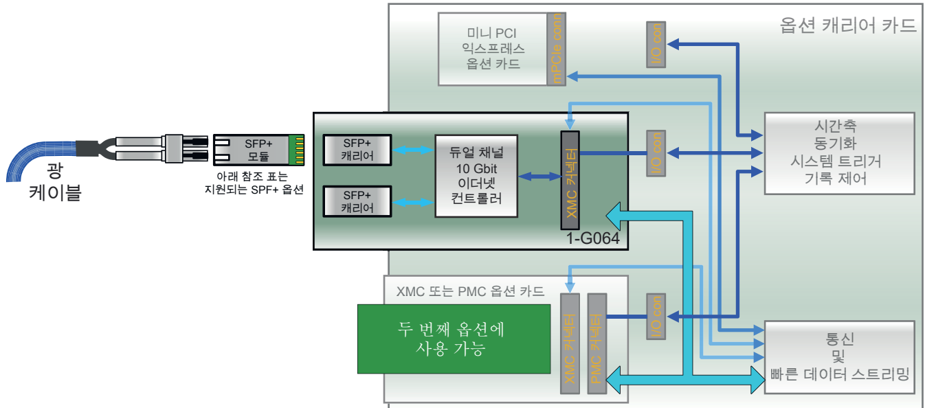
그림 1.22: 블록도 10Gbit 이더넷 카드, 광 (G081 필요)
