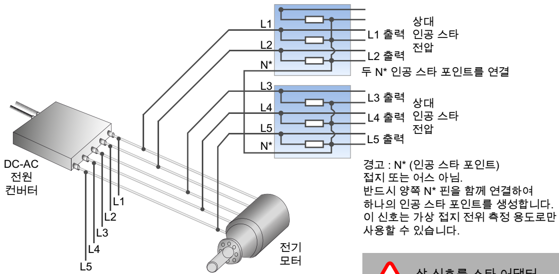
그림 1.30: 인공 스타 어댑터의 3 상 대표적 사용
