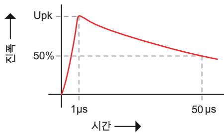
그림 1.7: 1.2/50 μs 임펄스 예
