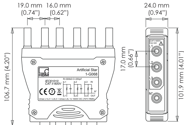
그림 1.29: 인공 스타 어댑터
