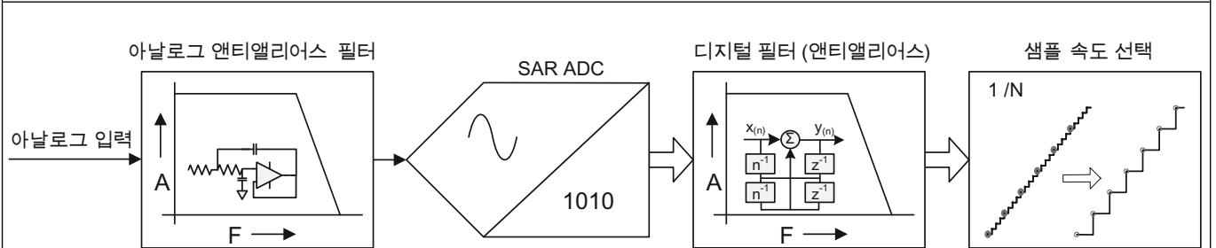
그림 1.8: 결합된 아날로그 및 디지털 엔티앨리어스 필터 블록도
