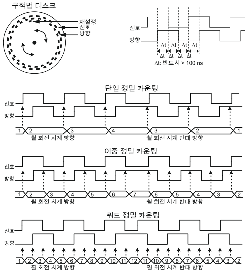
그림 1.18: 양방향 구적법(quadrature) 카운트 모드
