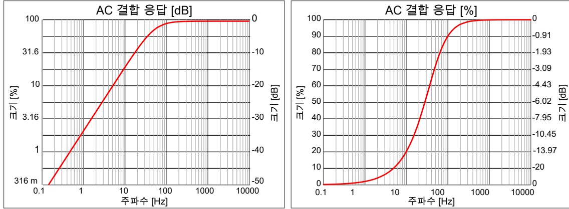
그림 1.4: 대표적인 AC 결합 응답
