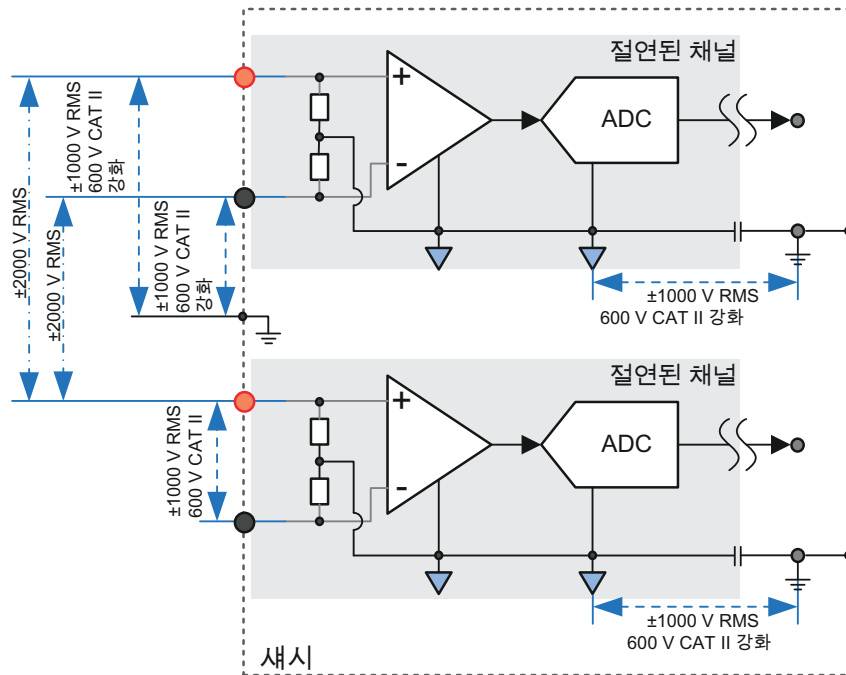
그림 1.6: 절연 1kV 데이터 수집 카드 개요
