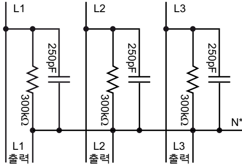
그림 1.28: 전기 회로도
