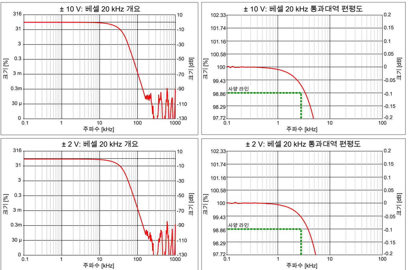
그림 1.10: 대표적 베셀 IIR 예시
