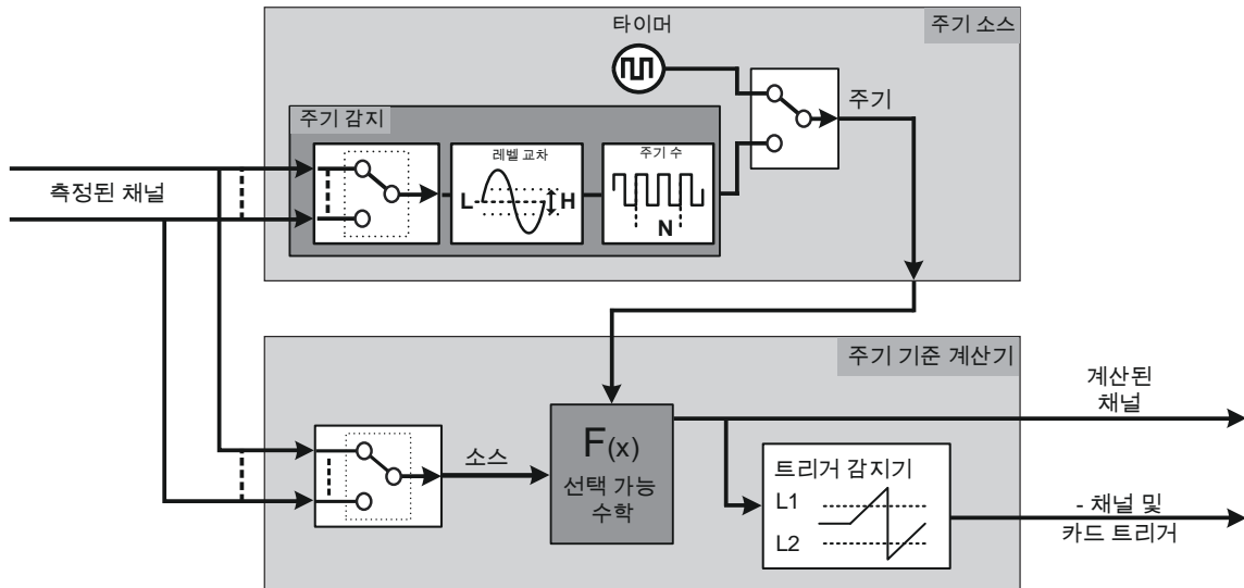
그림 1.24: 실시간 주기 기준 계산기
