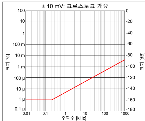
그림 1.15: 대표적 채널 대 채널 크로스토크
