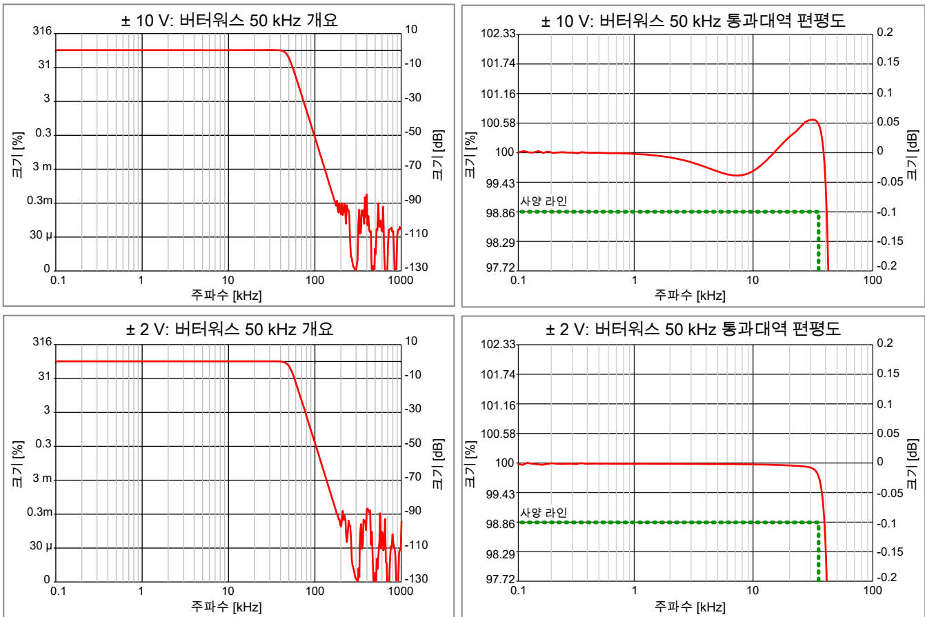
그림 1.12: 대표적 버터워스 IIR 예시
