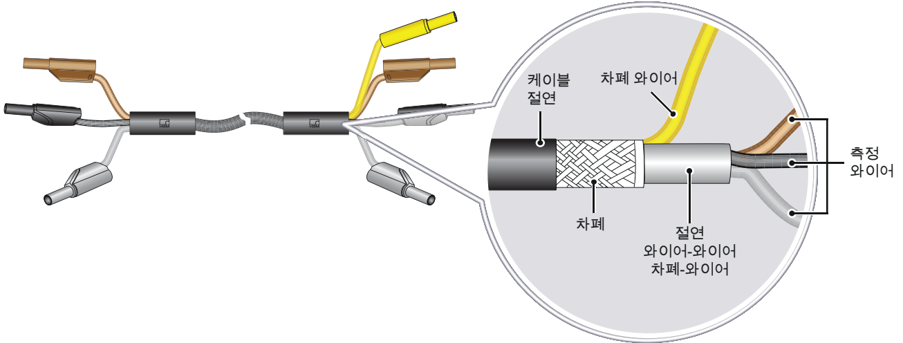
그림 1.26: 세 와이어 차폐 케이블 설정
