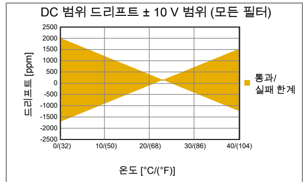
그림 1.5: 사용된 모든 필터 전압 사양
