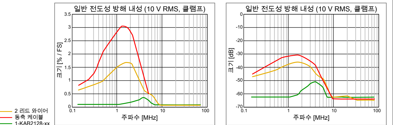
그림 1.27: 일반 전도 내성, ± 10 V 범위를 사용하여 테스트됨
