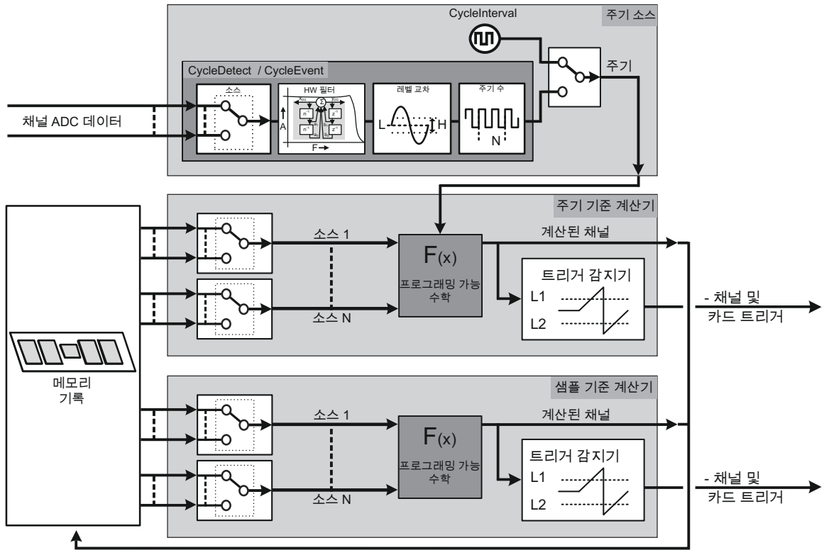
그림 1.25: 실시간 포물라 데이터베이스(formula database) (RT-FDB) 계산기
