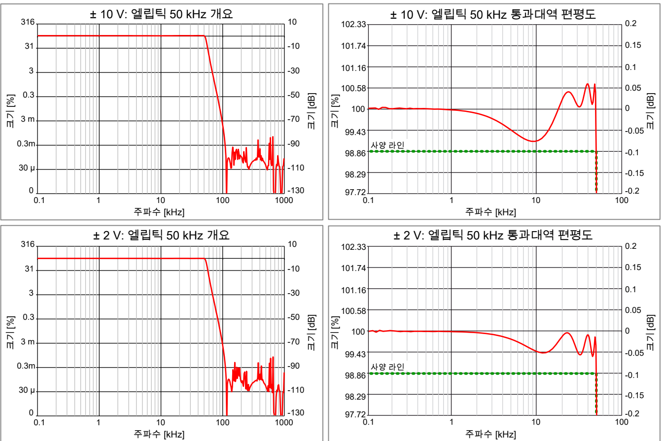
그림 1.14: 대표적 엘리틱 IIR 예시
