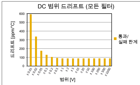
그림 1.5: 사용된 모든 필터 전압 사양
