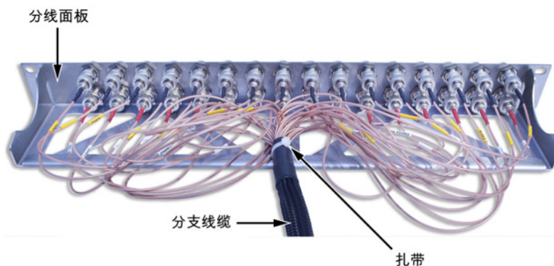
图 25: 分线线缆连接到分线面板
