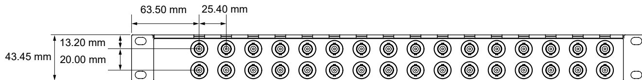
图 24: 分线面板尺寸
