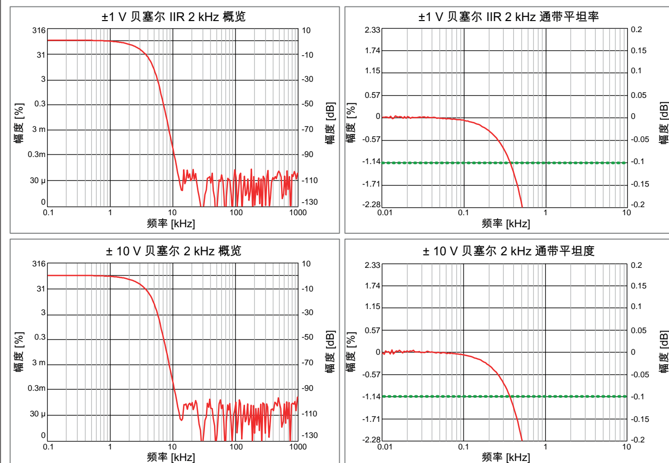
图 10: 典型贝塞尔 IIR 的示例
