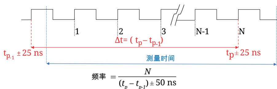
图 16: 频率测量
