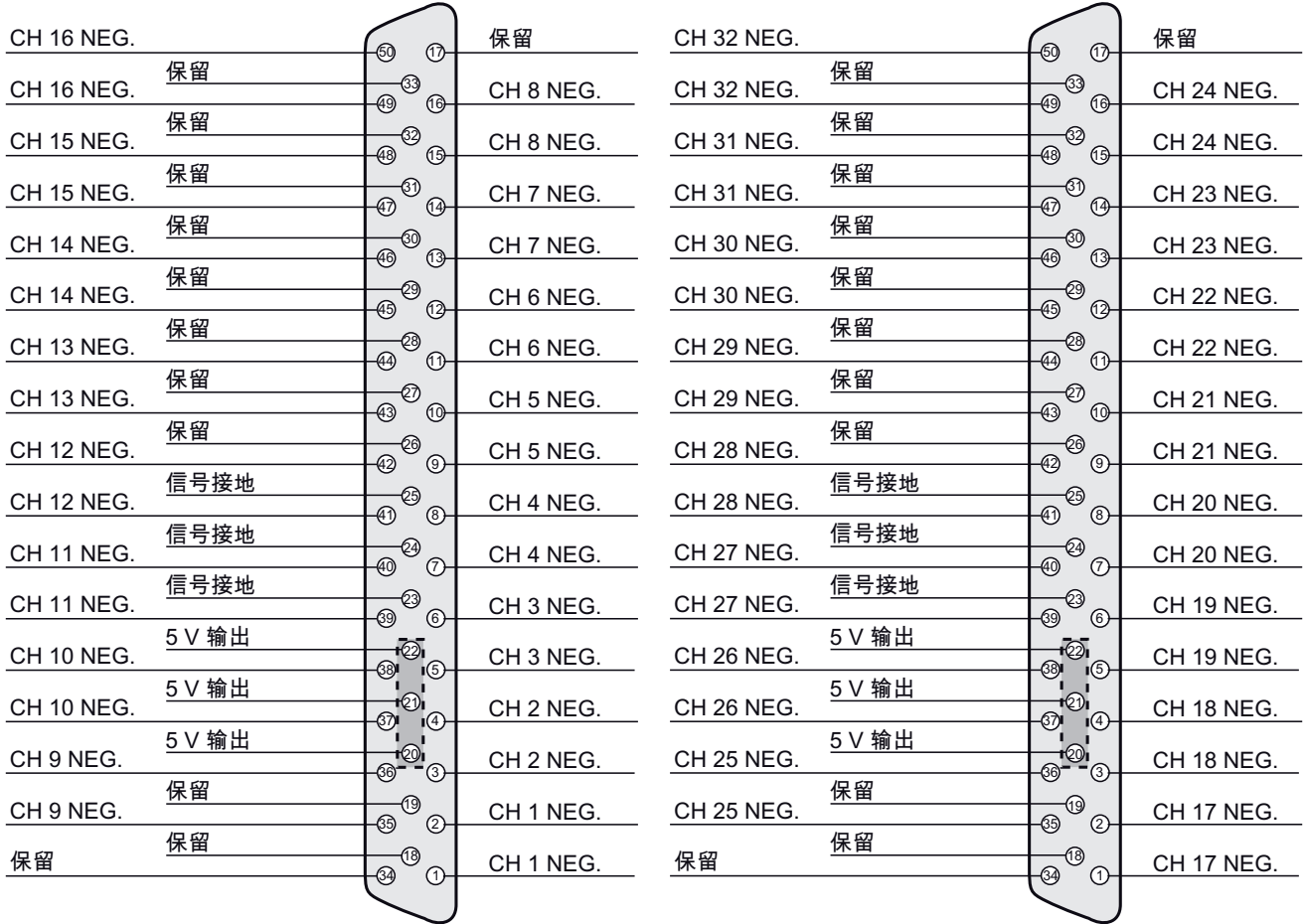
图 21: 输入接头引脚示意图 (正视图)
