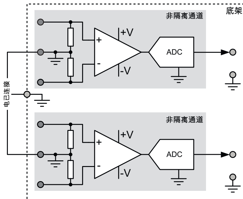
图 6: 接地图解
