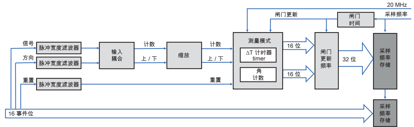
图 13: 计时器/计数器框图
