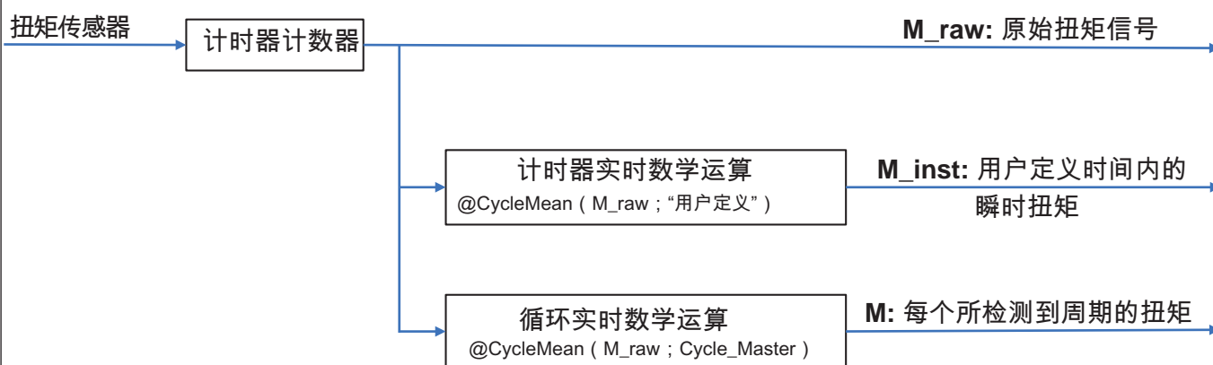
图 20: 同时动态的和精确的转矩计算
