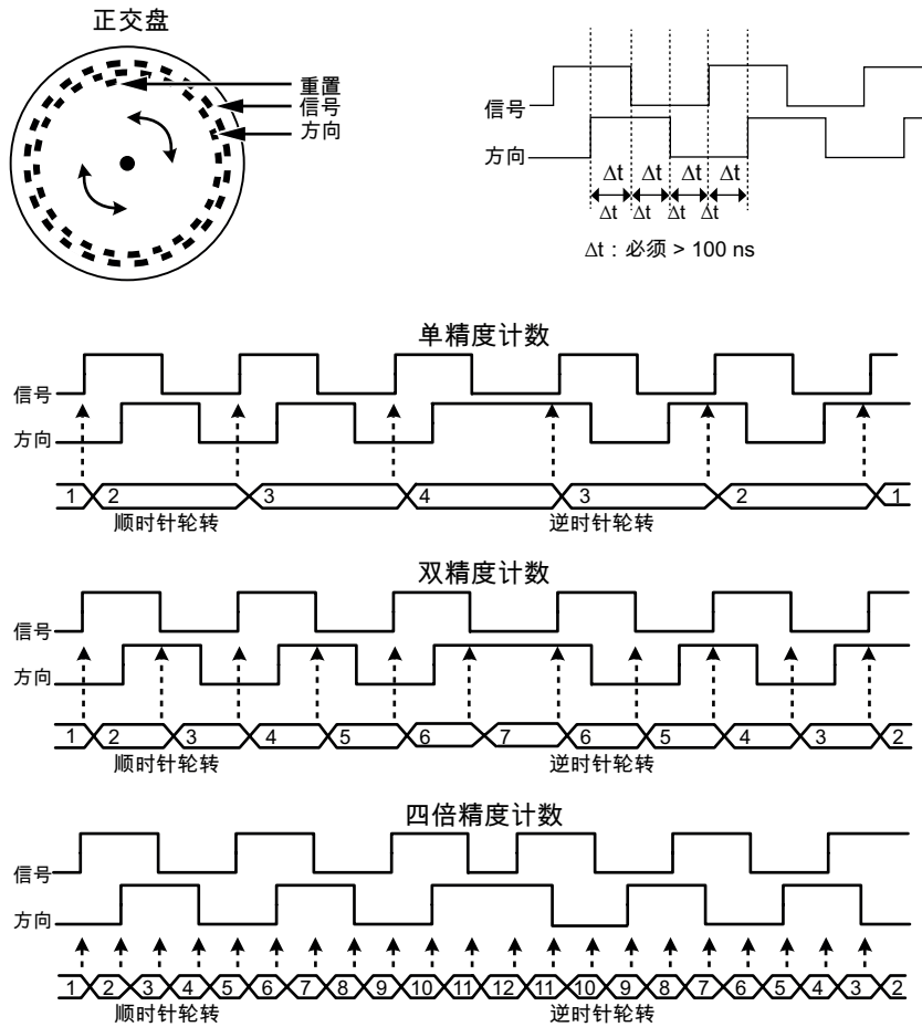
图 15: 双向正交计数模式
