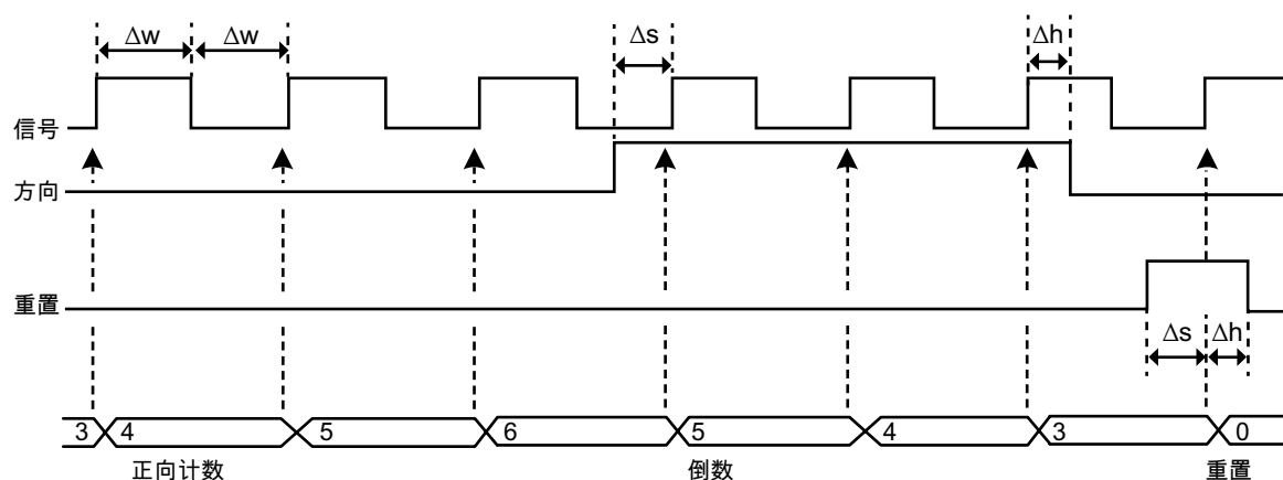
图 14: 单向和双向定时
