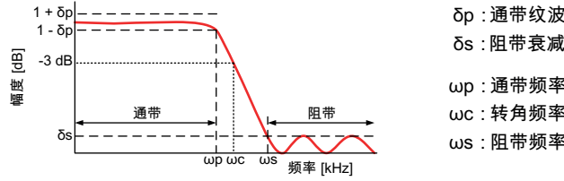
图 11: 数字巴特沃斯 IIR 滤波器
