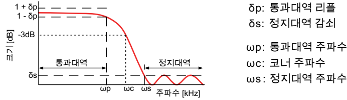
그림 9: 디지털 베셀 IIR 필터
