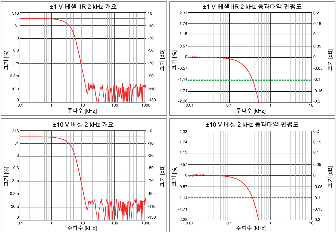
그림 10: 대표적 베셀 IIR 예시
