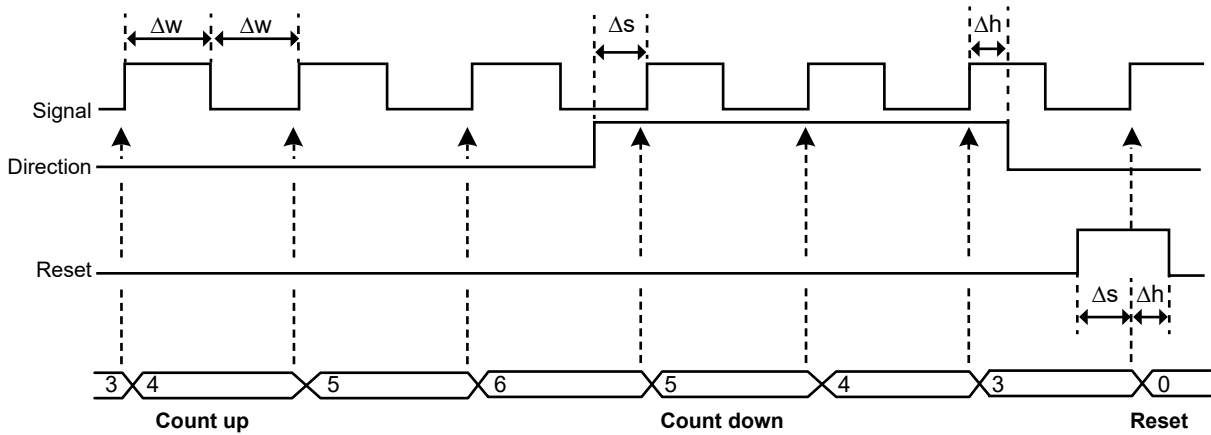
그림 14: 단방향 및 양방향 타이밍
