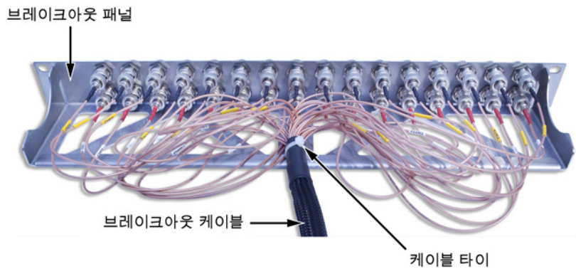
그림 25: 브레이크아웃 패널에 연결된 브레이크아웃 케이블
