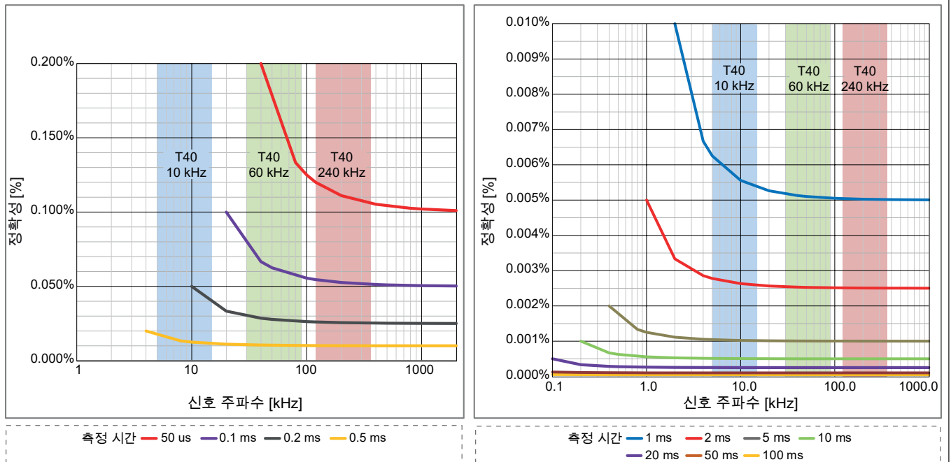
그림 18: 토크 작동 범위 대 부정확 및 측정 시간
