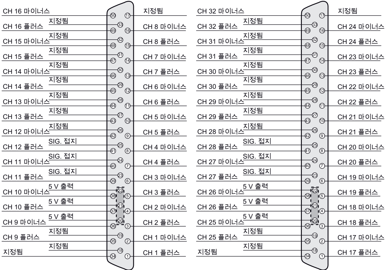
그림 21: 입력 커넥터 핀 다이어그램 (정면도)
