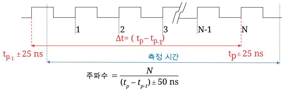
그림 16: 주파수 측정
