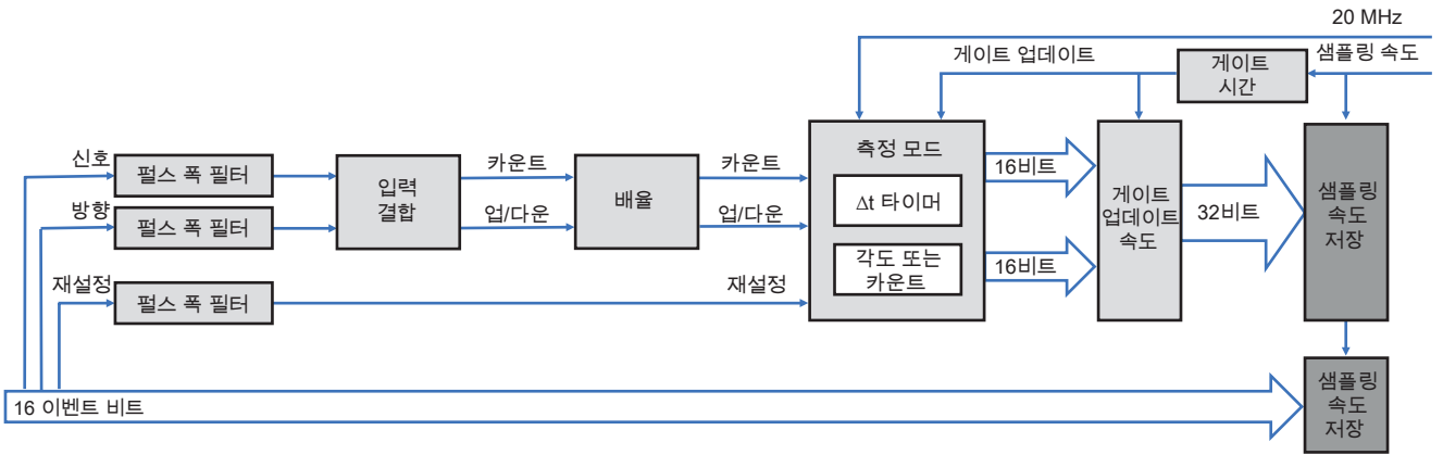
그림 13: 타이머/카운터 블록도
