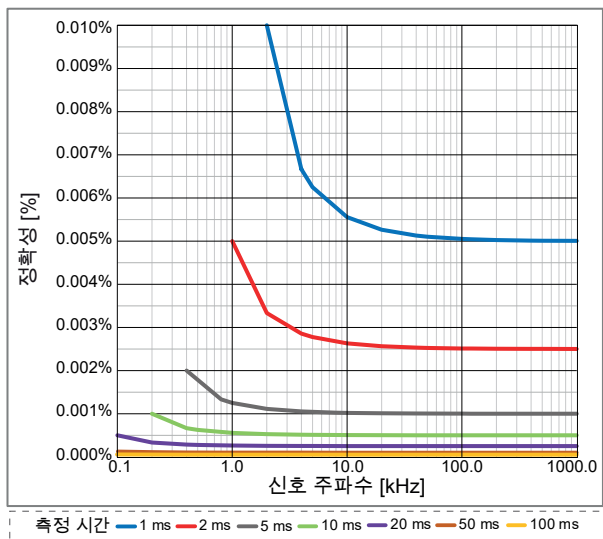
그림 17: 최대 타이머 부정확
