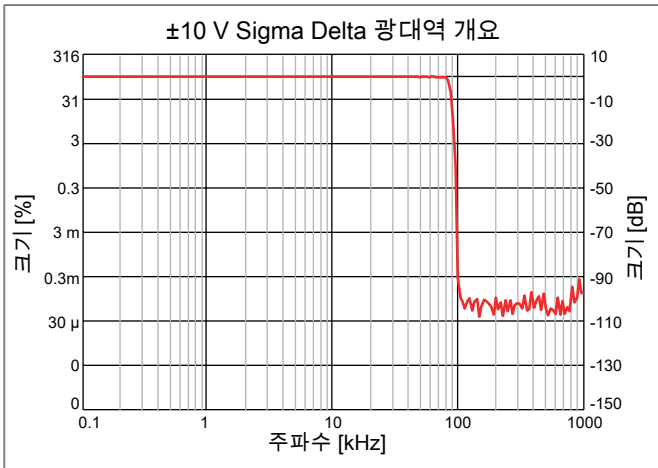
그림 8: 대표적 Sigma Delta 광대역 예시
