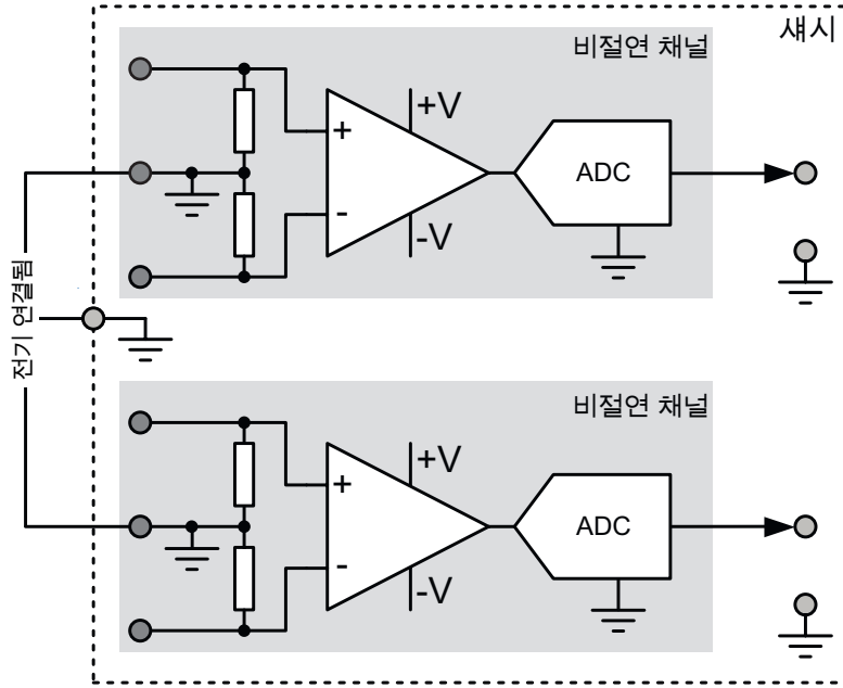
그림 6: 접지 회로도
