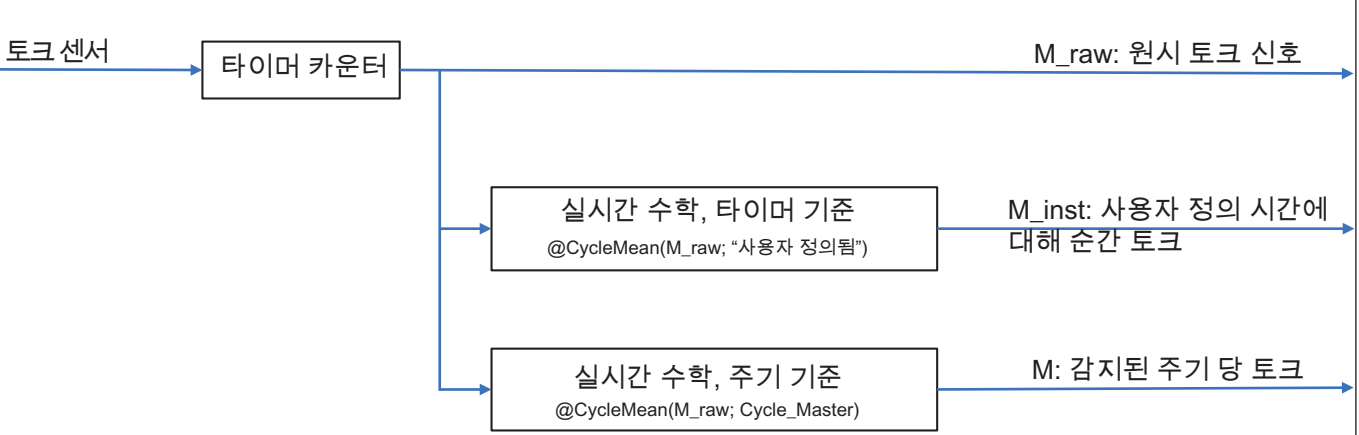
그림 20: 동시 동적 및 정확한 토크 계산
