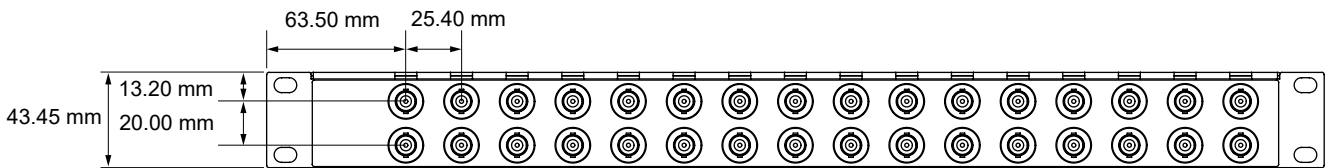
그림 24: 브레이크아웃 패널 치수
