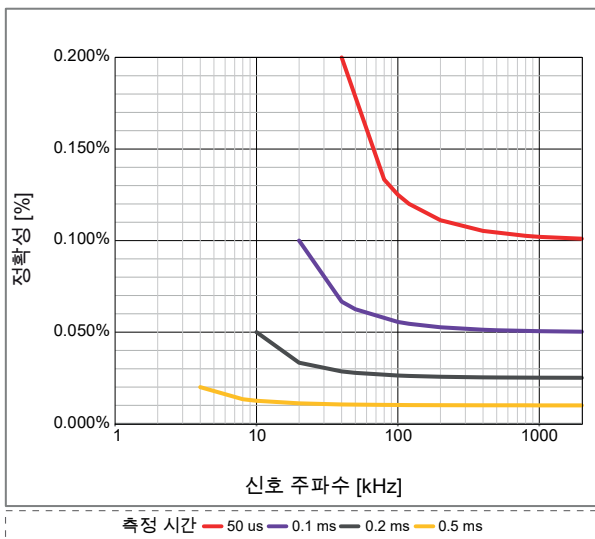
그림 17: 최대 타이머 부정확
