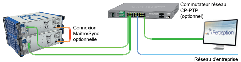
Figure 4 : Deux appareils de base
