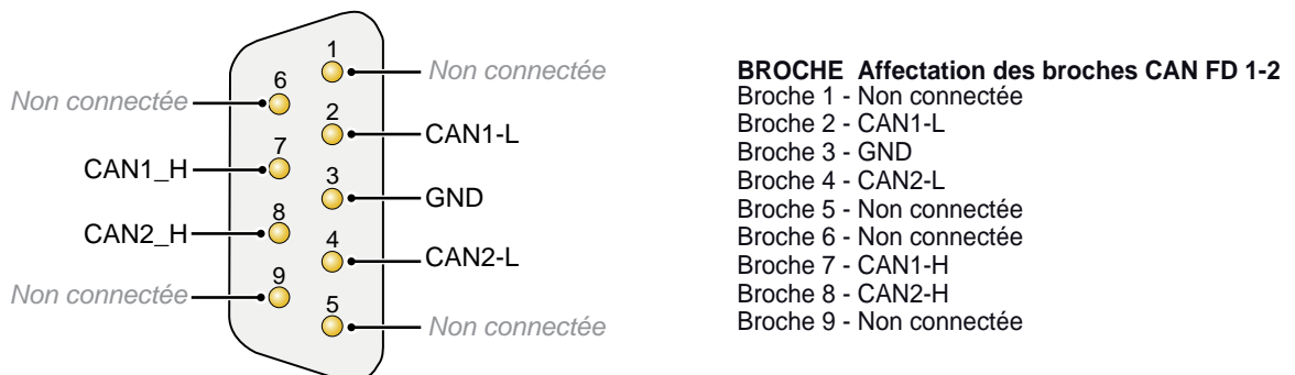
Figure 33 : Affectation des broches de l'option CAN FD
