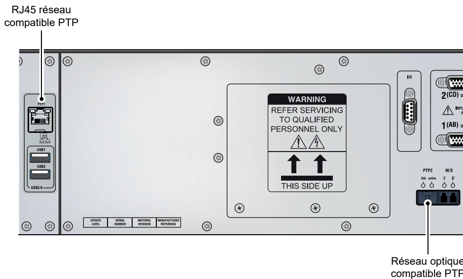
Figure 10 : Interfaces réseau électrique et optique 1 Gbit
