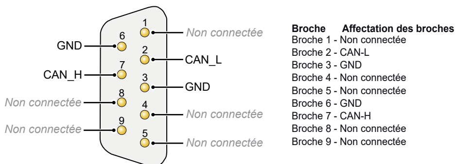
Figure 35 : Affectation des broches du connecteur D-Sub
