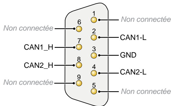
Figure 24 : Affectation des broches de l'option CAN FD
