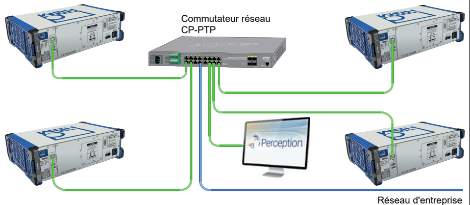
Figure 6 : Multiples appareils de base (distribués)
