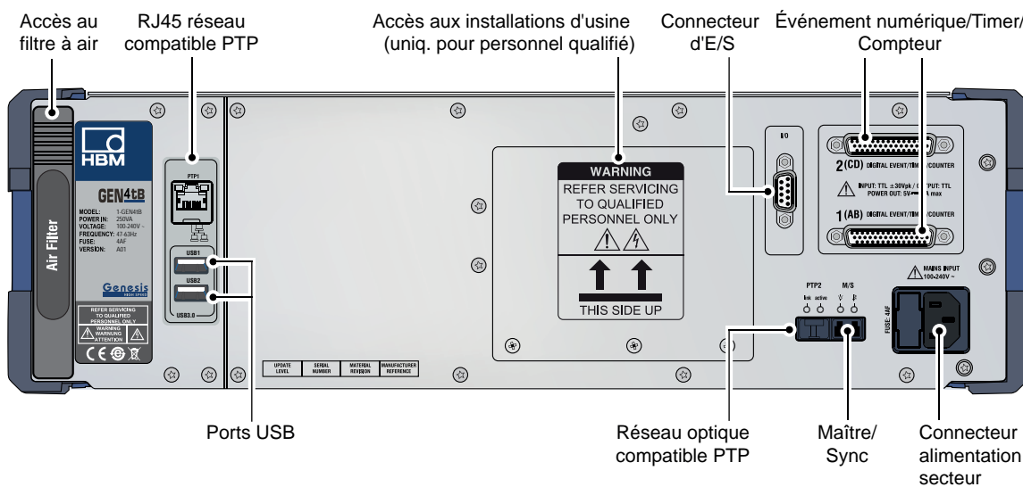
Figure 9 : Vue d'ensemble de la connectique sur la face arrière
