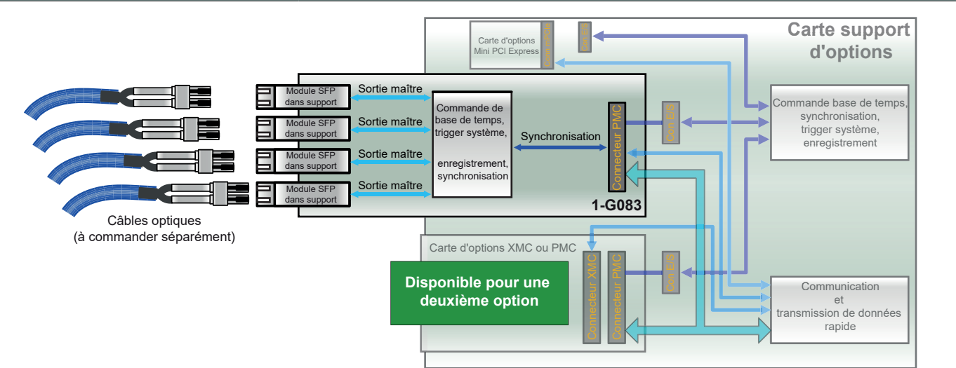
Figure 21 : Synoptique de la carte de sorties maîtres (carte G081 requise)
