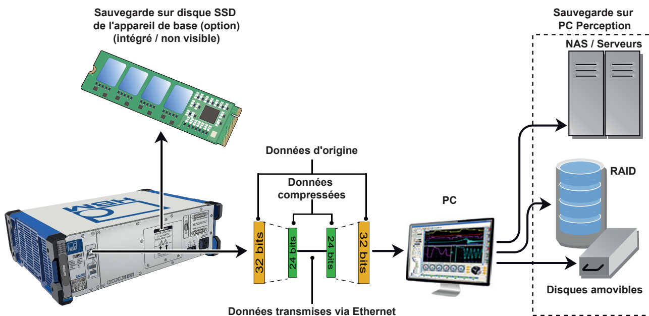
Figure 11 : Vue d'ensemble de la transmission continue
