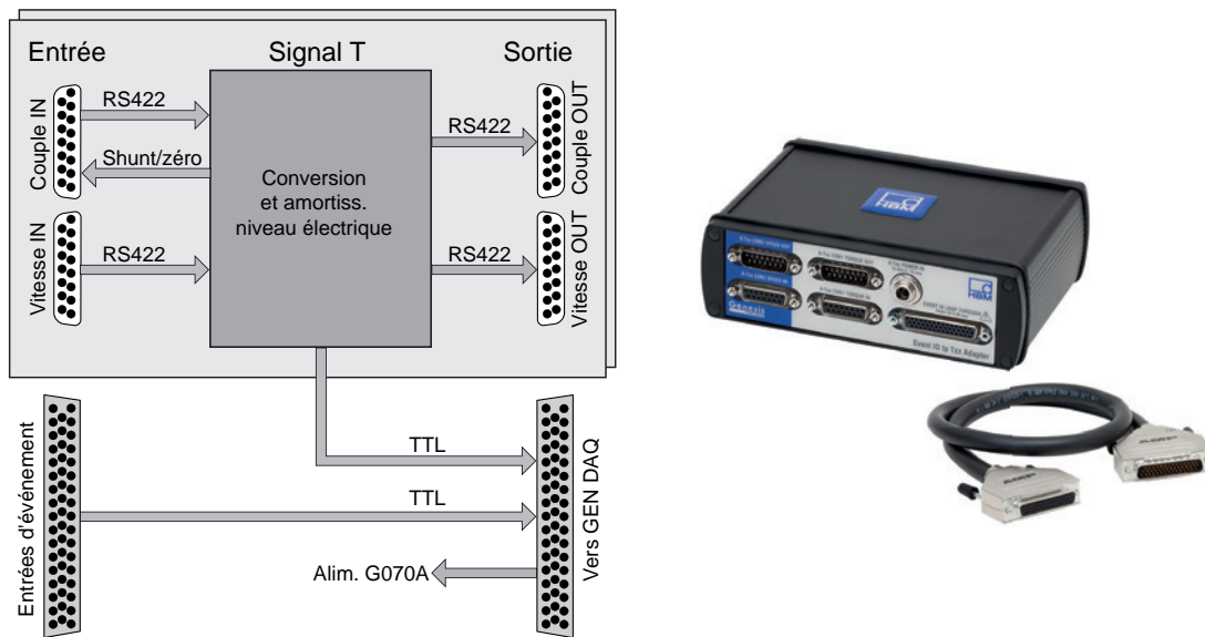
Figure 28 : Synoptique et photo
