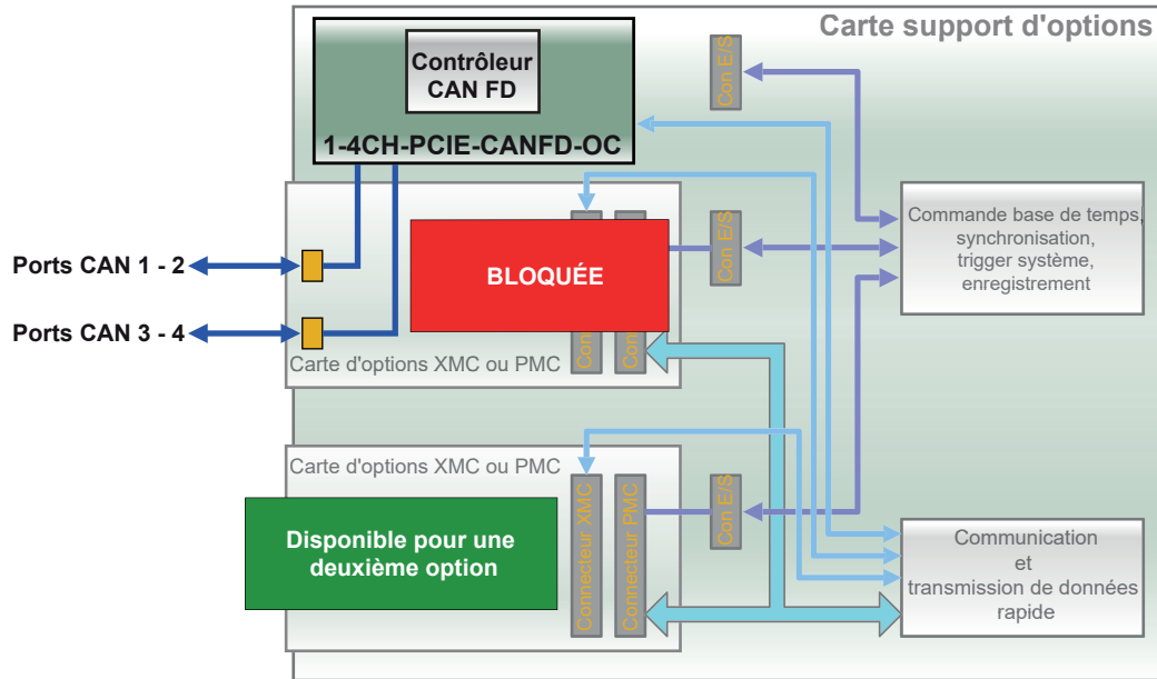
Figure 23 : Synoptique 1-4C-PCIE-CANFD-OC (carte G081 requise)
