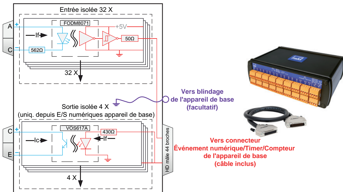
Figure 29 : Synoptique et photo
