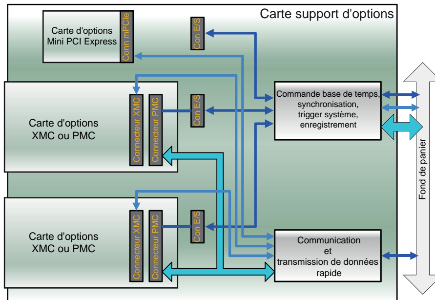
Figure 19 : Synoptique de la carte support d'options
