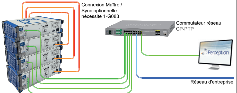
Figure 5 : Multiples appareils de base
