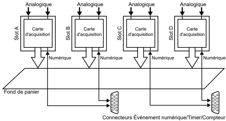
Figure 15 : Synoptique Événement numérique/Timer/Compteur
