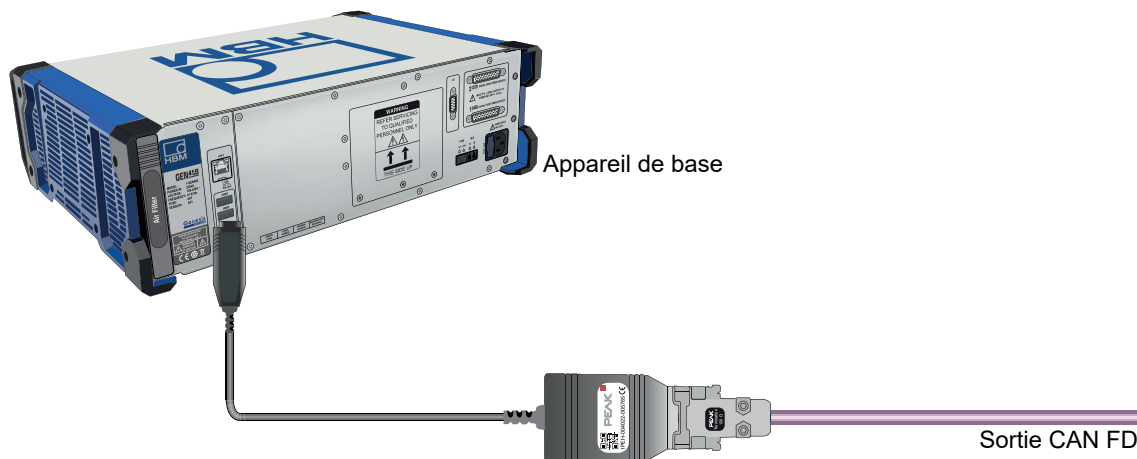
Figure 34 : Sortie CAN FD autonome du GEN4tB
