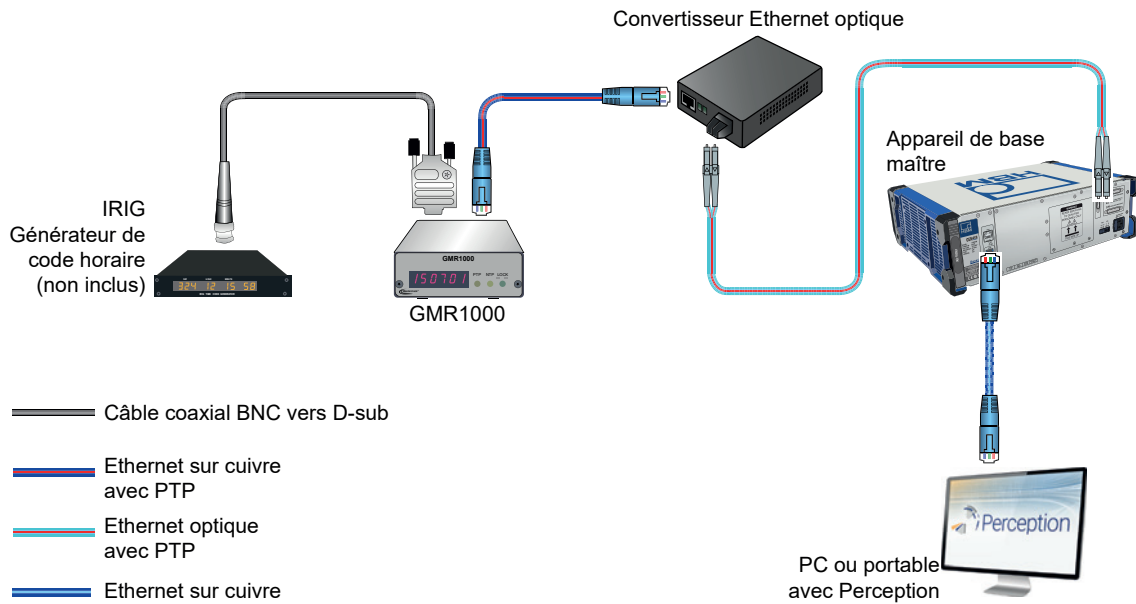
Figure 30 : Exemple de configuration de la synchronisation horaire IRIG
