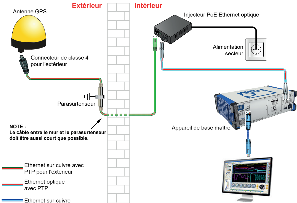
Figure 31 : Exemple de configuration de la synchronisation horaire GPS
