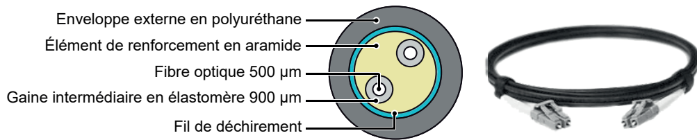
Figure 27 : Synoptique et photo
