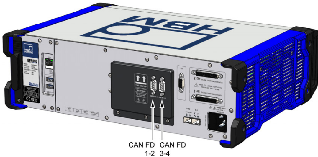
Figure 32 : GEN4tB avec pièce CAN FD installée (détail)
