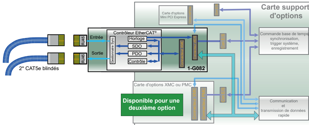
Figure 22 : Synoptique de la carte EtherCAT®
