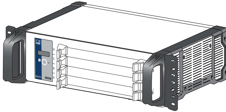
Figure 36 : Kit de montage en rack GEN4tB
