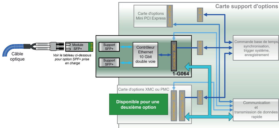
Figure 20 : Synoptique de la carte Ethernet 10 Gbit, optique (carte G081 requise)
