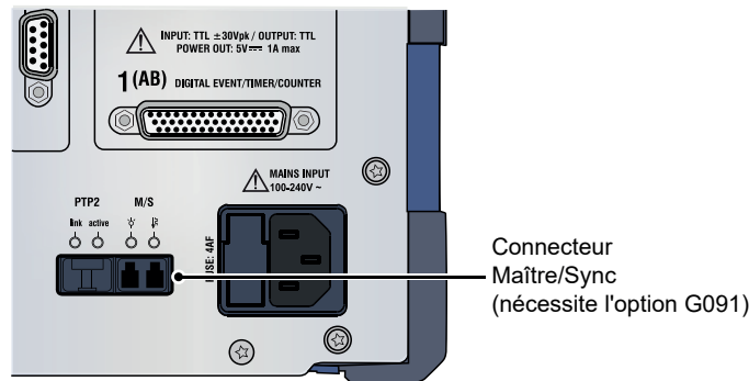
Figure 12 : Connecteur Maître/Sync
