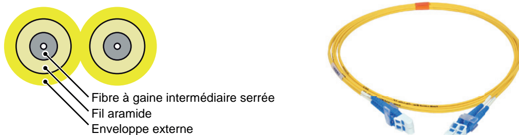
Figure 26 : Synoptique et photo
