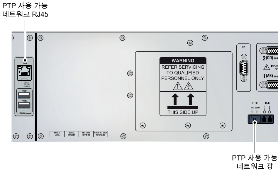
그림 10: 전기 및 광 1 Gbit 네트워크 인터페이스
