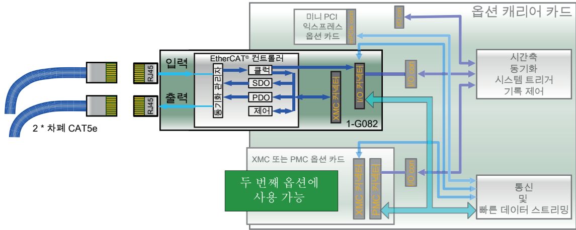
그림 22: 블록도 EtherCAT® 카드
