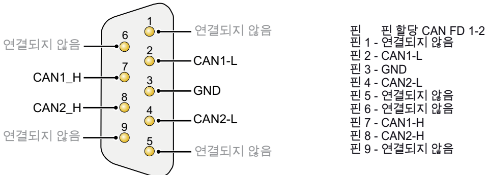
그림 33: 핀 할당 CAN FD 옵션
