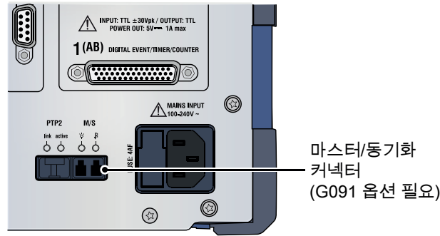
그림 12: 마스터/동기화 커넥터
