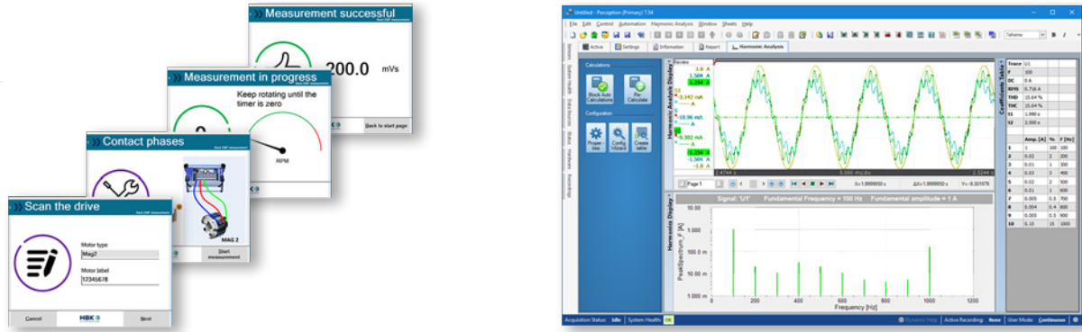
그림 40: Perception CSI 예시 BackEMF (왼쪽) 조화 분석 (오른쪽)
