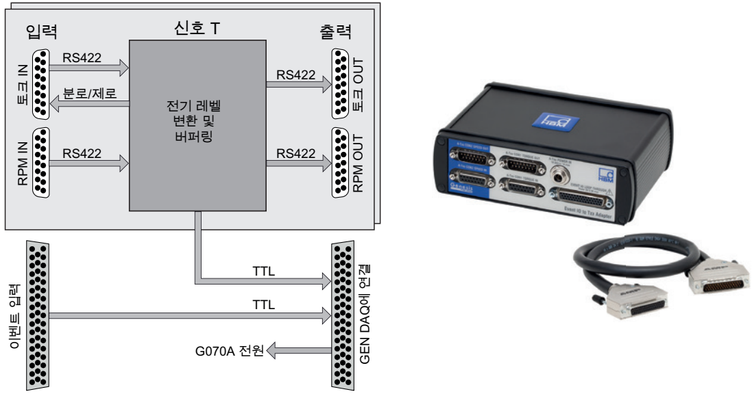
그림 28: 블록도 및 이미지
