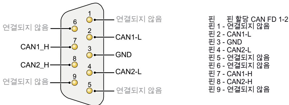
그림 24: 핀 할당 CAN FD 옵션
