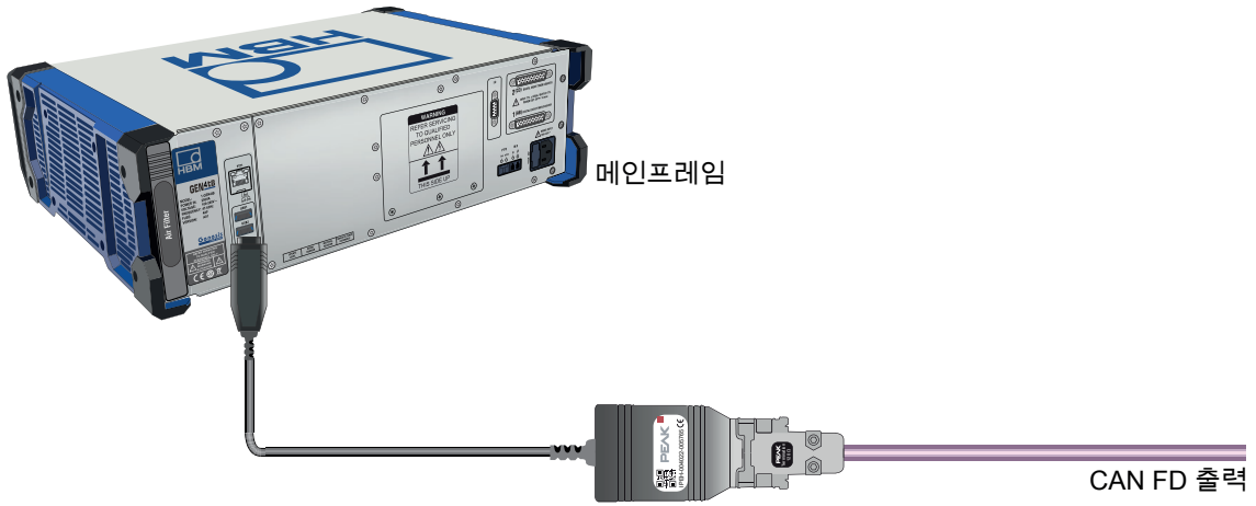
그림 34: GEN4tB 독립형 CAN FD 출력
