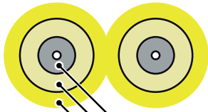
타이트 버퍼 섬유 아라미드 원사 외장 재킷
