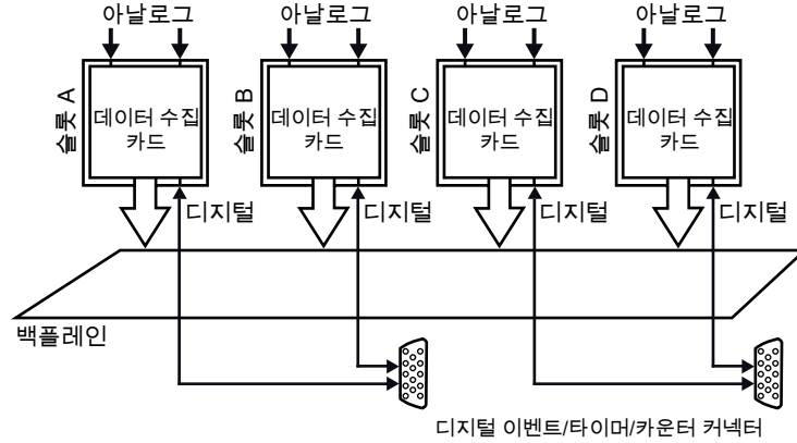
그림 15: 디지털 이벤트/타이머/카운터 블록도
