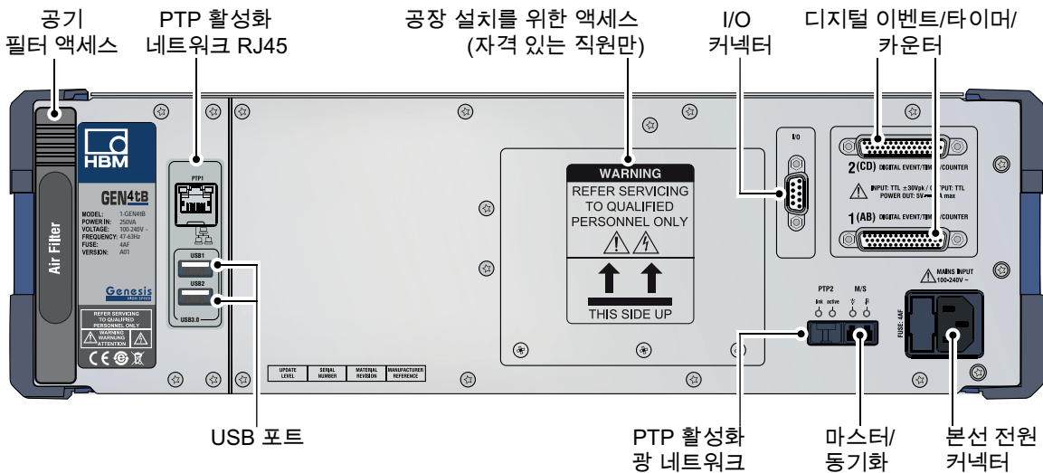
그림 9: 배면도 연결 개요
