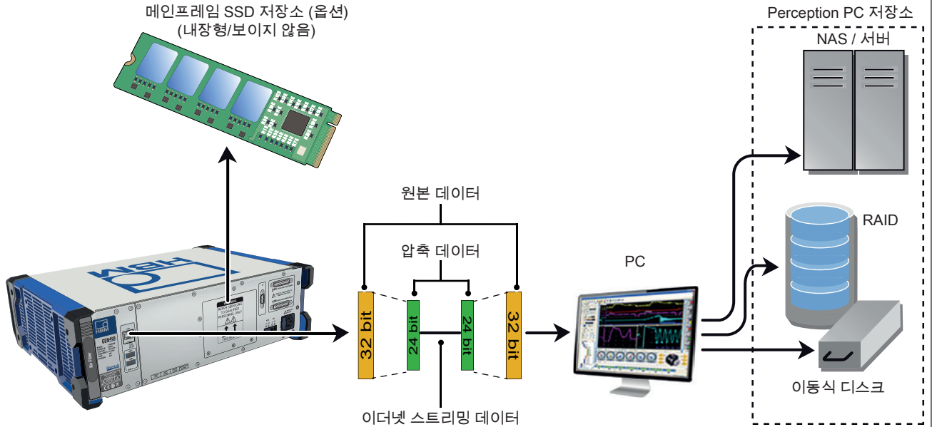
그림 11: 연속 스트리밍 개요
