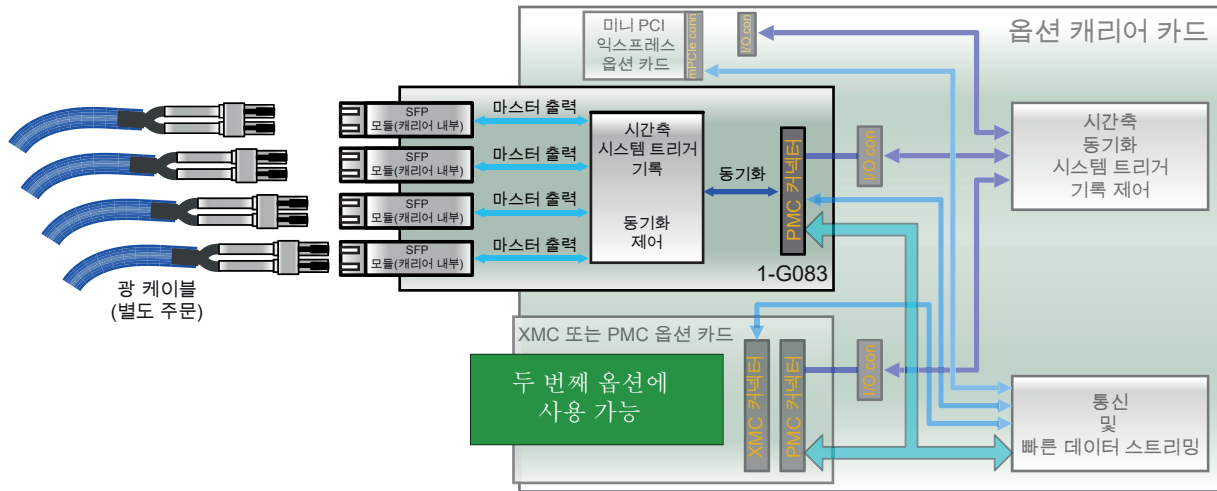
그림 21: 블록도 마스터 출력 카드 (G081 필요)
