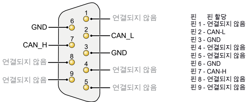
그림 35: 핀 할당 D-Sub
