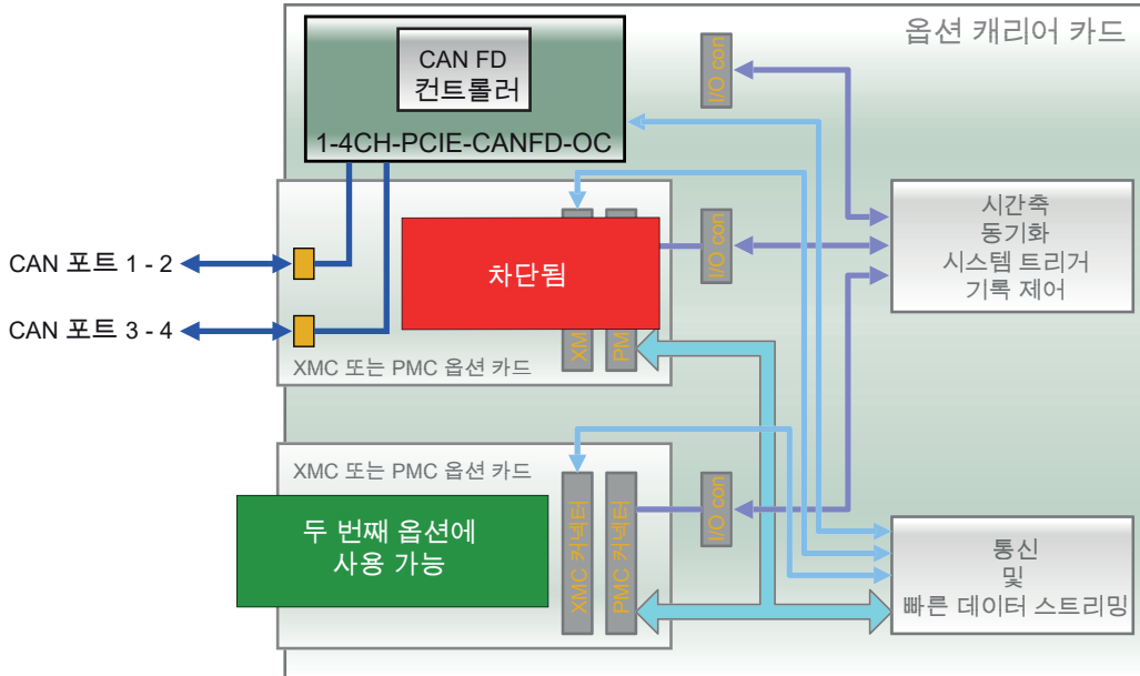
그림 23: 블록도 1-4C-PCIE-CANFD-OC (G081 필요)
