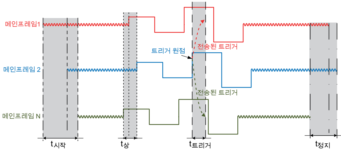
그림 13: 동기화 사양 개요
