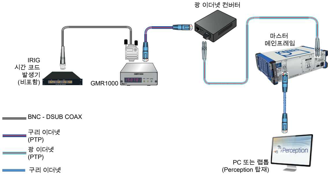
그림 30: 예제 설정 IRIG 시간 동기화
