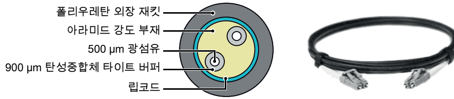
그림 27: 블록도 및 이미지
