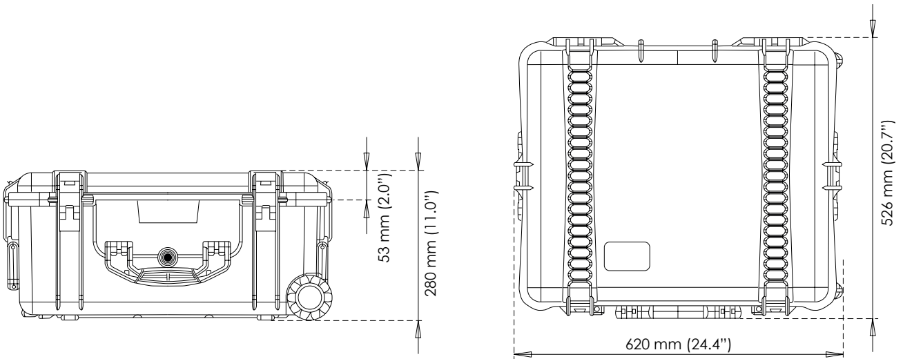
그림 37: 재활용 가능 하드커버 배송 케이스(휠 및 운송 핸들 포함)
