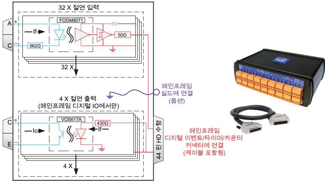
그림 29: 블록도 및 이미지
