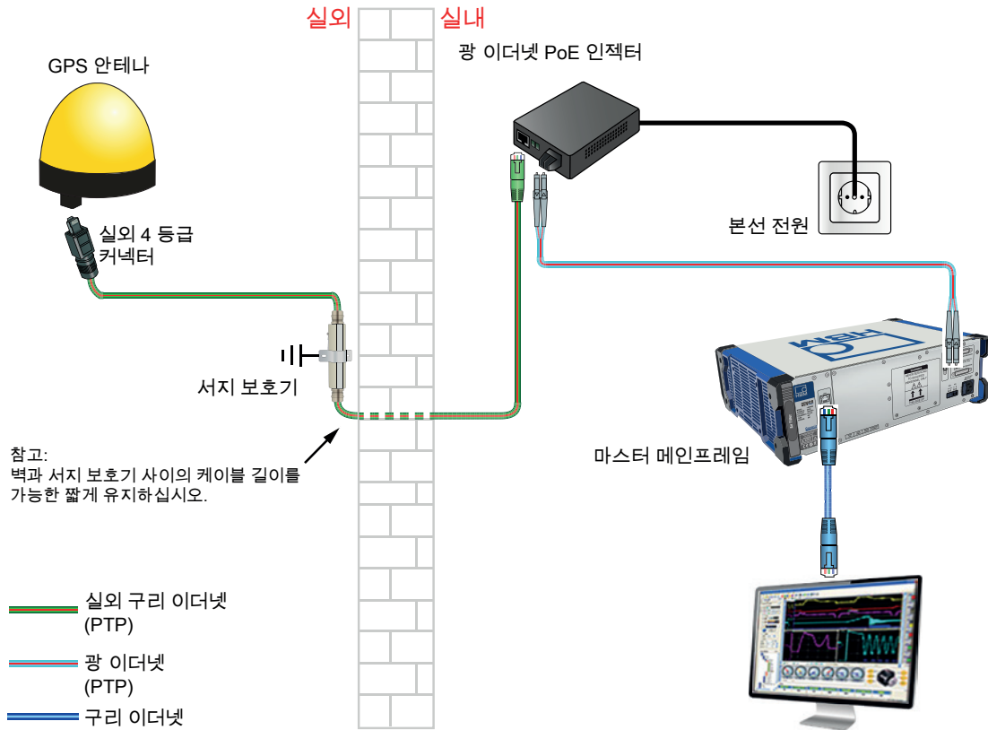
그림 31: 예제 설정 GPS 시간 동기화
