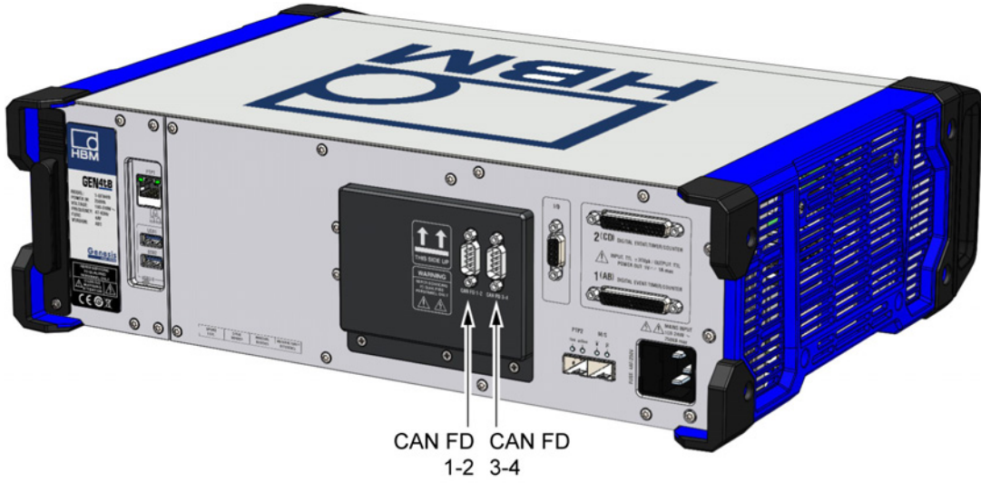
그림 32: GEN4tB, 설치된 CAN FD 상단 부분(세부) 포함
