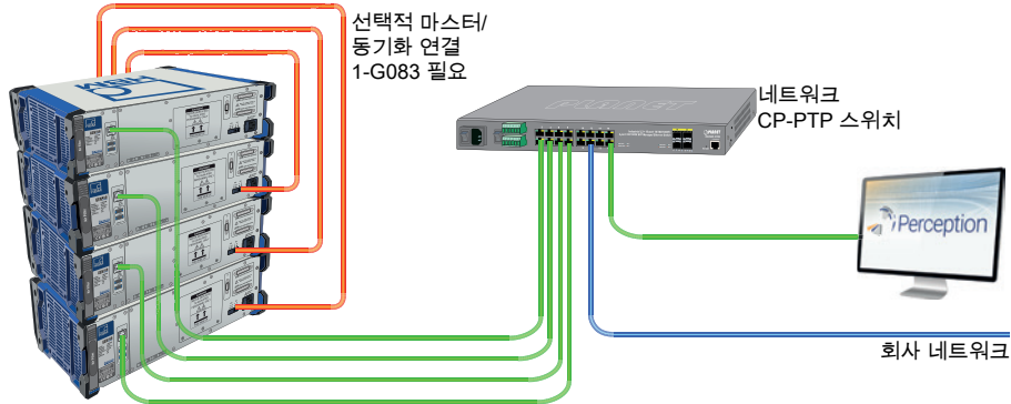
그림 5: 멀티 메인프레임
