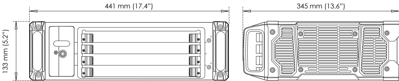
그림 1: GEN4tB 치수
