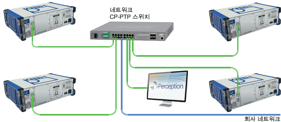
그림 6: 멀티 메인프레임 (분산)
