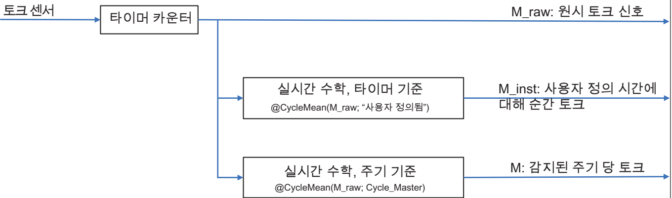
그림 40: 동시 동적 및 정확한 토크 계산
