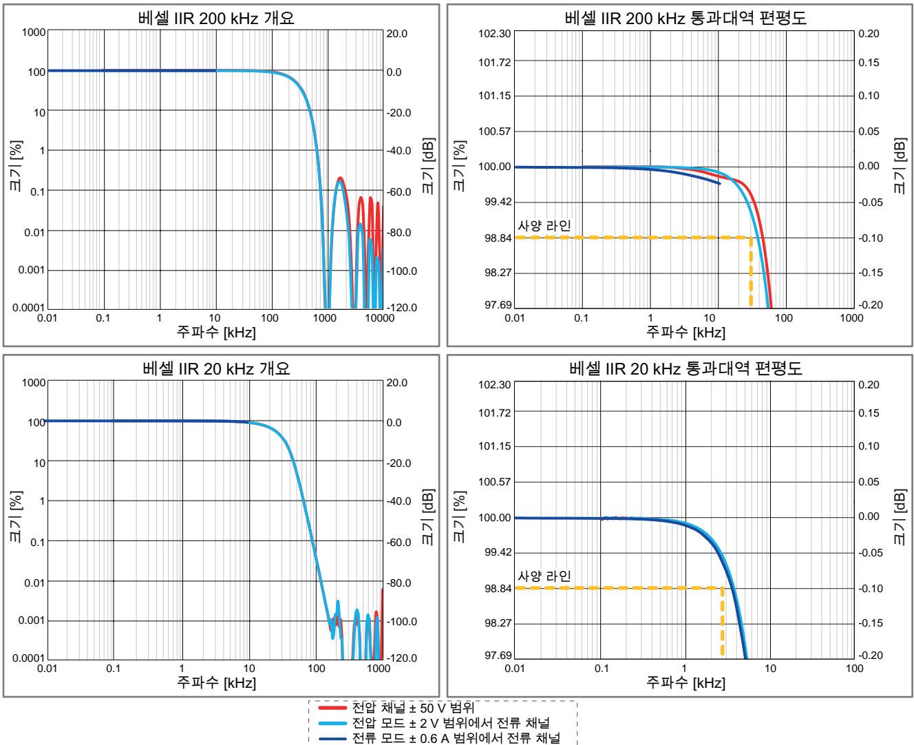
그림 27: 대표적 베셀 IIR 예제 (GN310B의 경우만 200 kHz; GN310B 및 GN311B의 경우 20 kHz)
