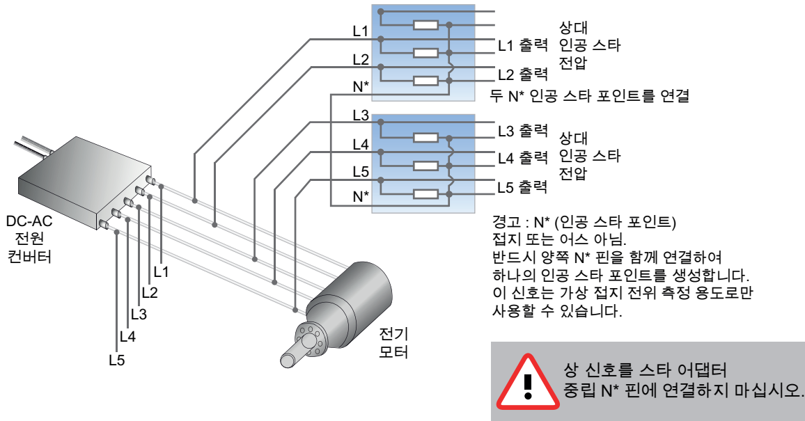
그림 43: 이중 스타 어댑터의 5 상 이상 대표적 사용
