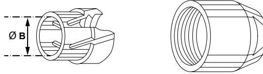
그림 15: 케이블 콜릿 설정
