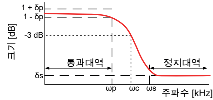
그림 22: 베셀 필터
