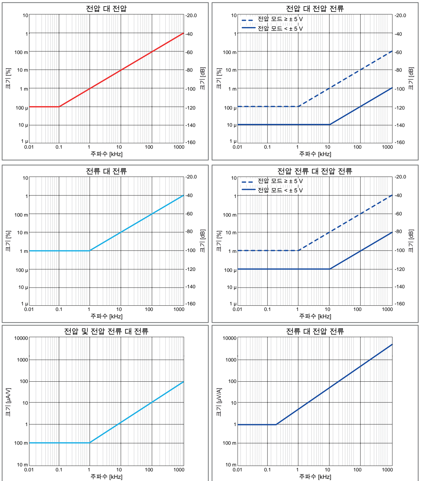
그림 32: 대표적 채널 대 채널 크로스토크
