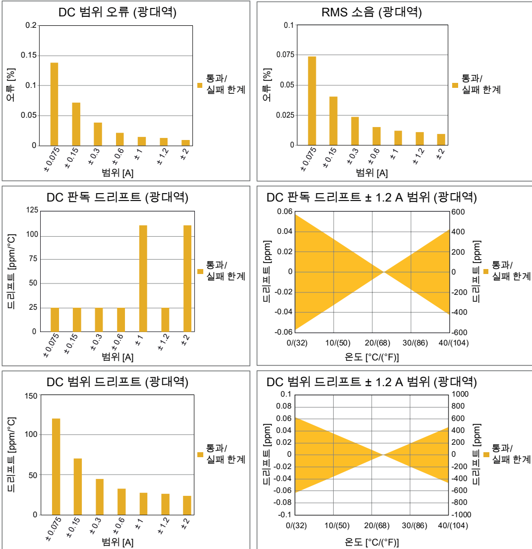
그림 9: 광대역 전류 모드 사양
