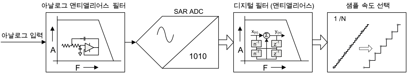
그림 20: 결합된 아날로그 및 디지털 앤티앨리어스 필터 블록도
