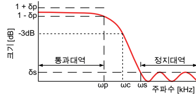
그림 26: 대표적 베셀 IIR 예제 (GN310B의 경우만 200 kHz; GN310B 및 GN311B의 경우 20 kHz)
