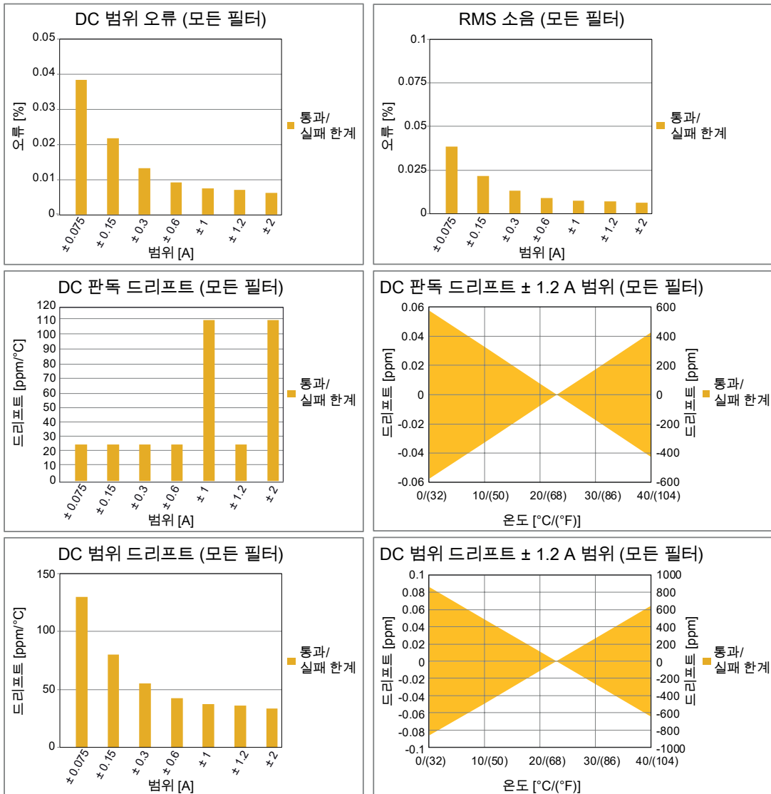
그림 10: 모든 필터 사용 전류 모드 사양
