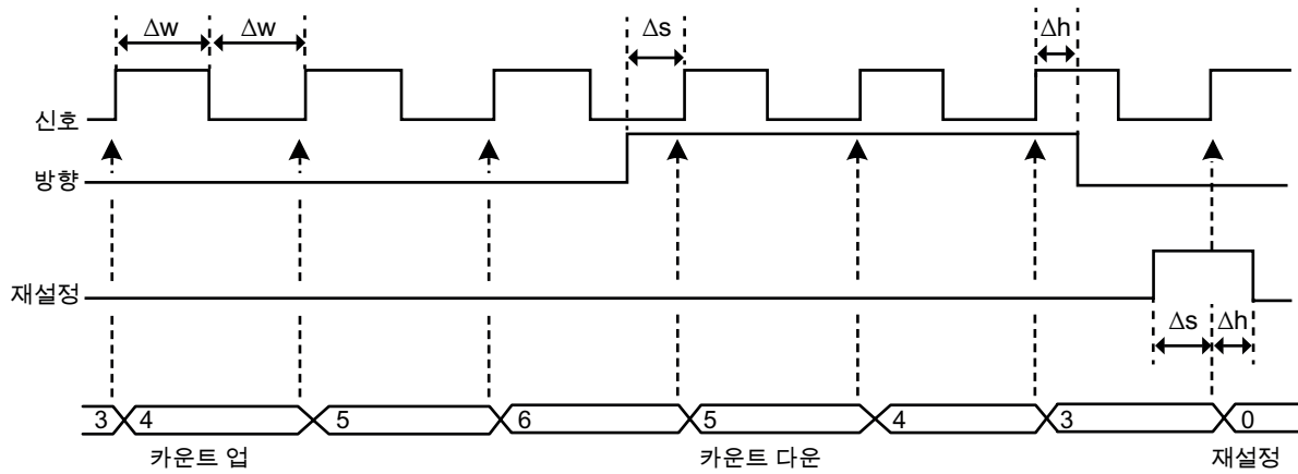
그림 34: 단방향 및 양방향 타이밍
