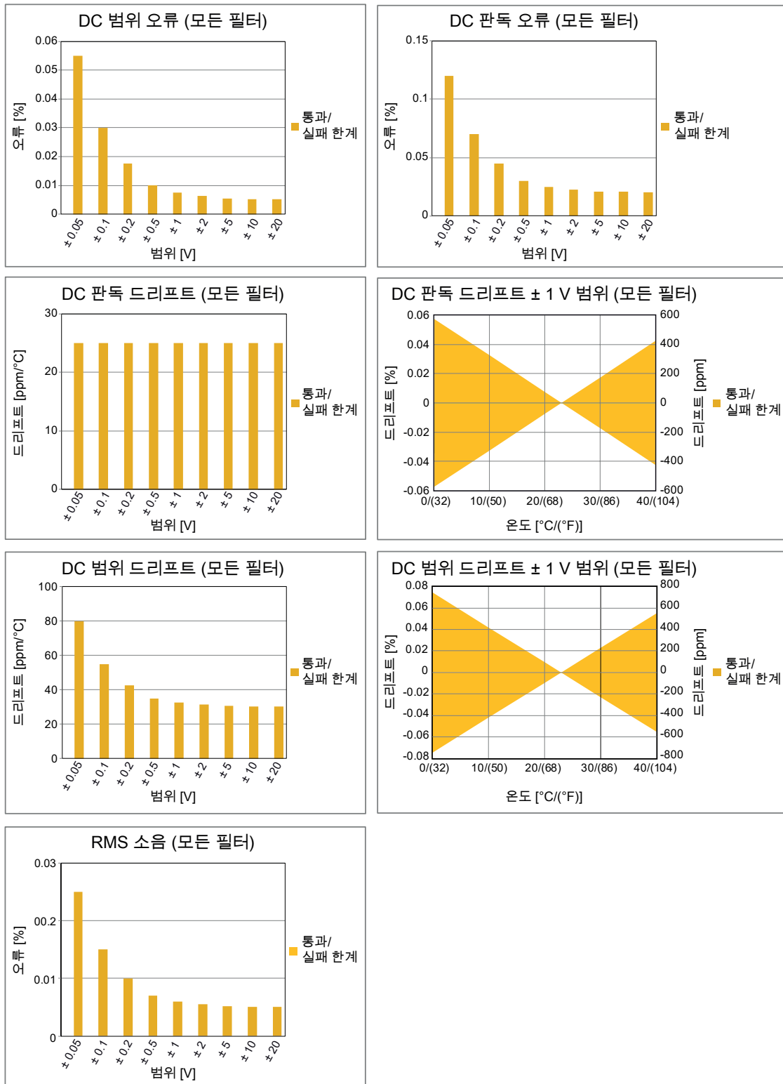
그림 13: 모든 필터 사용 전압 모드 사양
