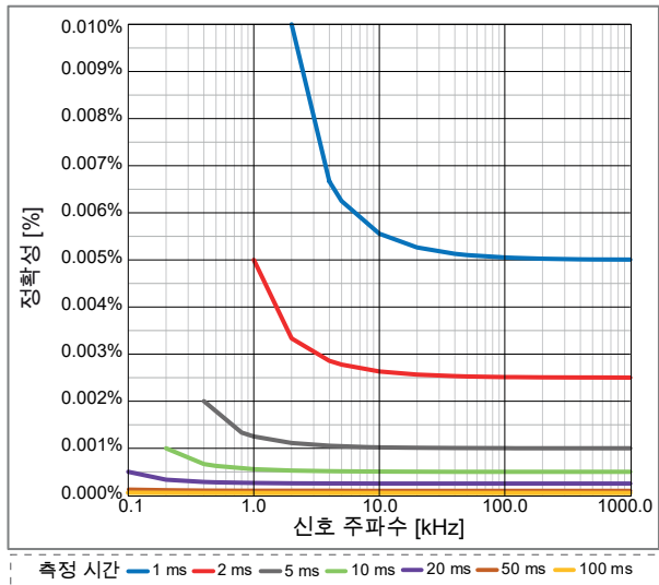
그림 37: 최대 타이머 부정확
