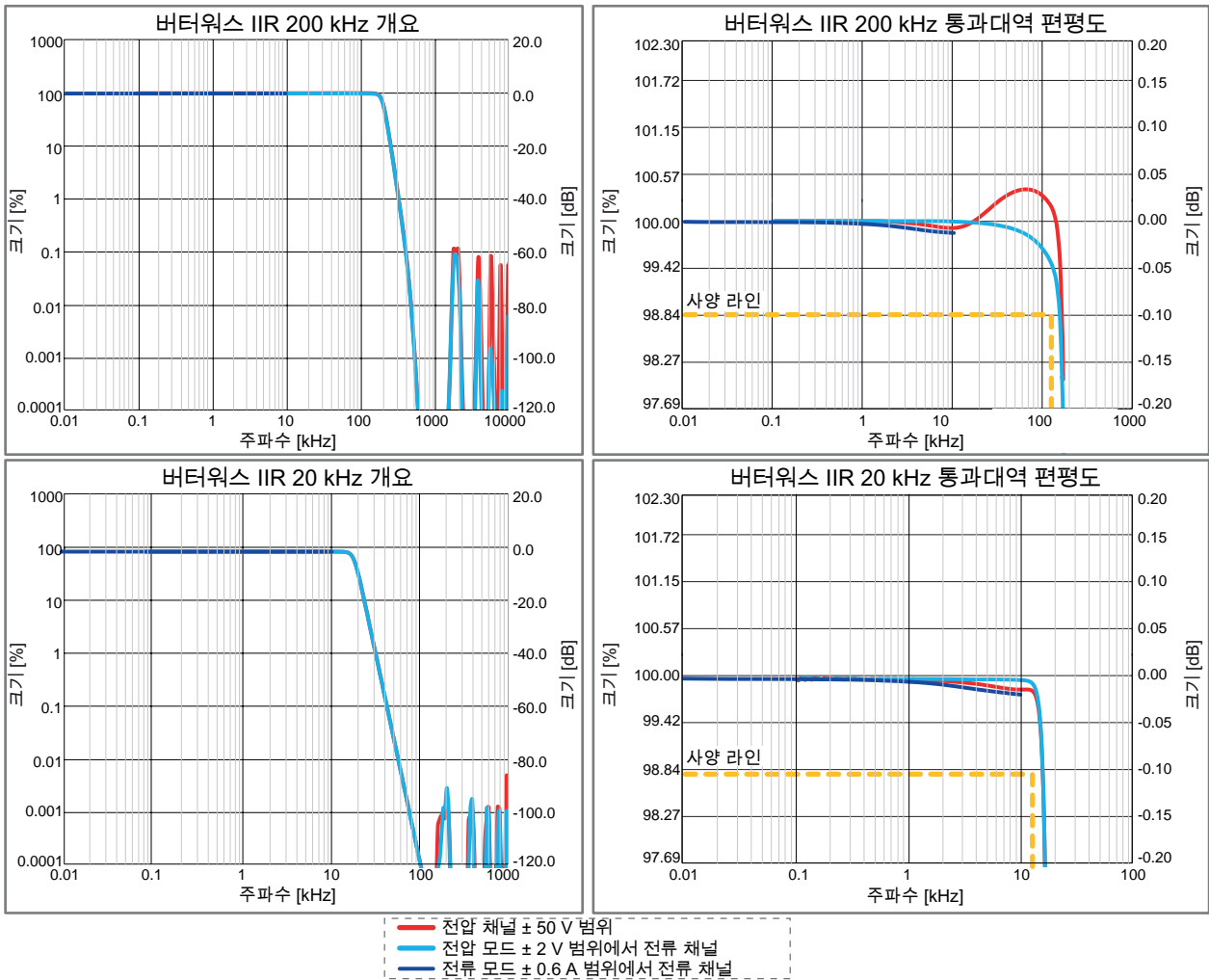
그림 29: 대표적 버터워스 IIR 예제 (GN310B의 경우만 200 kHz; GN310B 및 GN311B의 경우 20 kHz)
