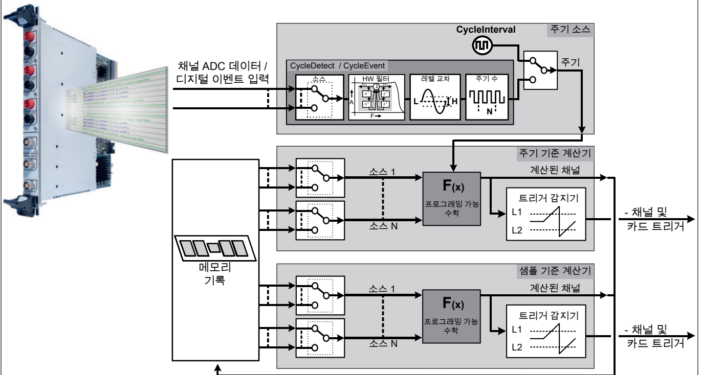
그림 41: 실시간 포뮬라 데이터베이스(formula database) (RT-FDB) 계산기
