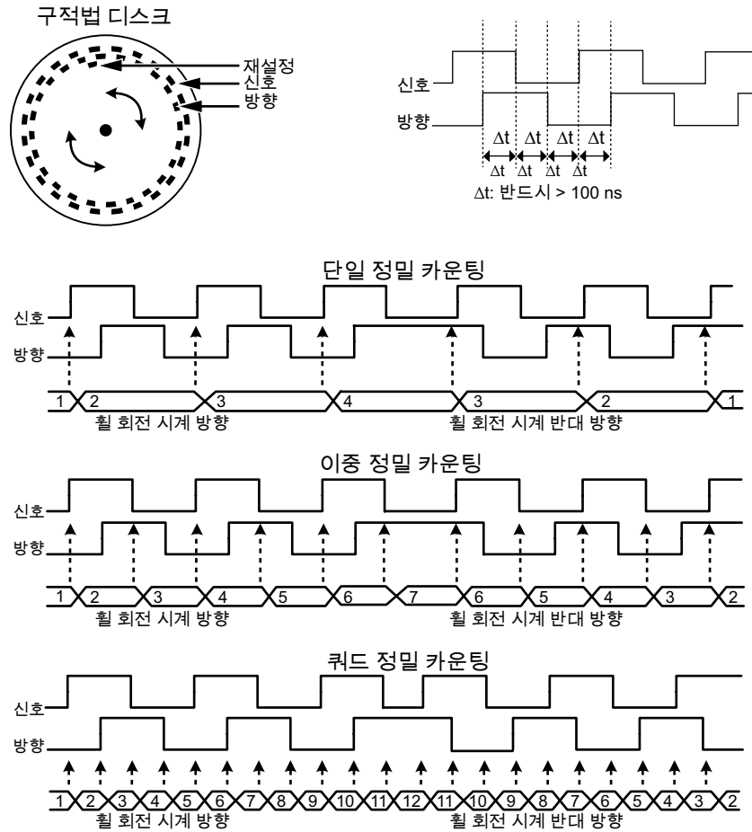
그림 35: 양방향 구적법(quadrature) 카운트 모드
