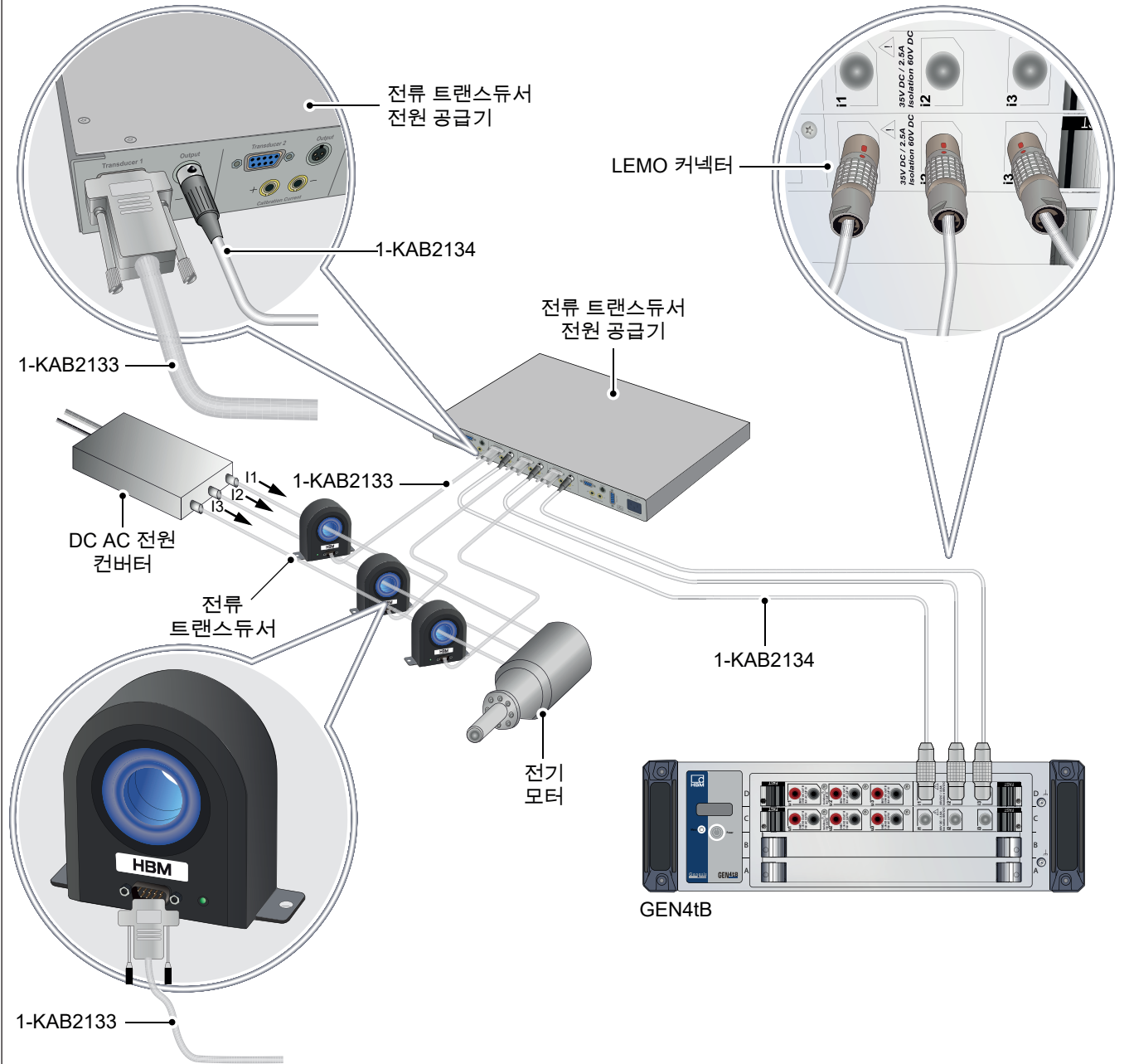
그림 46: 전류 트랜스듀서 연결도
