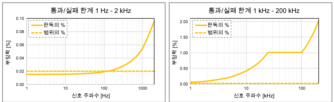
그림 4: 전원 통과/실패 한계 (0.33 Ω 션트), 광대역 및 0.5 ≤ 역률 ≤ 1
