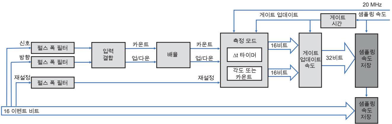
그림 33: 타이머/카운터 블록도
