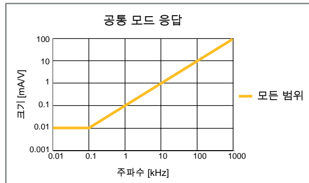
그림 8: 공통 모드 응답 (전류 채널: 전류 모드)
