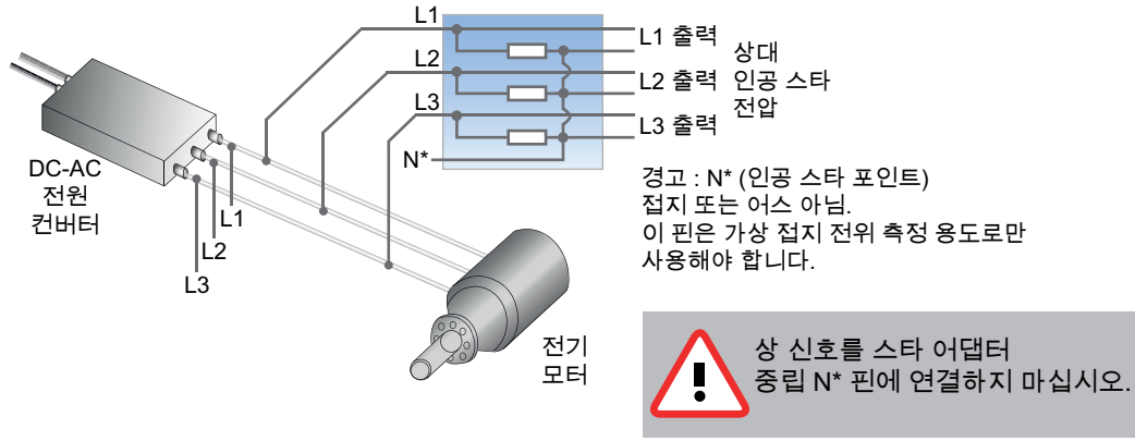
그림 42: 인공 스타 어댑터의 3 상 대표적 사용
