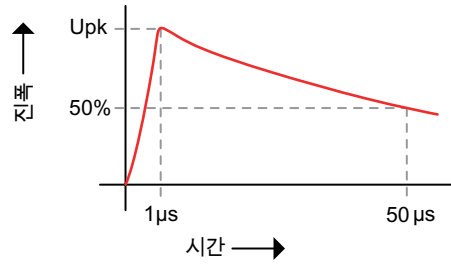
그림 19: 1.2/50 μs 임펄스 예
