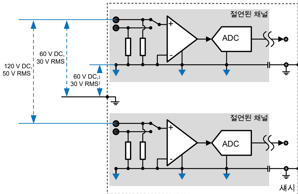
그림 18: 전류 채널 절연 등급
