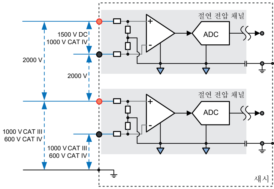
그림 17: 전압 채널 절연 등급
