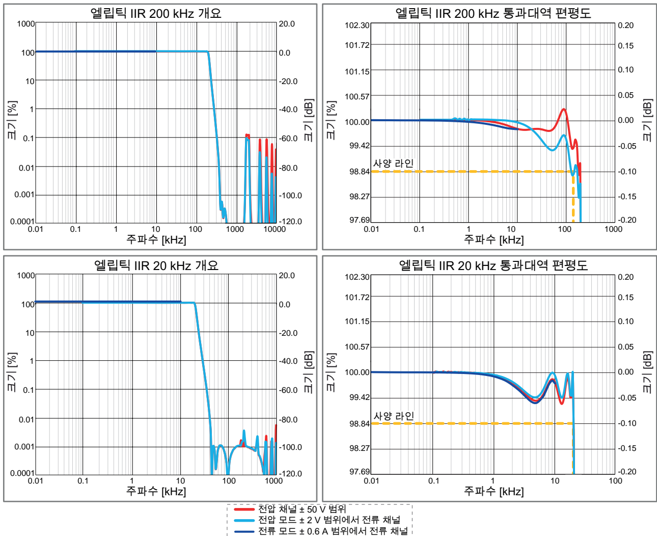
그림 31: 대표적 엘리틱 IIR 예제 (GN310B의 경우만 200 kHz; GN310B 및 GN311B의 경우 20 kHz)
