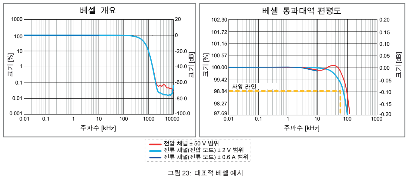
그림 23: 대표적 베셀 예시
