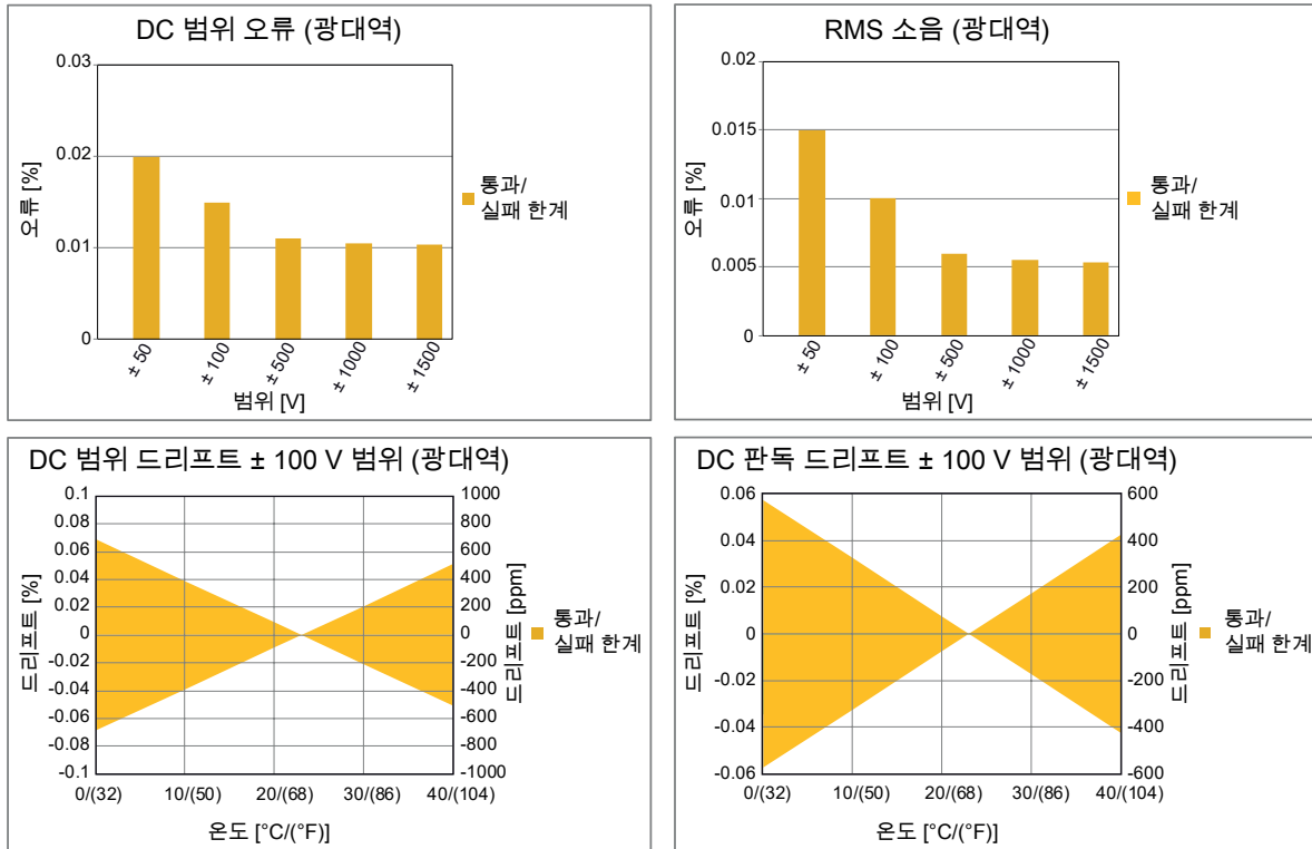
그림 6: 광대역 전압 사양
