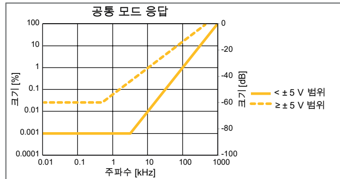
그림 11: 공통 모드 응답 (전류 채널: 전압 모드)
