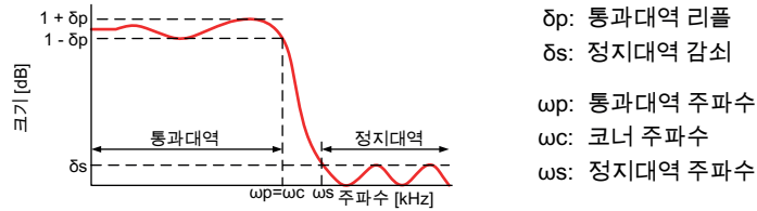
그림 30: 디지털 엘리틱 IIR 필터
