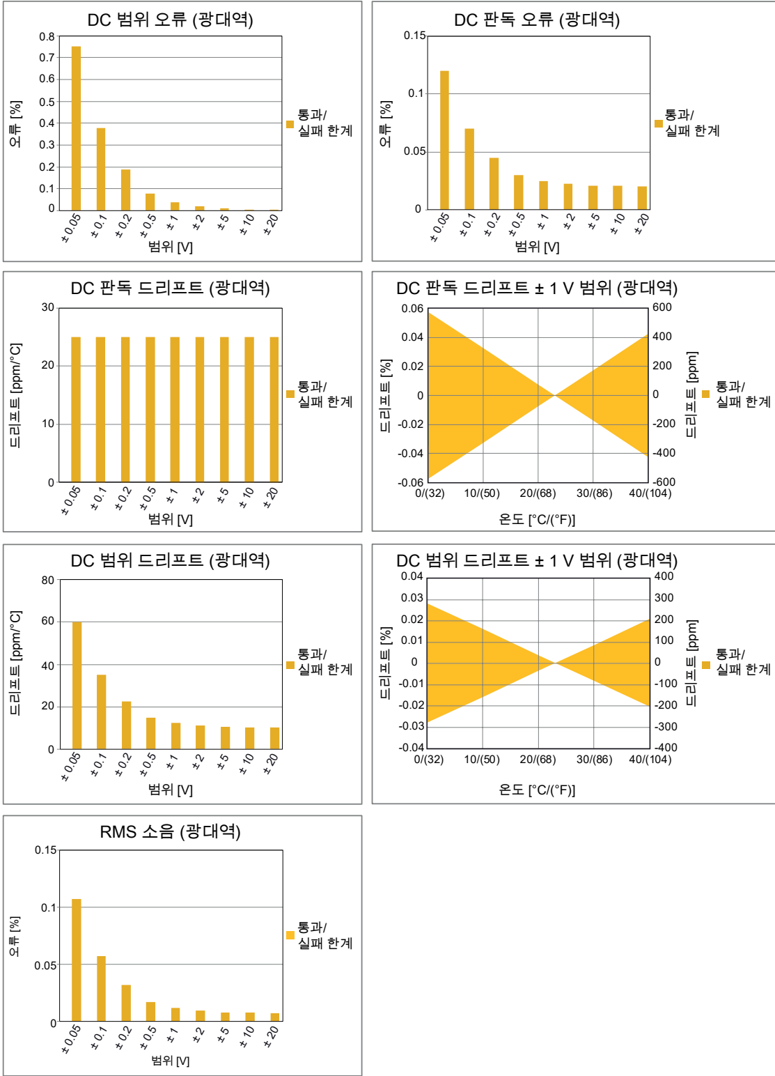
그림 12: 광대역 전압 모드 사양
