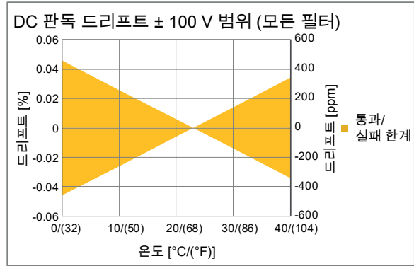
그림 7: 사용된 모든 필터 전압 사양
