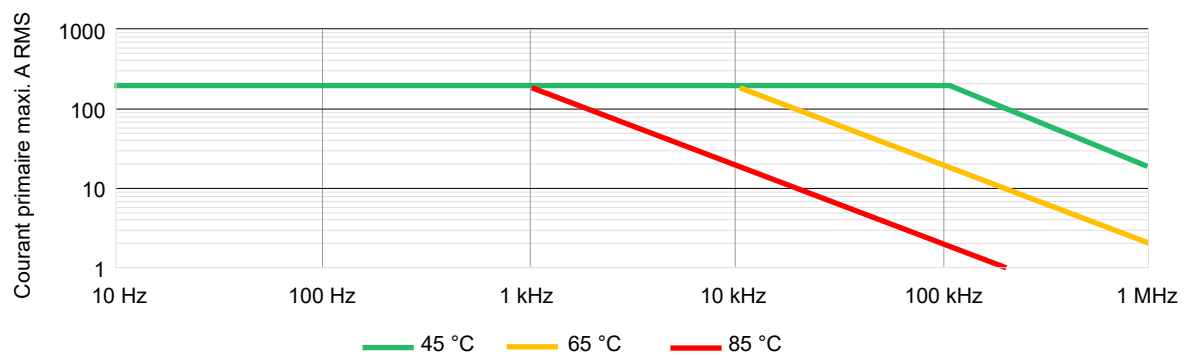
Figure 1.2 : Fréquence et limitation de la température ambiante
