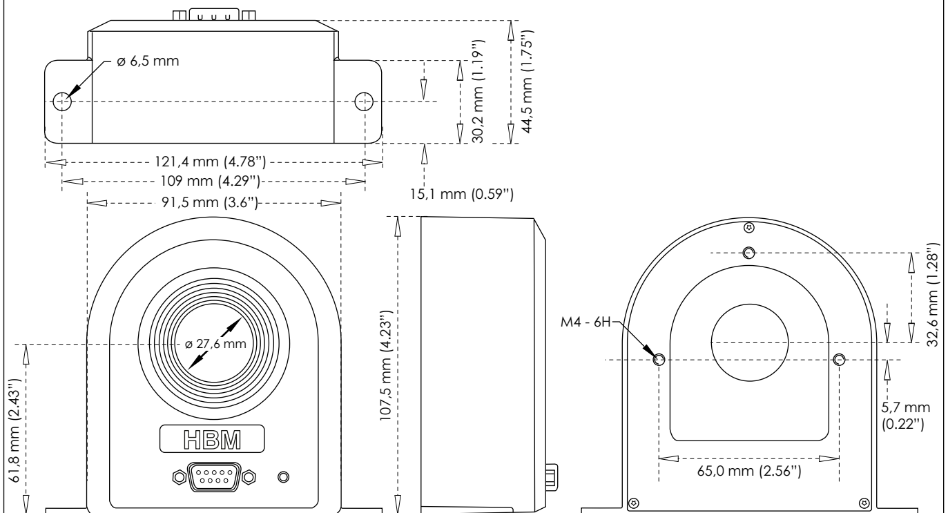
Abbildung 1.5: Abmessungen CTS50/200ID/400ID/600ID
