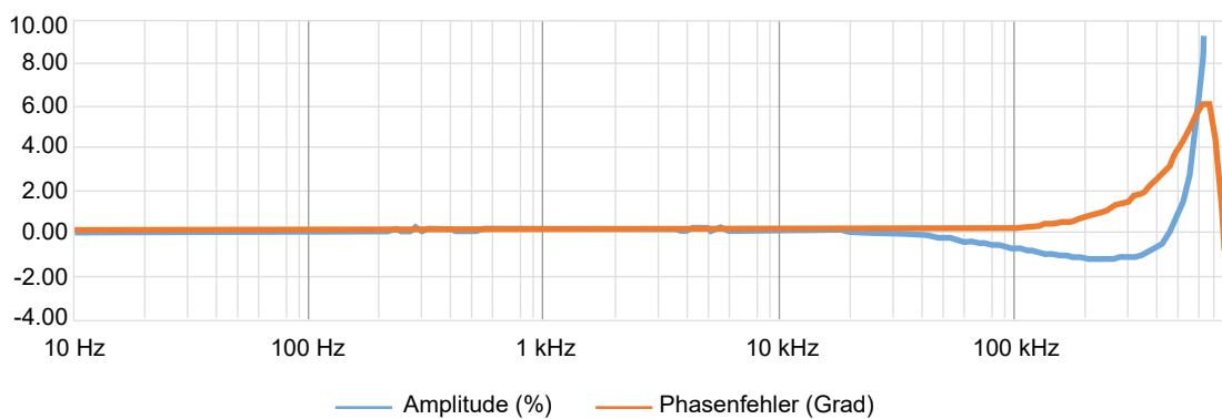
Abbildung 1.3: Frequenzkennlinie
