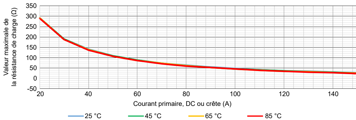
Figure 1.1 : Résistance de charge RM et limitation de la température ambiante
