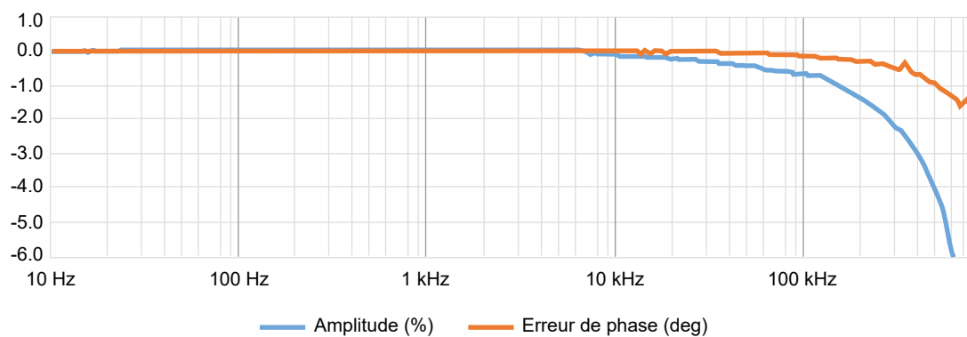
Figure 1.3 : Caractéristiques en fonction de la fréquence
