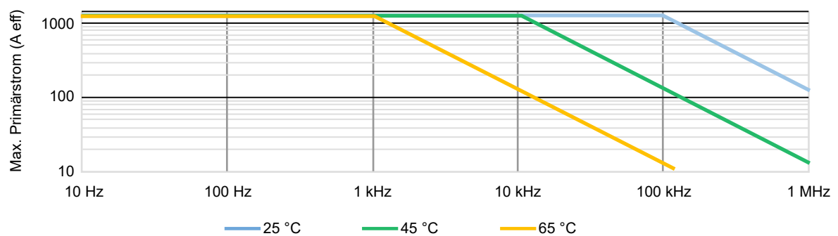
Abbildung 1.2: Herabsetzung der Nennwerte durch Frequenz und Umgebungstemperatur
