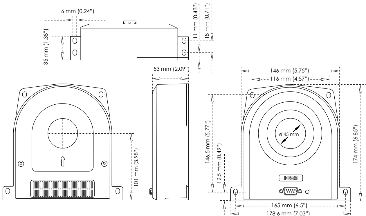
Abbildung 1.5: Abmessungen CTM1200ID/CTM1200ID-CD3000
