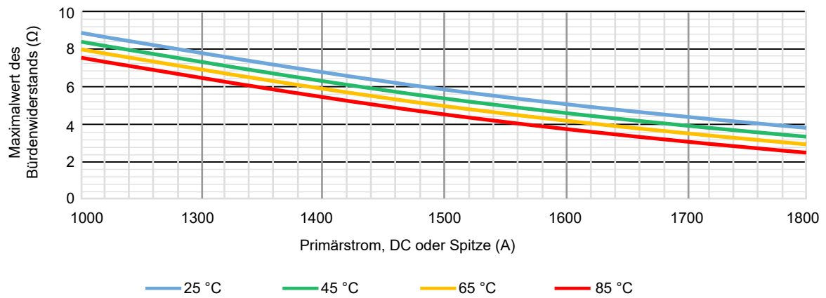
Abbildung 1.1: Herabsetzung der Nennwerte durch Bürdenwiderstand RM und Umgebungstemperatur
