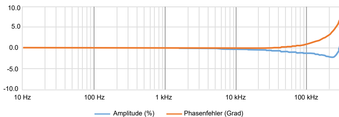
Abbildung 1.3: Frequenzkennlinie
