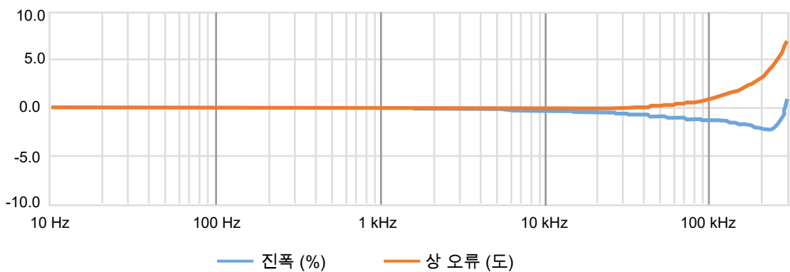
그림 1.3: 주파수 특성
