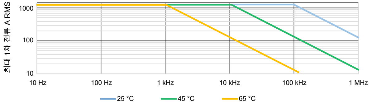
그림 1.2: 주파수 및 주변 온도 경감
