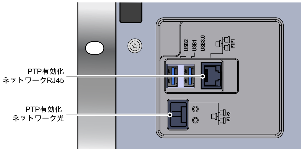
図 1.8: 電子式および光学式 1Gbit ネットワーク・ インタフェース
