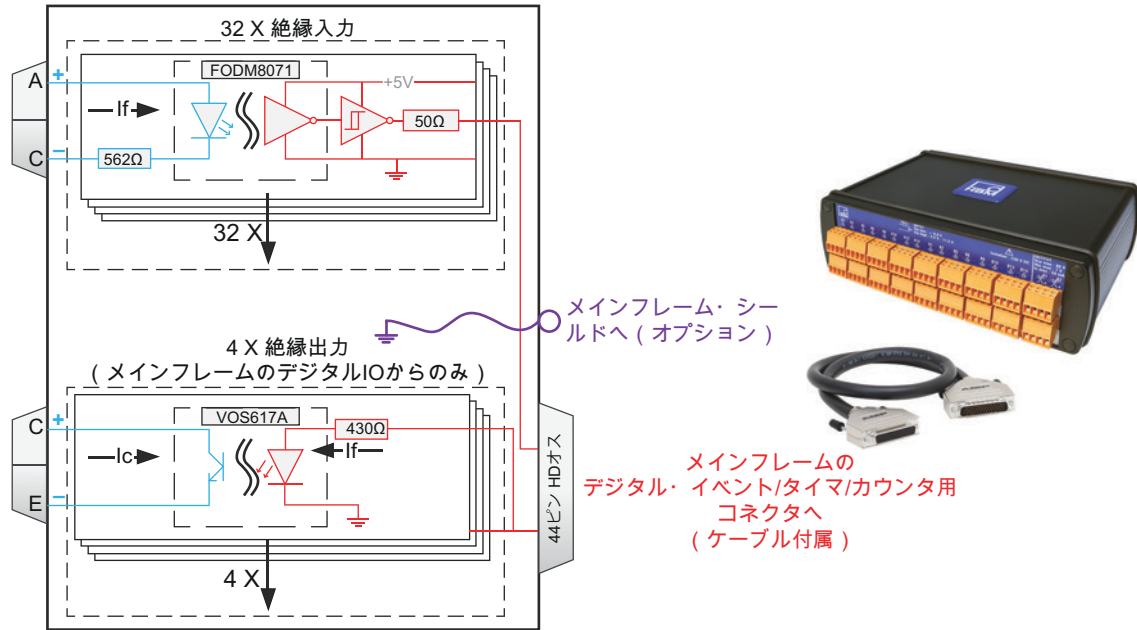
図 1.31: ブロック図と画像
