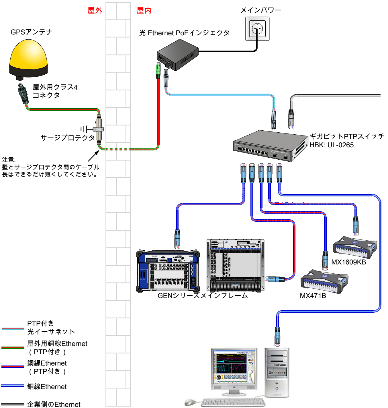
図 1.35: 接続されたメインフレームと QuantumX 用の GPS 設定
