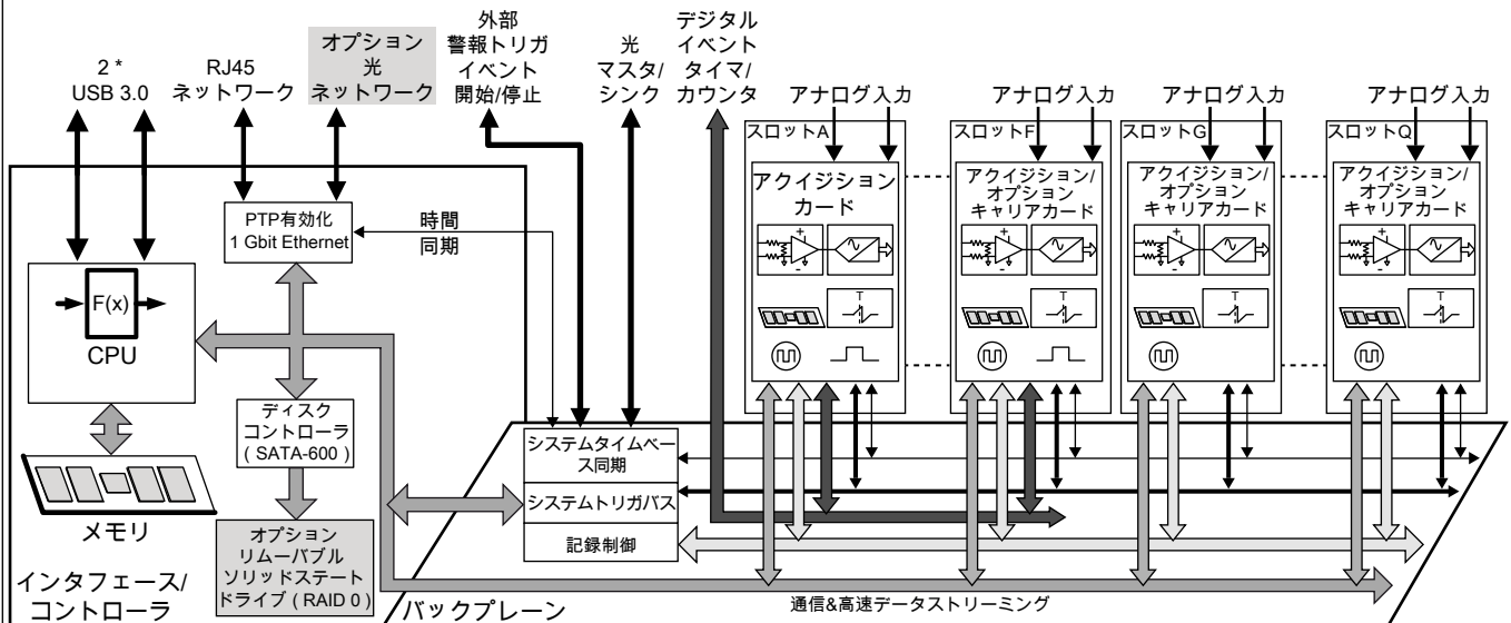
図 1.6: ブロック図
