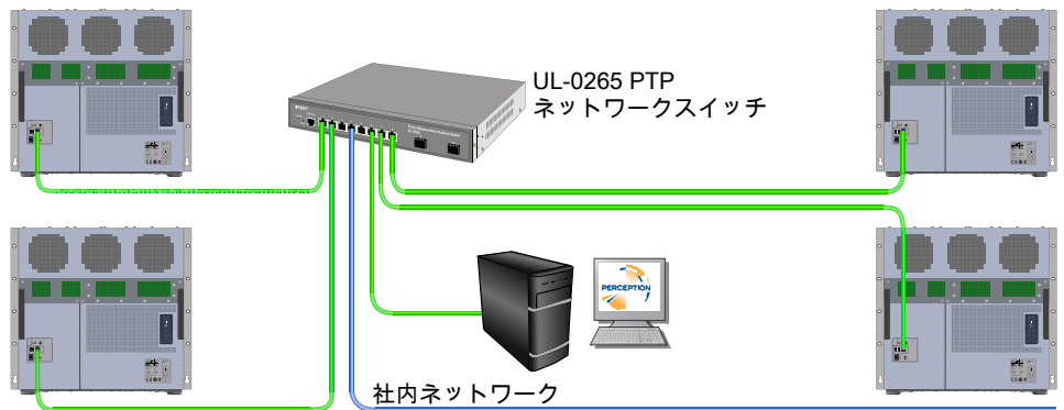
図 1.5: マルチメインフレーム (分散)
