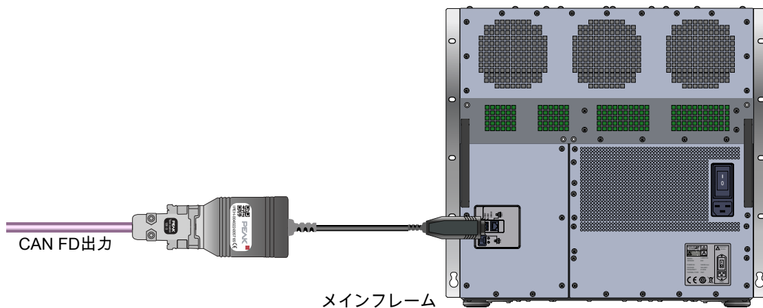
図 1.36: GEN17tA スタンドアロン CAN FD 出力
