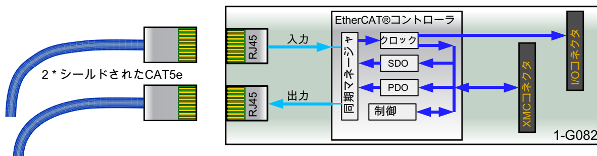
図 1.21: EtherCAT®ボードのブロック図
