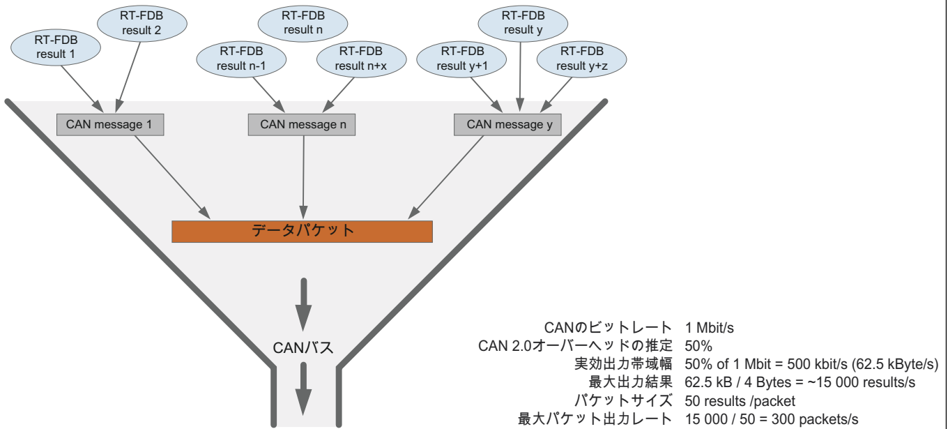
図 1.40: CAN のパケット転送速度の概略計算
