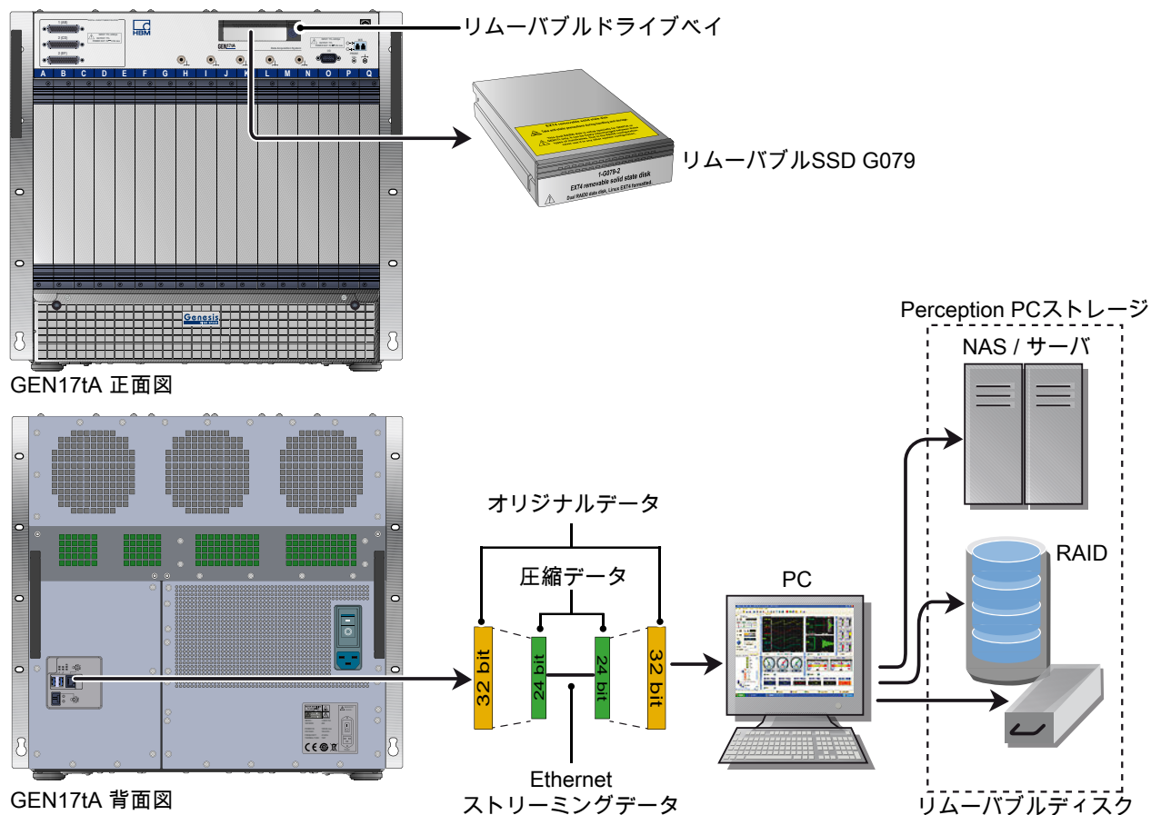
図 1.9: 連続ストリーミングの概要
