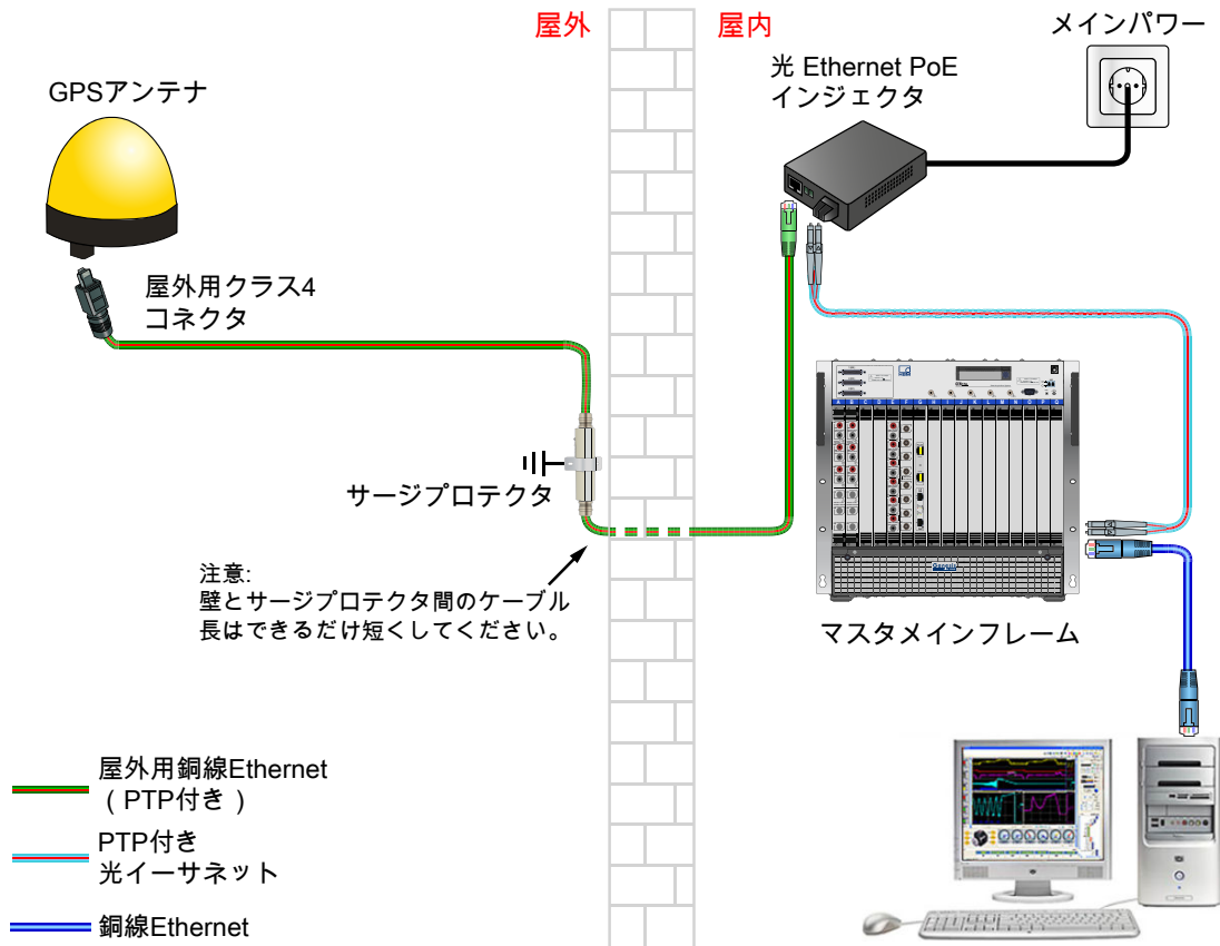
図 1.33: 設定例 GPS 時間同期
