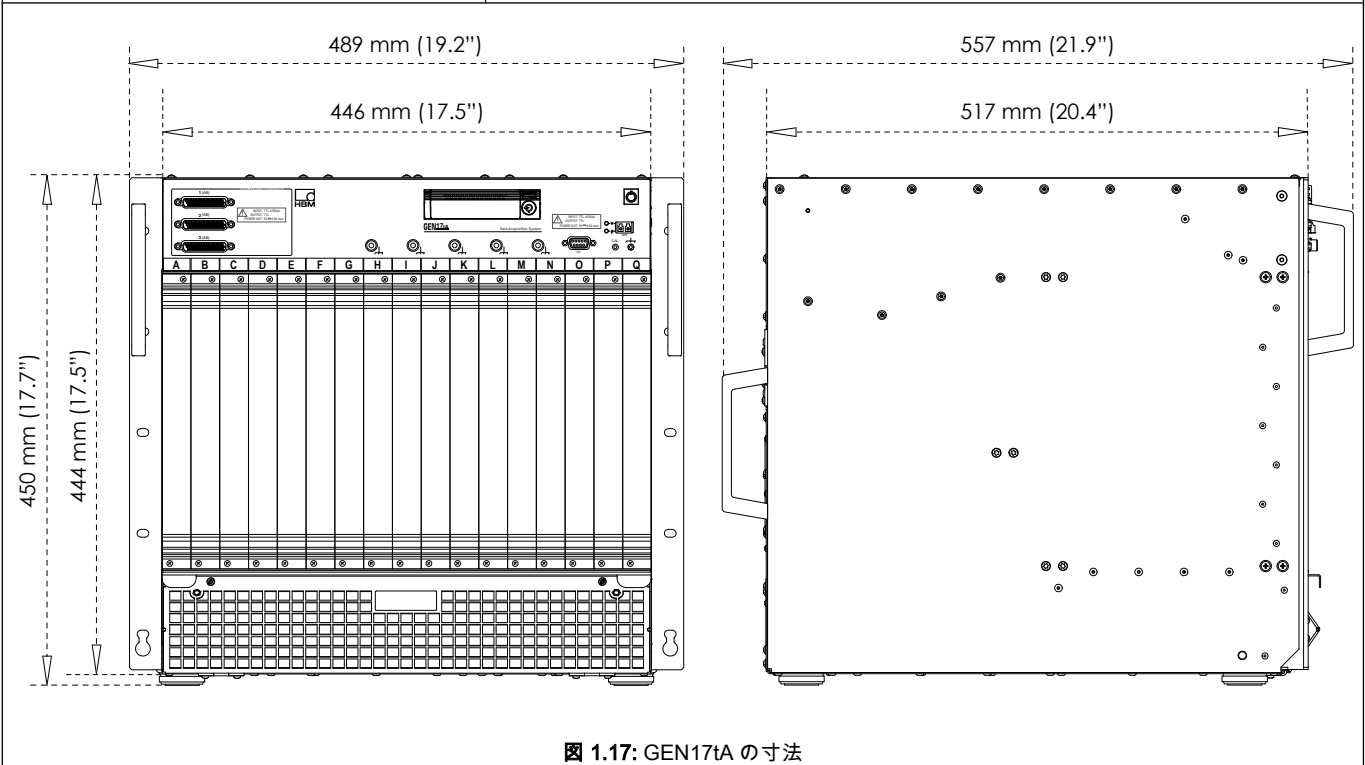
図 1.17: GEN17tA の寸法
