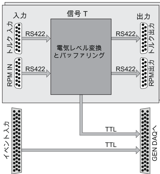
図 1.30: ブロック図と画像
