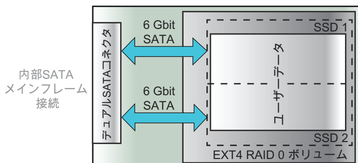
図 1.19: ドライブのブロック図
