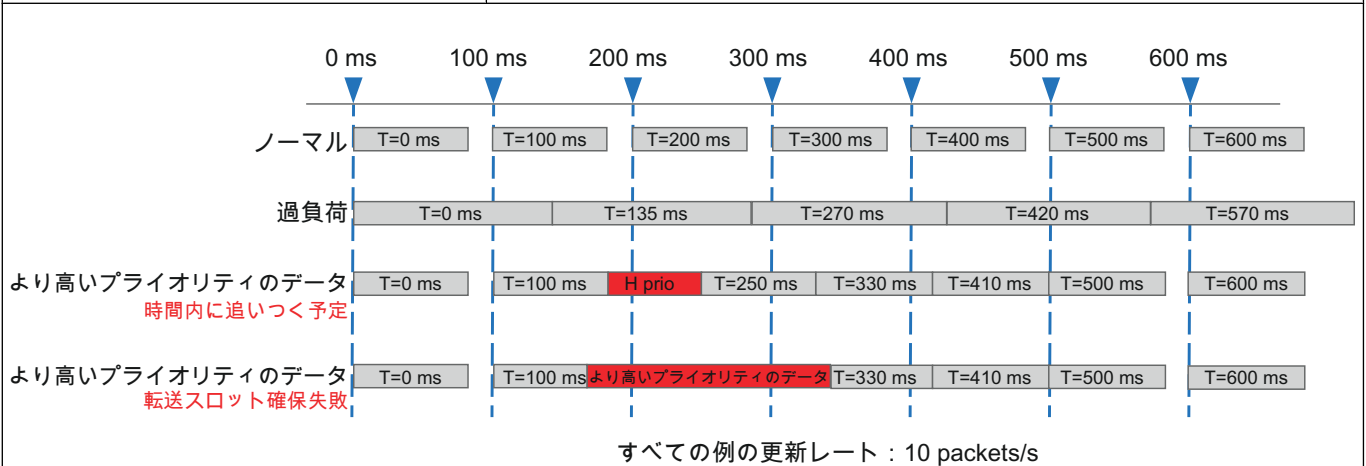
図 1.41: CAN 出力転送レートと待機時間処理
