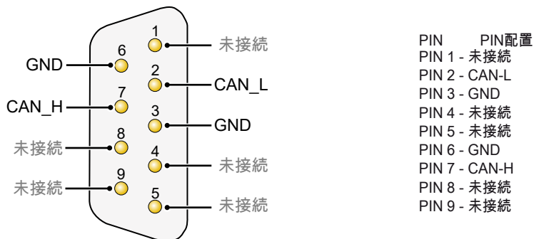
図 1.37: ピン割り当て D-Sub
