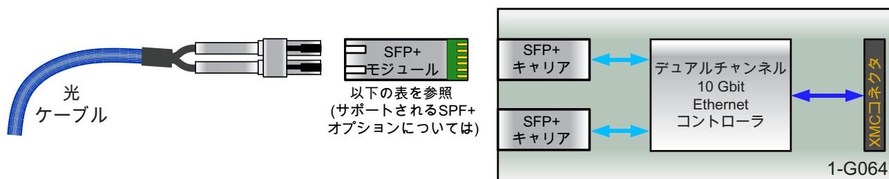
図 1.23: 10Gbit Ethernet ボード、光学式(G081 必須)のブロック図
