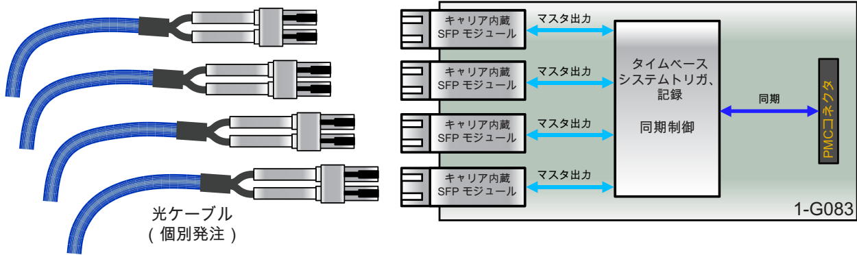
図 1.22: マスタ出力ボードのブロック図 (G081 が必要)
