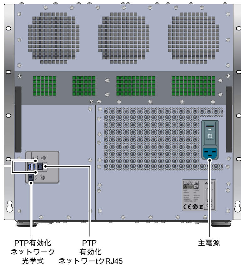
図 1.7: 接続の概要 ( GEN171A 正面図と背面図 )
