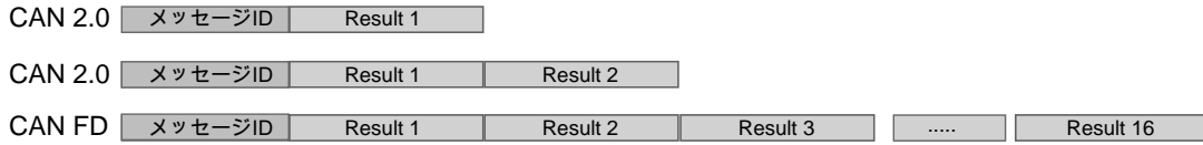
図 1.38: CAN メッセージ設定
