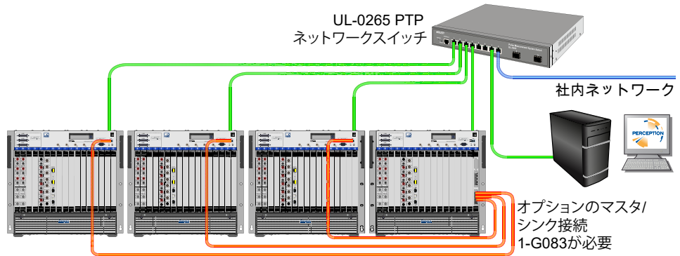
図 1.4: マルチメインフレーム
