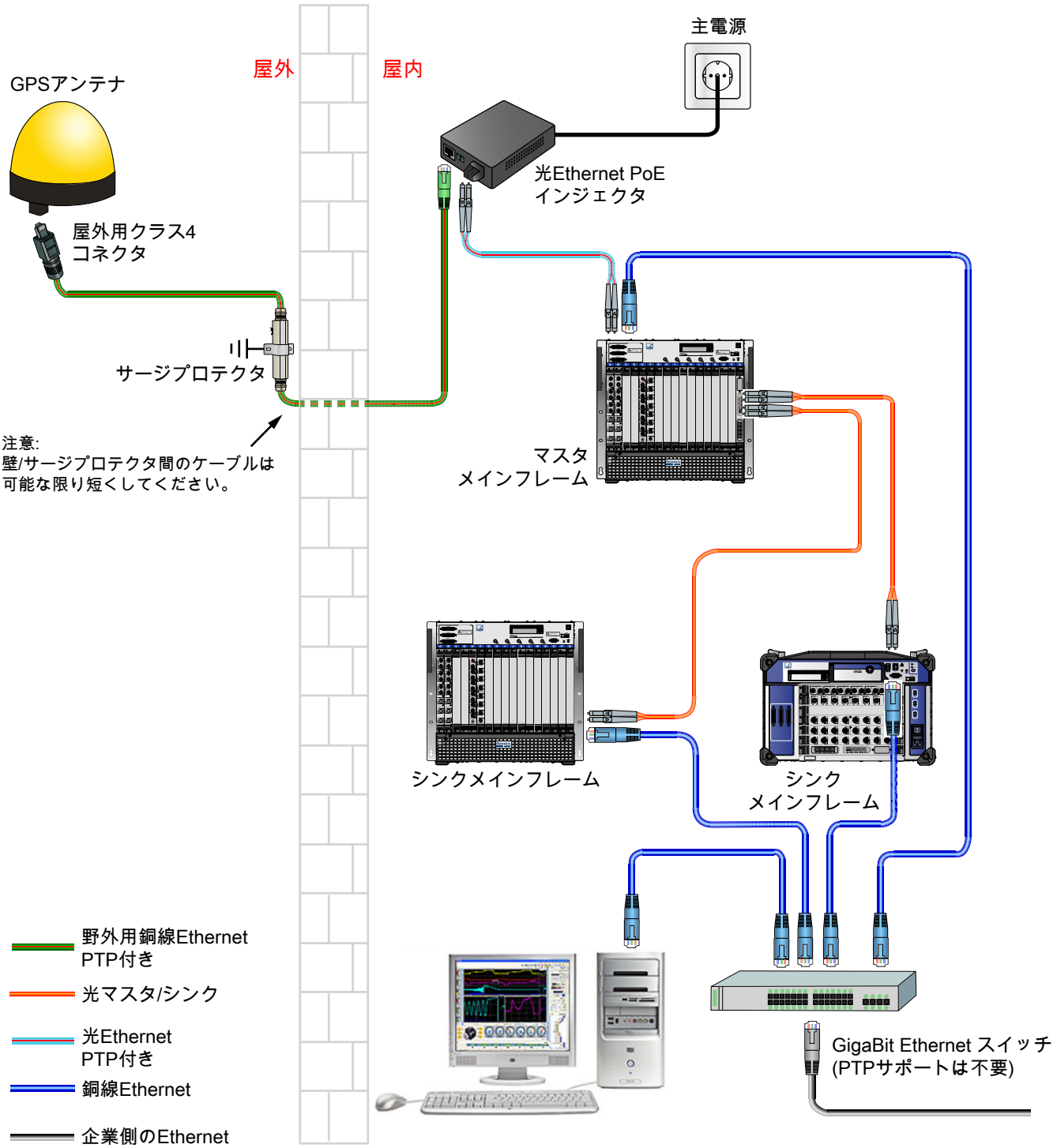
図 1.34: シンク・メインフレームに接続されたマスタ/シンクにメインフレームを接続するための GPS 設定
