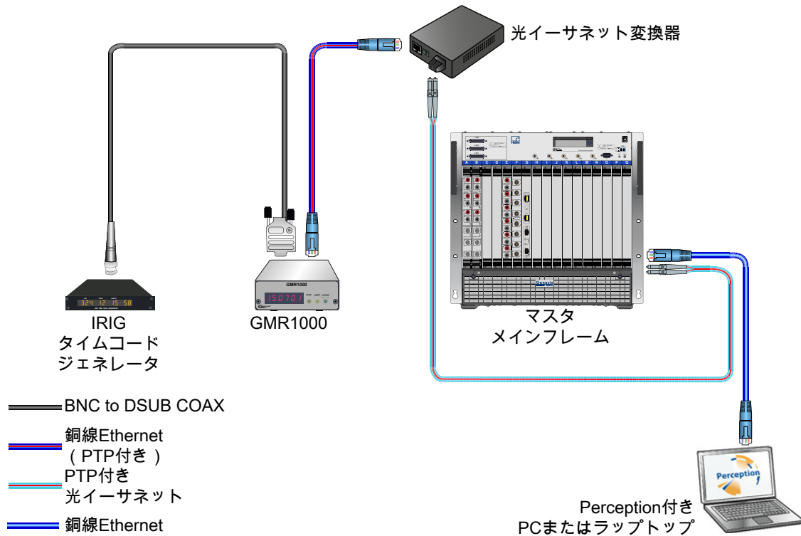
図 1.32: IRIG 時間同期の設定例
