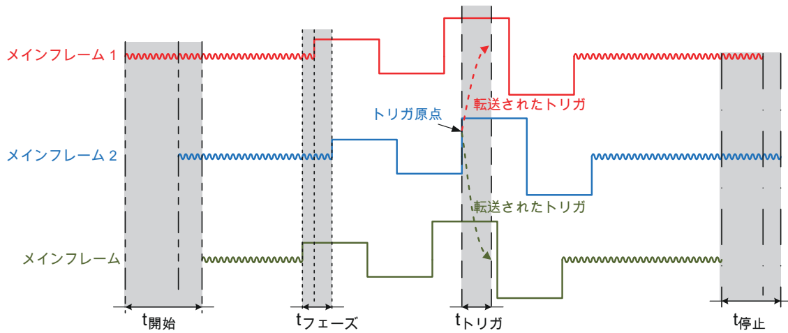
図 1.11: 同期仕様の概要
