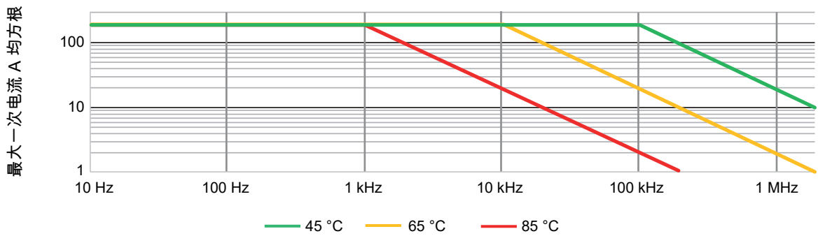
图 2: 频率和环境温度降额
