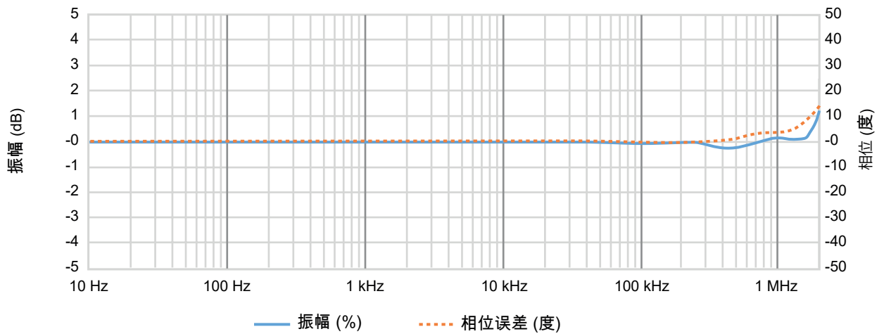
图 3: 频率特征
