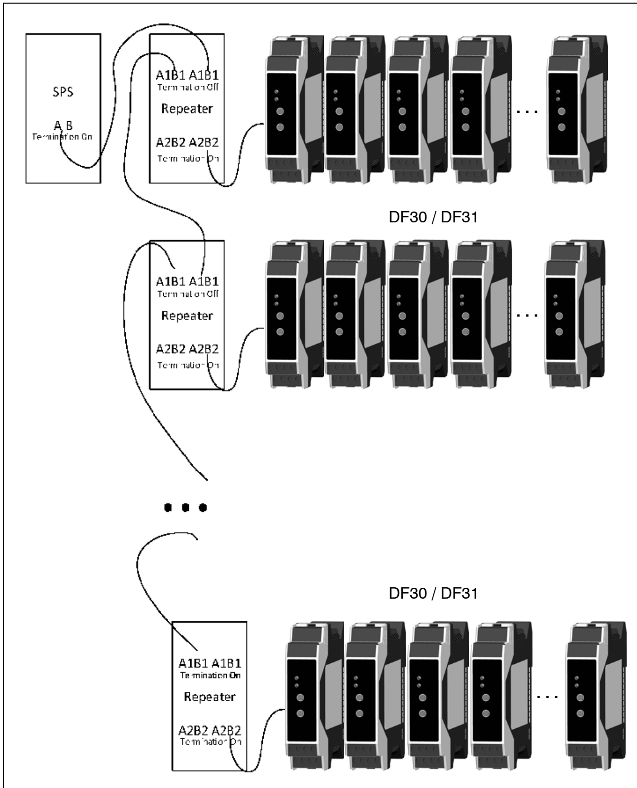
Abb. 4.11: Standard-Repeater für den universellen digiCLIP-Einsatz in einem Profibus-Netz
