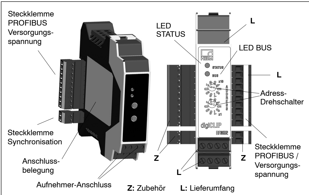
Abb. 2.1: digiCLIP-Modul DF30DP
