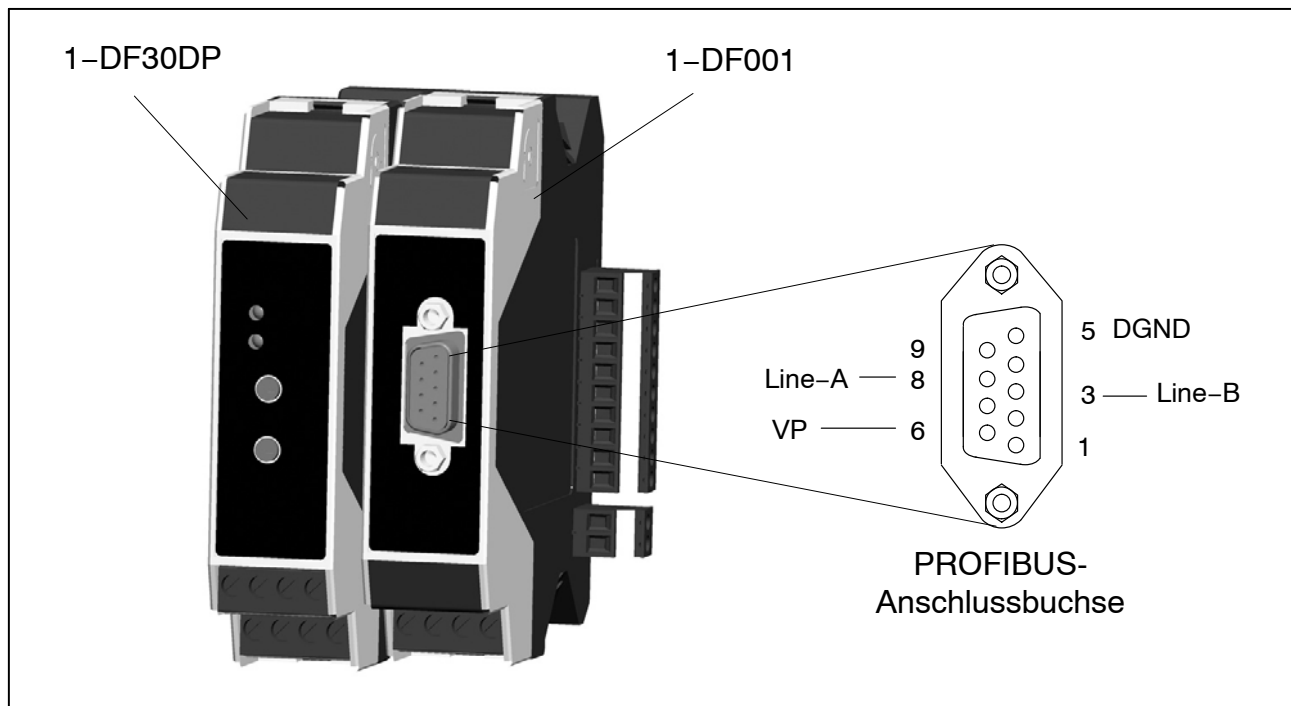
Abb. 4.6: PROFIBUS-Anschlussstecker (9polige D-Sub-Anschlussbuchse)
