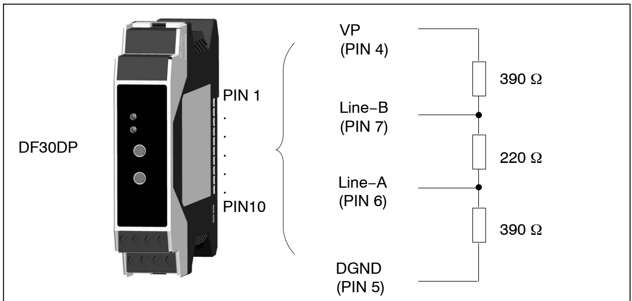
Abb. 4.7: Abschlusswiderstand anschließen, 10polige seitliche Steckerleiste (ohne Modul DF001)
