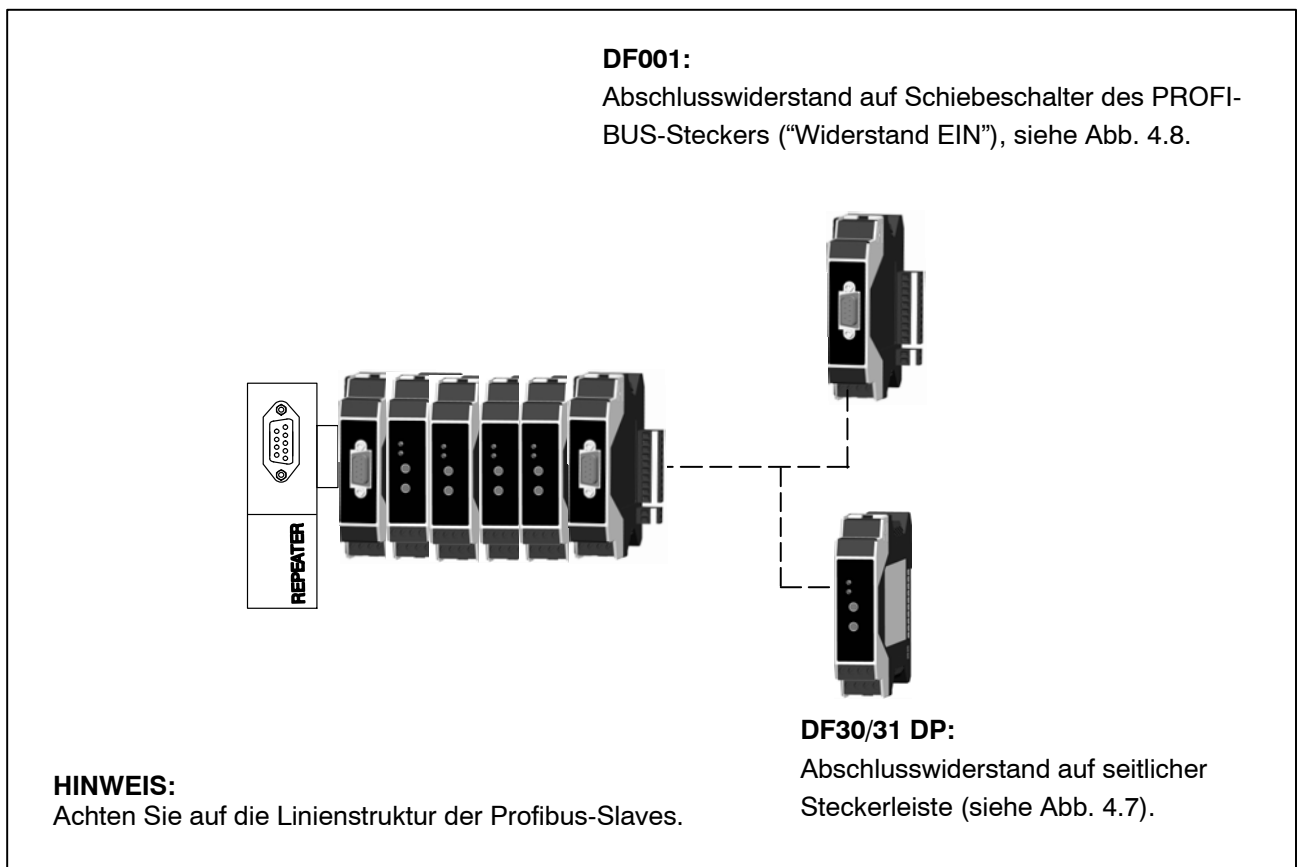
Abb. 4.9: digiCLIP-Gruppe am Ende des Profibus-Segmentes
