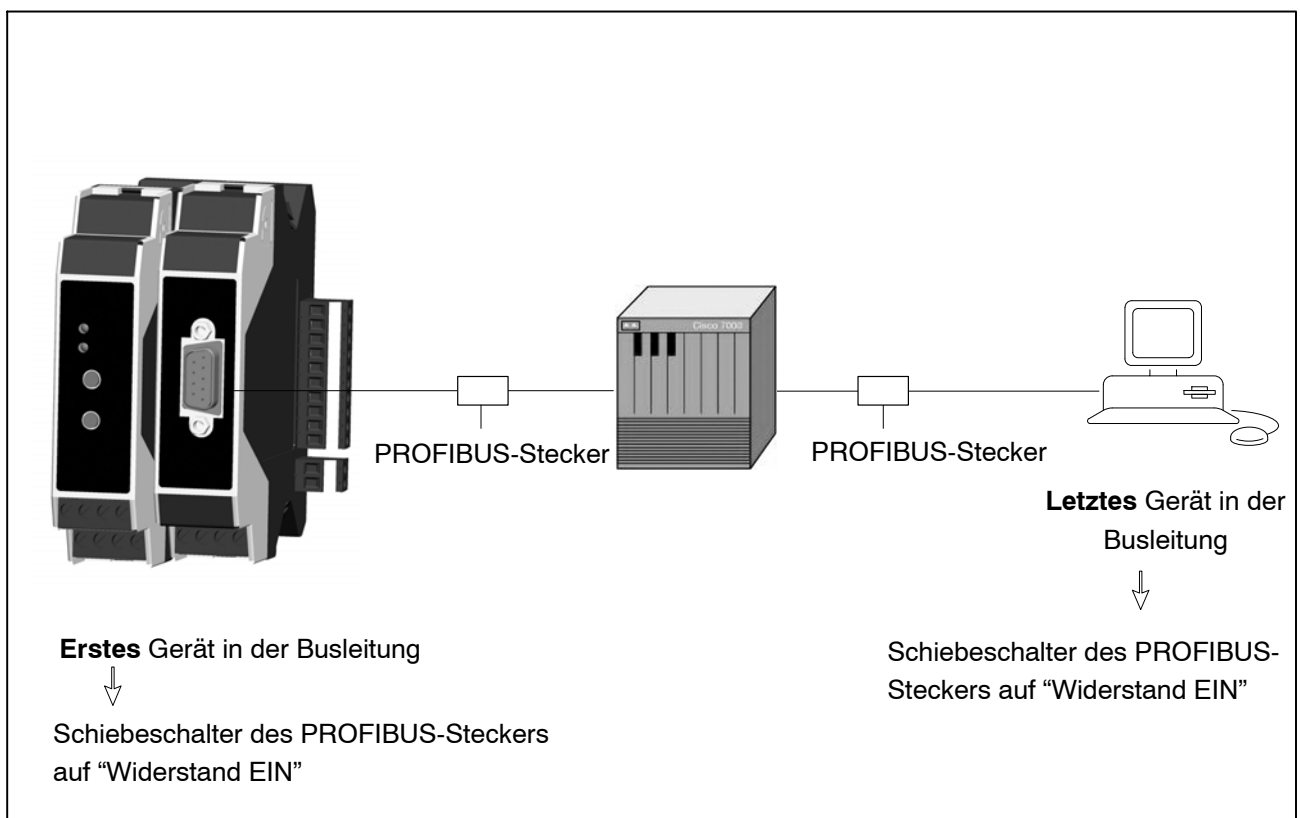
Abb. 4.8: PROFIBUS-Betrieb
