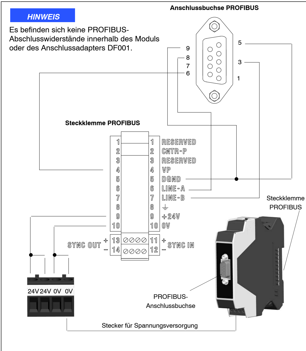
Abb. 4.1: DF30DP :Pinbelegung des Adaptermoduls DF001
