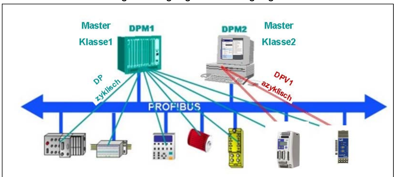
Abb. 7.1: Aufbau und Konfiguration eines Profibus-DP-Systems
