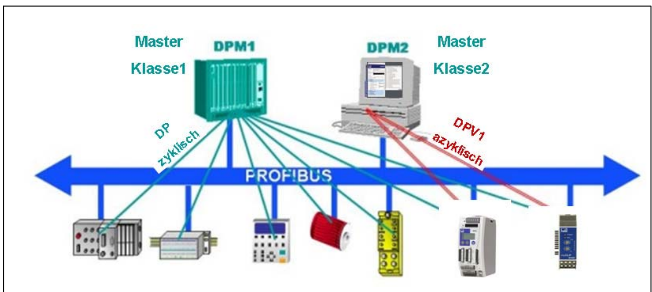
Abb. 7.4: PROFIBUS–Netzwerk mit zyklischem und azyklischen Datentransfer
