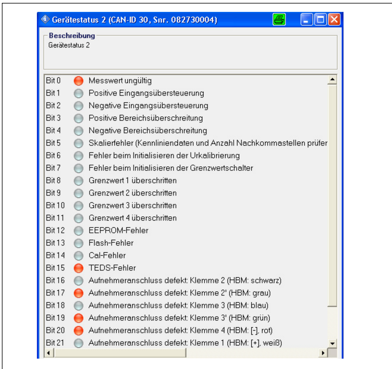
Abb 6.1: Assistent: Gerätestatus
