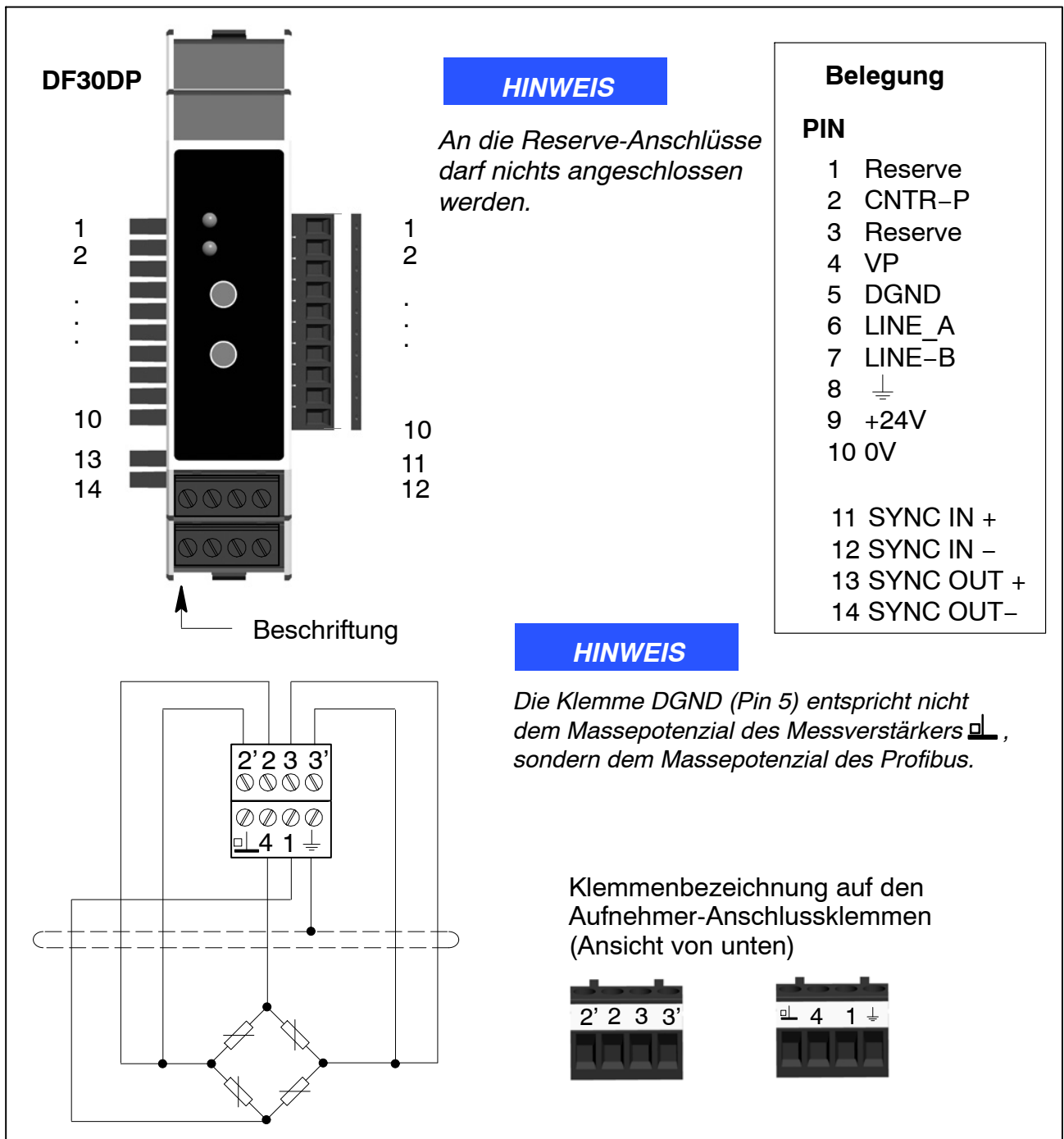
Abb. 4.2: DF30DP: Steckklemmenbelegung (einfach geschirmtes Kabel)
