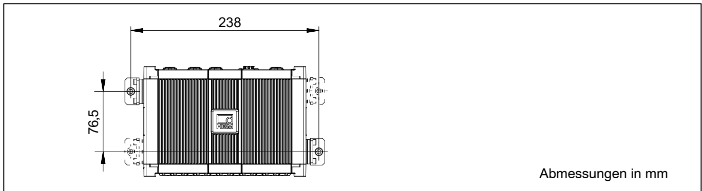
Abb. 1: Montage-Abmessungen CASEMOUNT
