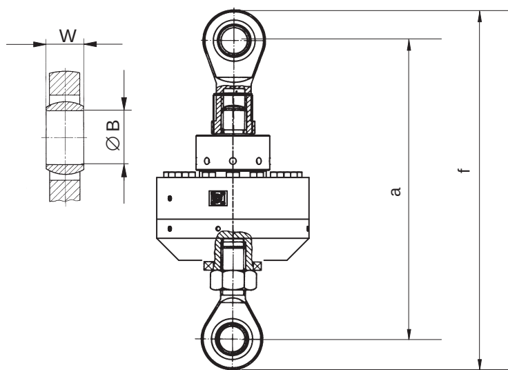
Anneaux à rotule
