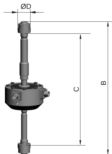
Introduction d'effort en traction ZKM selon ISO 376
