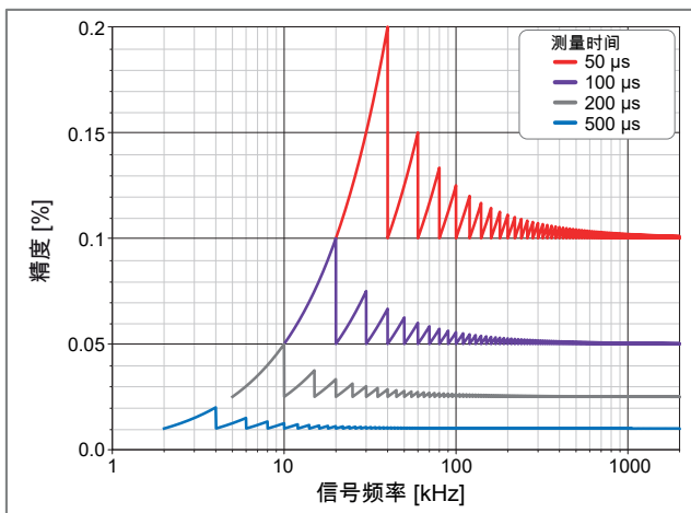
图 26: 最大频率不准确度
