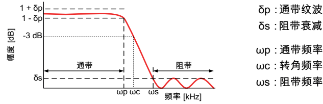
图 15: 数字巴特沃斯 IIR 滤波器
