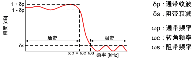
图 17: 数字椭圆 IIR 滤波器
