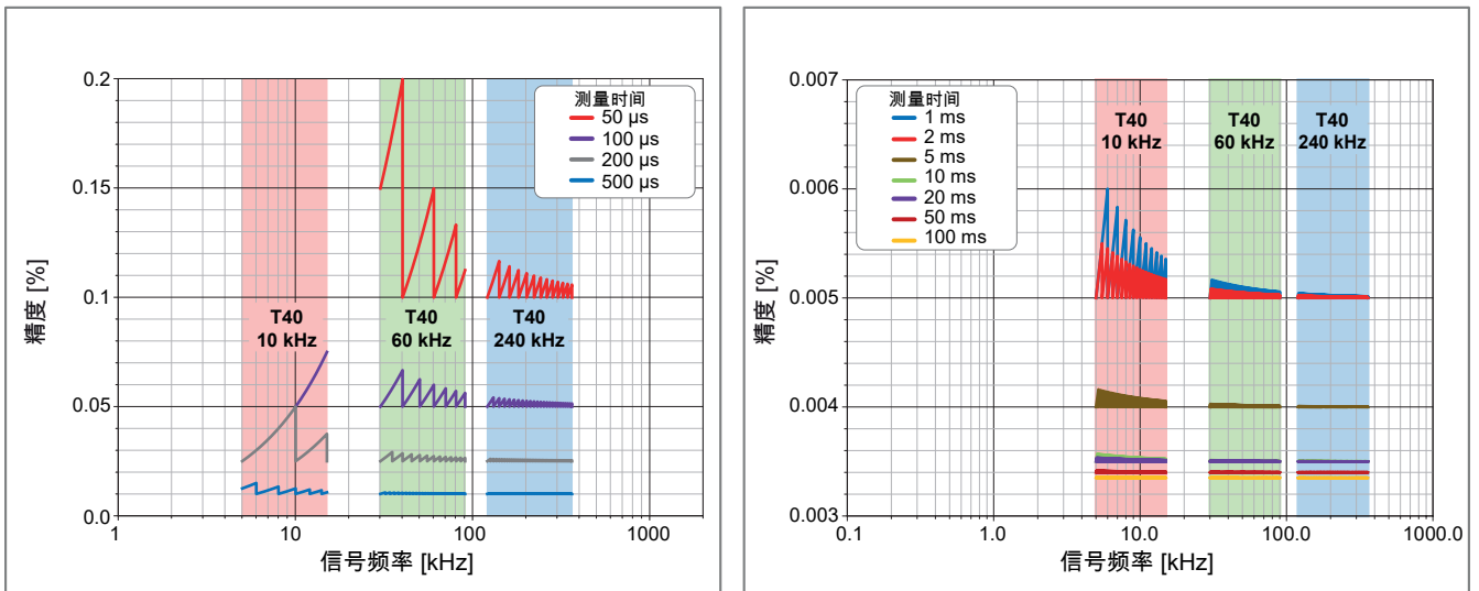
图 27: 扭矩工作范围相对于偏差和测量时间之间的关系
