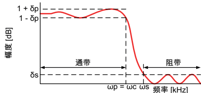
图 19: 数字椭圆 IIR 滤波器
