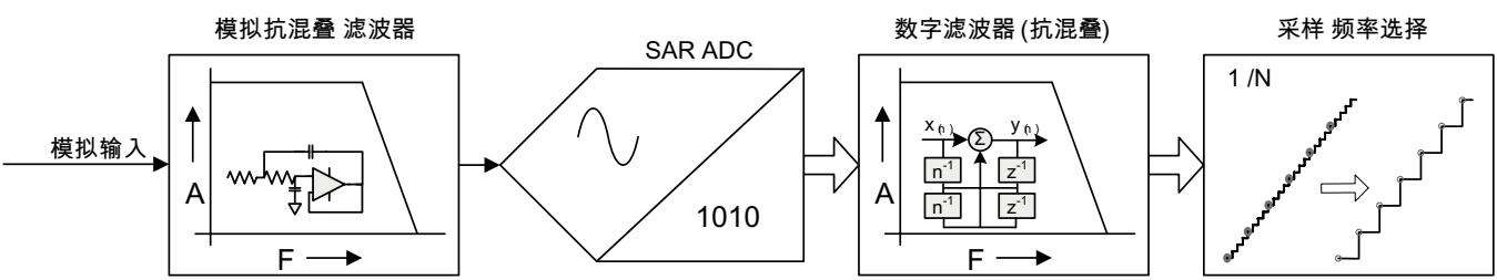
图 7: 混合模拟和数字抗混叠滤波器框图
