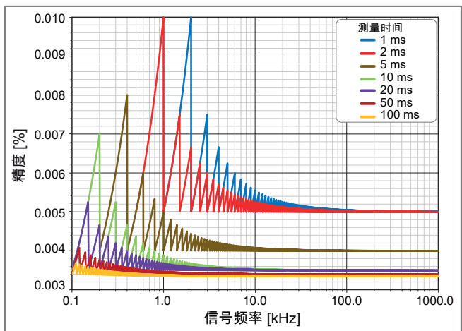
图 26: 最大频率不准确度
