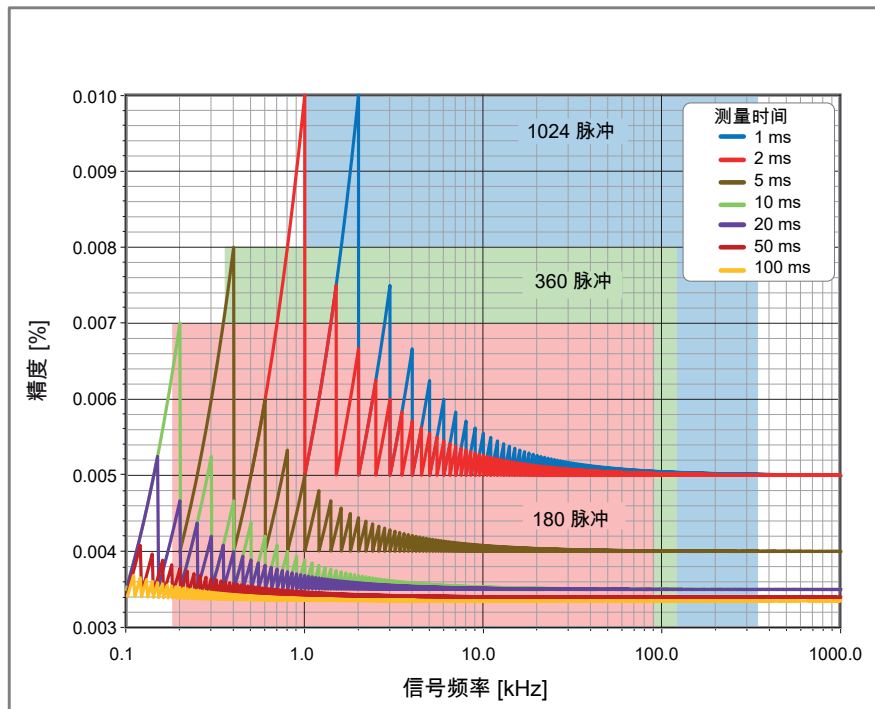
图 28: RPM 传感器工作范围相对于误差和测量时间之间的关系
