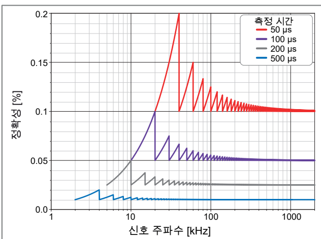
그림 26: 최대 주파수 부정확
