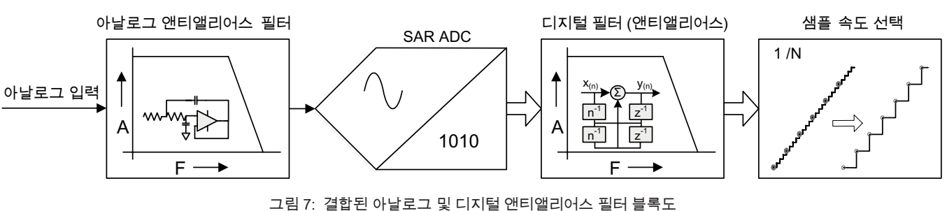
그림 7: 결합된 아날로그 및 디지털 앤티앨리어스 필터 블록도
