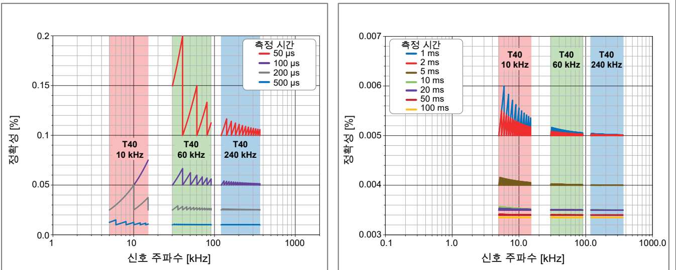
그림 27: 토크 작동 범위 대 부정확 및 측정 시간
