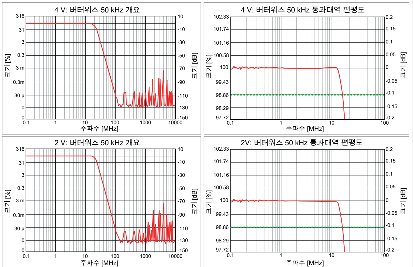
그림 16: 대표적 버터워스 IIR 예시(GN816)
