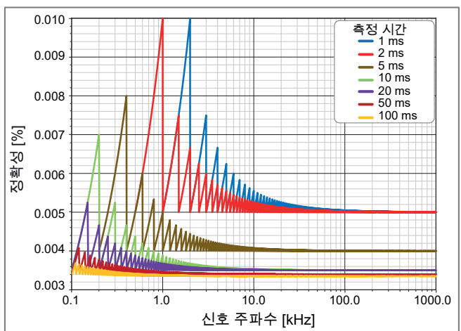
그림 26: 최대 주파수 부정확
