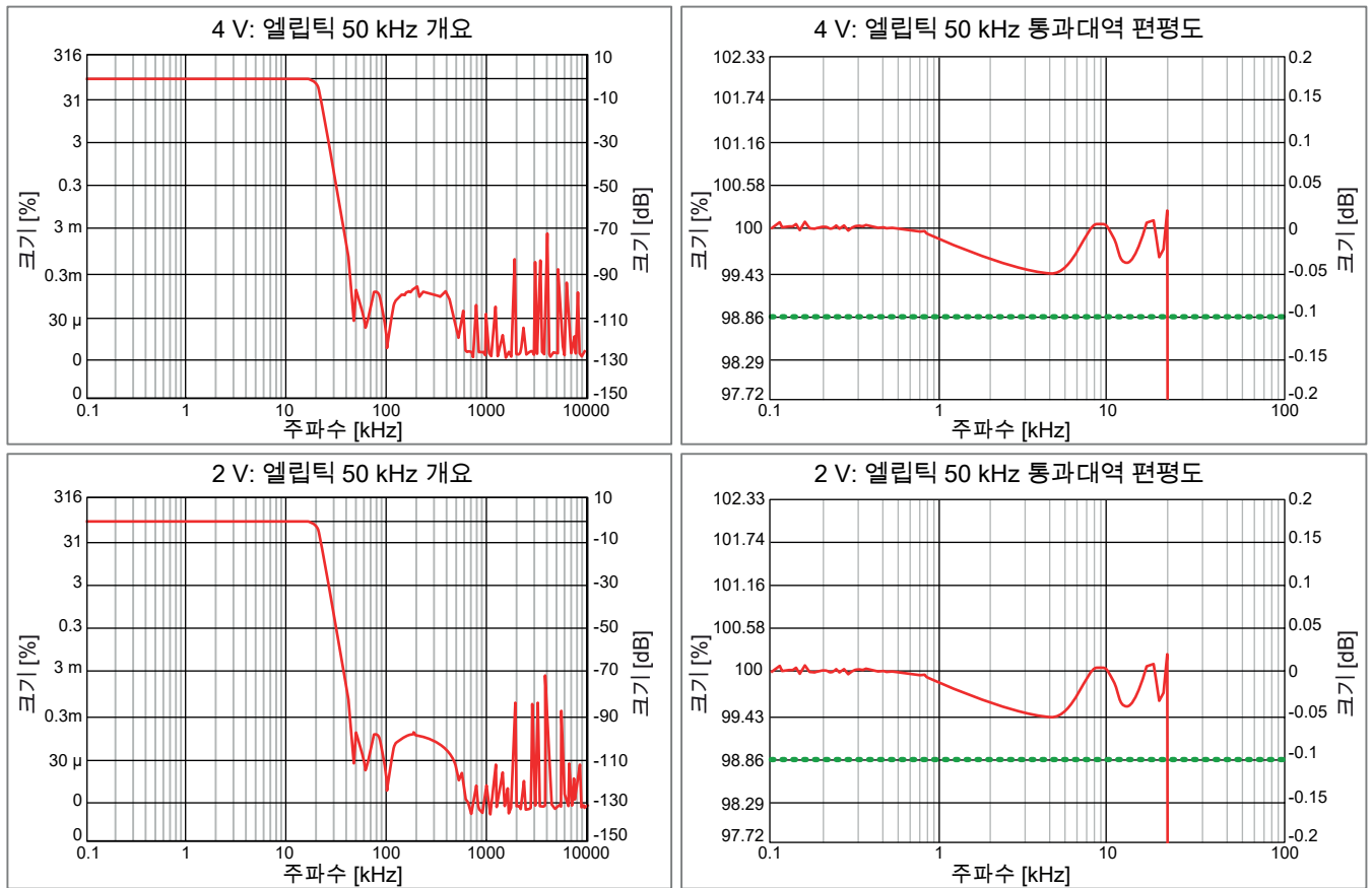
그림 20: 대표적 엘리틱 IIR 예시(GN816)
