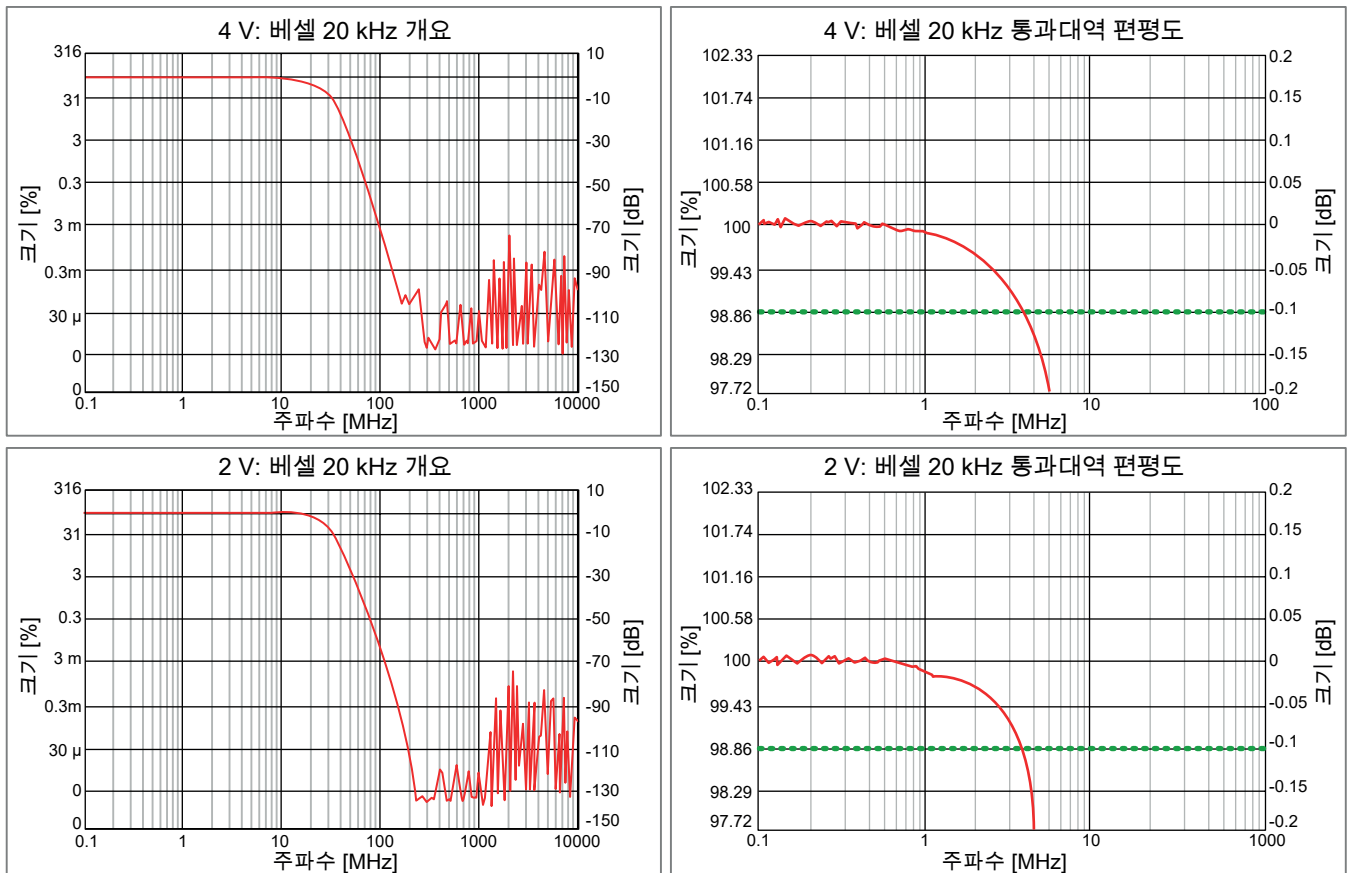
그림 12: 대표적 베셀 IIR 예시(GN816)
