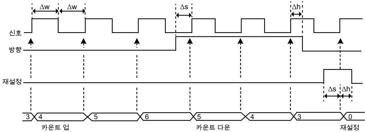
그림 23: 단방향 및 양방향 타이밍
