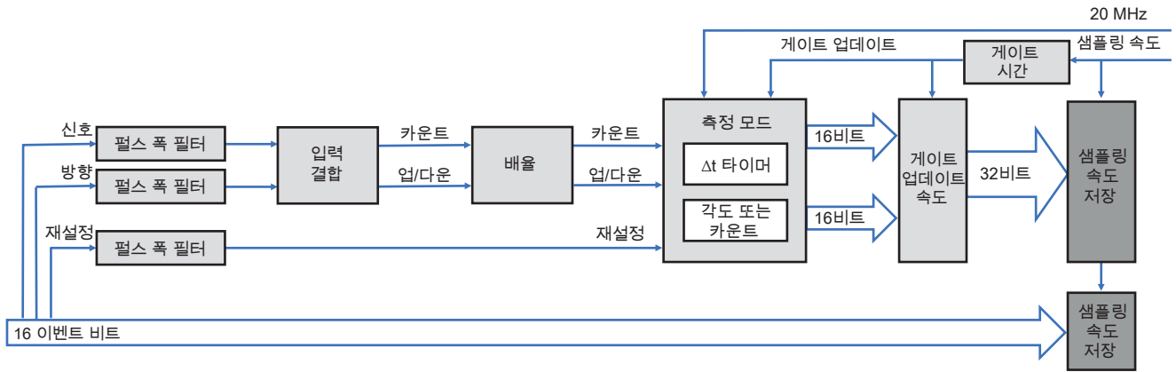
그림 22: 타이머/카운터 블록도
