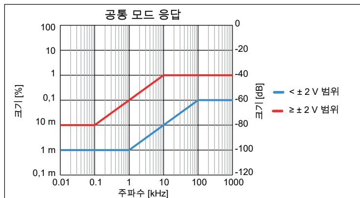
그림 5: 대표적 공통 모드 응답
