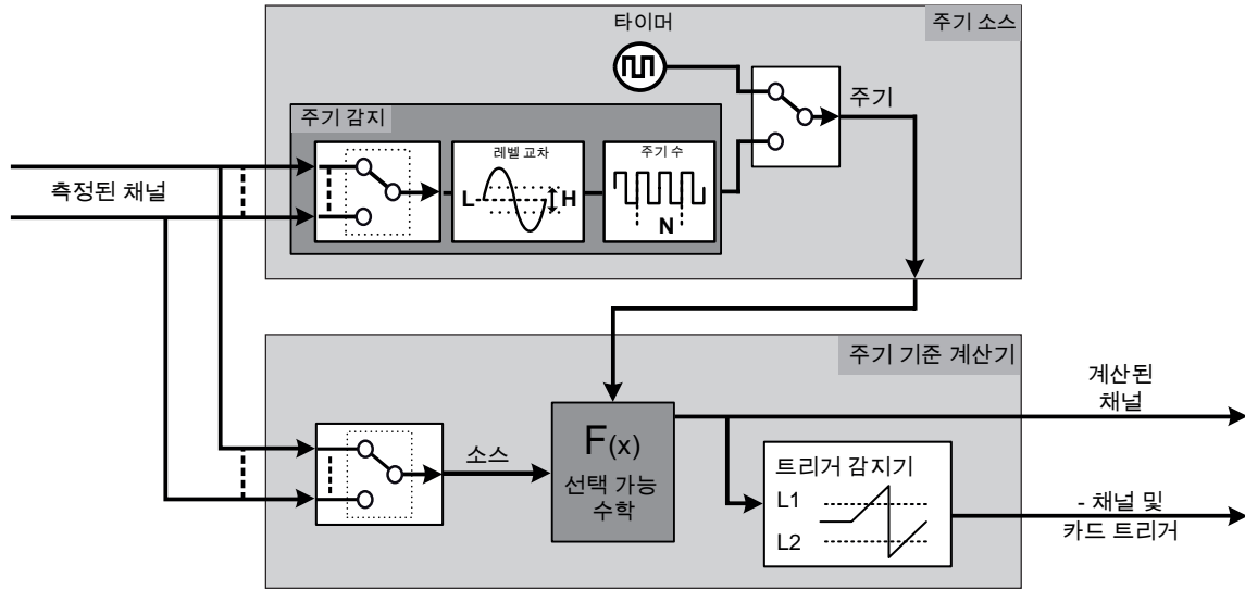
그림 30: 실시간 주기 기준 계산기
