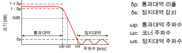
그림 13: 디지털 버터워스 IIR 필터
