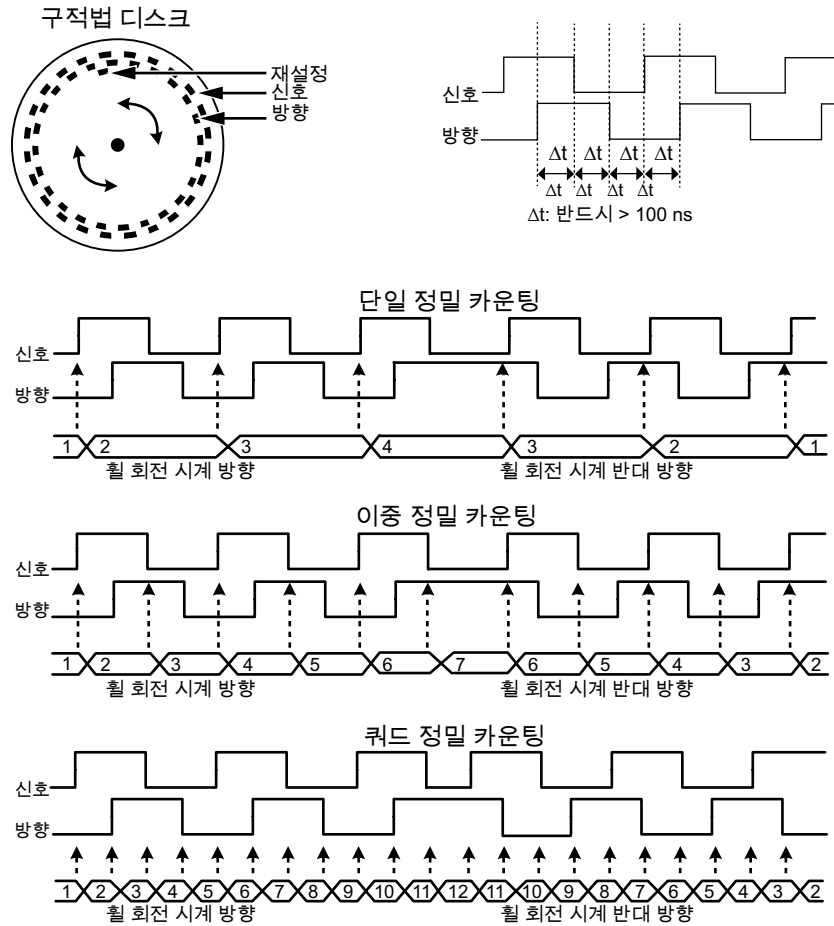
그림 24: 양방향 구적법(quadrature) 카운트 모드
