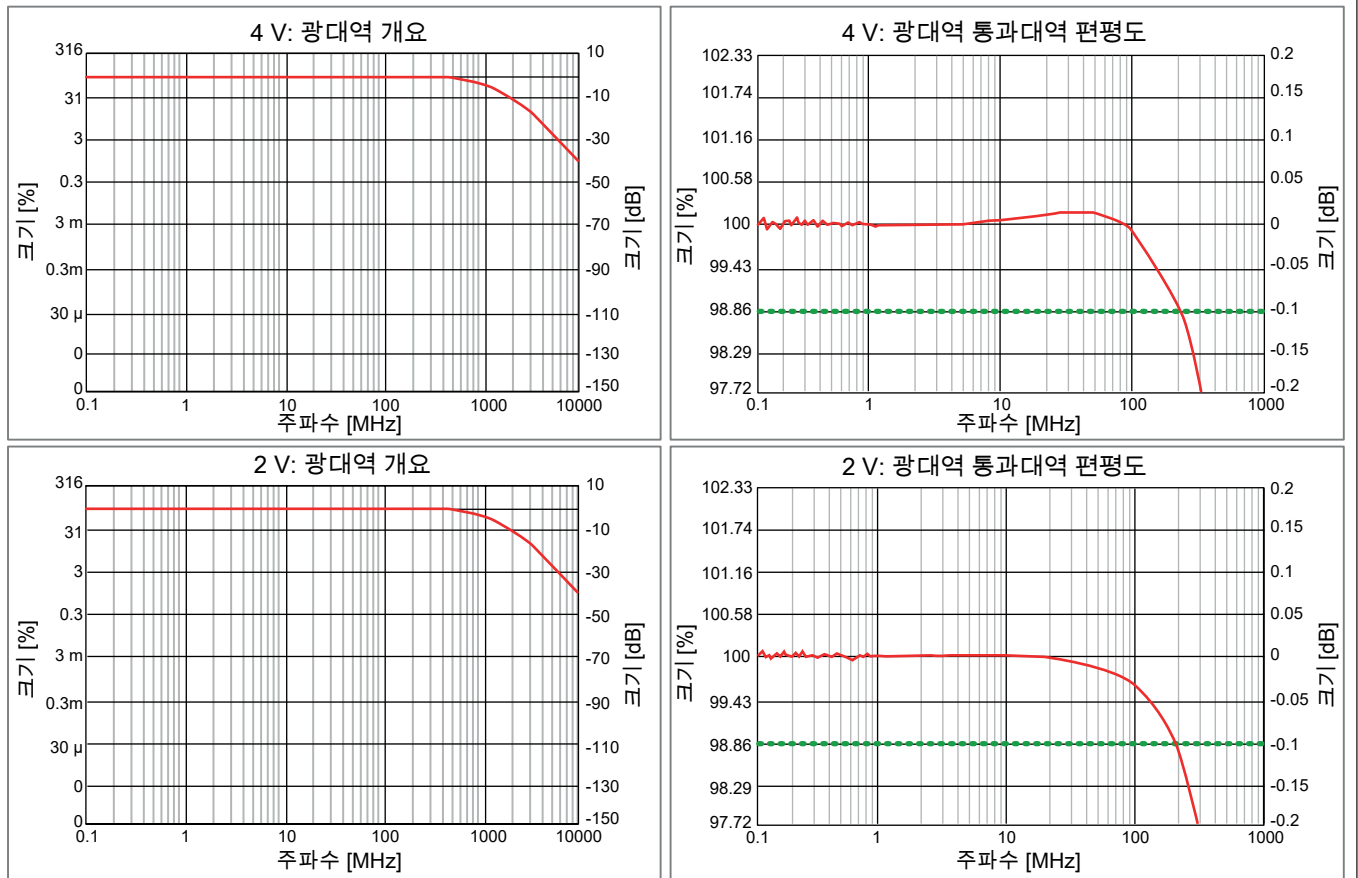
그림 8: 대표적 광대역 예시
