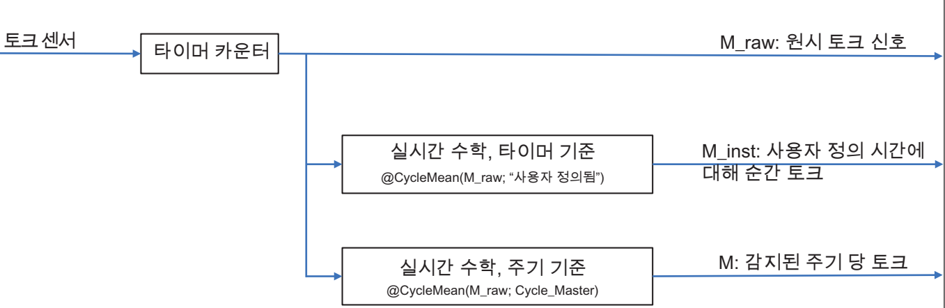
그림 29: 동시 동적 및 정확한 토크 계산
