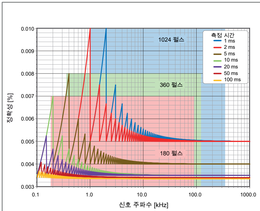
그림 28: RPM 센서 작동 범위 대 부정확 및 측정 시간
