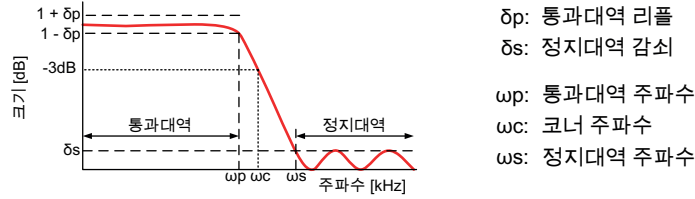
그림 15: 디지털 버터워스 IIR 필터
