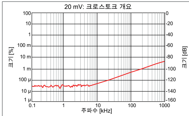
그림 21: 대표적 채널 대 채널 크로스토크
