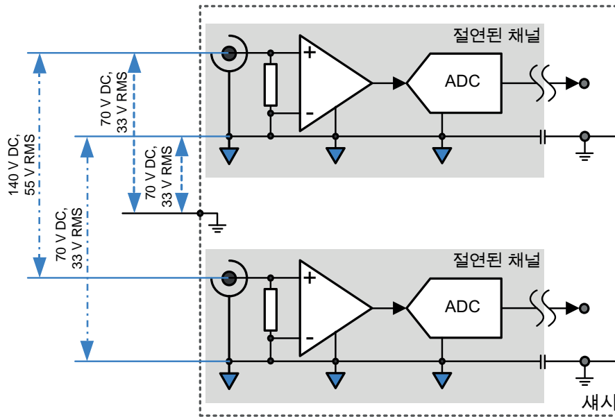
그림 6: 절연 회로도
