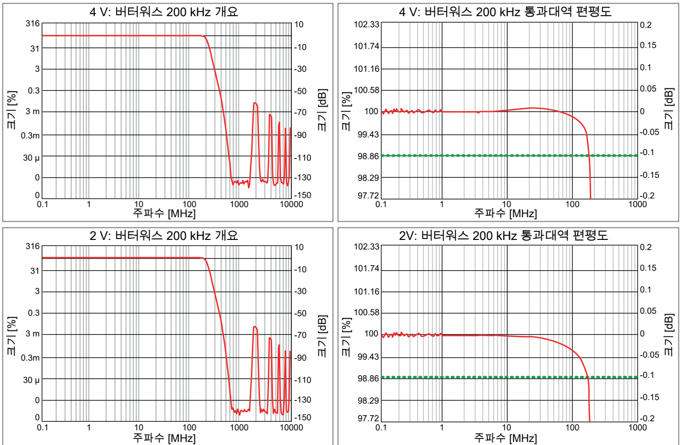
그림 14: 대표적 버터워스 IIR 예시(GN815)
