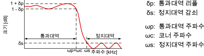
그림 17: 디지털 엘리틱 IIR 필터
