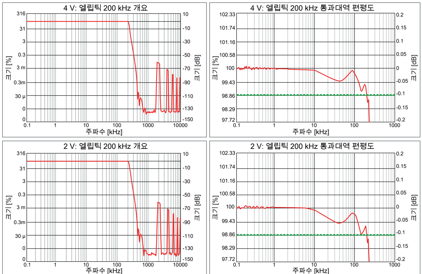
그림 18: 대표적 엘리틱 IIR 예시(GN815)
