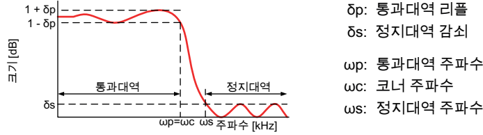
그림 19: 디지털 엘리틱 IIR 필터
