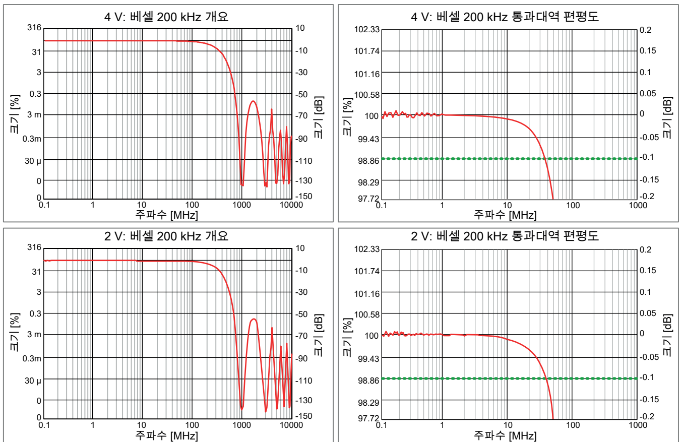
그림 10: 대표적 베셀 IIR 예시(GN815)
