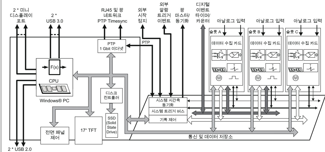
그림 1.6: 블록도
