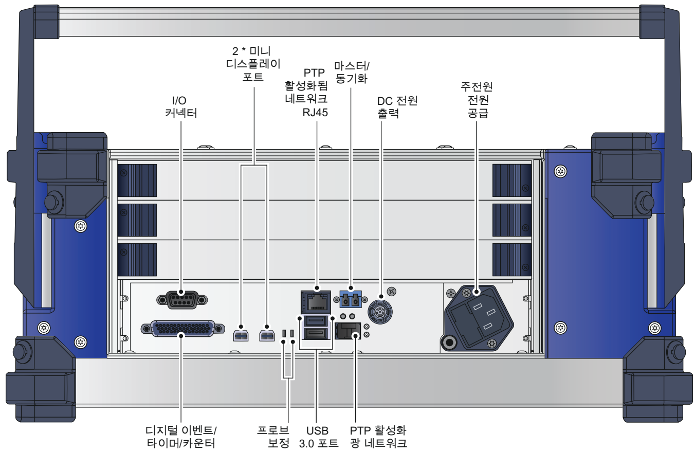
그림 1.7: 연결 개요
