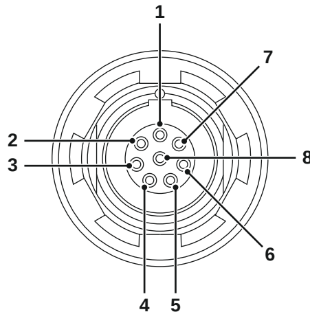
그림 1.17: 커넥터 전원 출력
