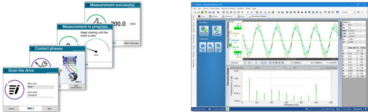
그림 1.39: Perception CSI 예시 BackEMF (왼쪽) 조화 분석 (오른쪽)
