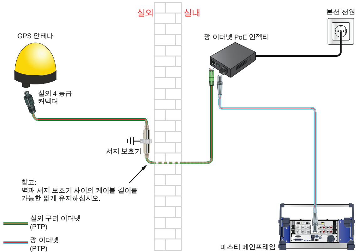
그림 1.32: 예제 설정 GPS 시간 동기화
