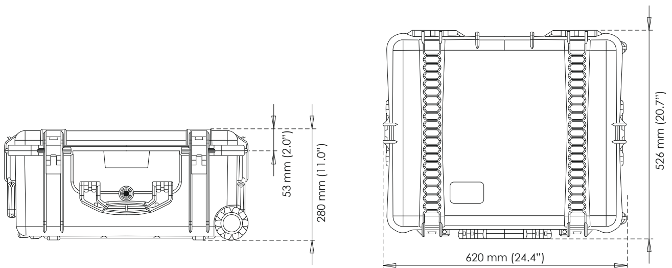
그림 1.35: 재활용 가능 하드커버 배송 케이스(휠 및 운송 핸들 포함)
