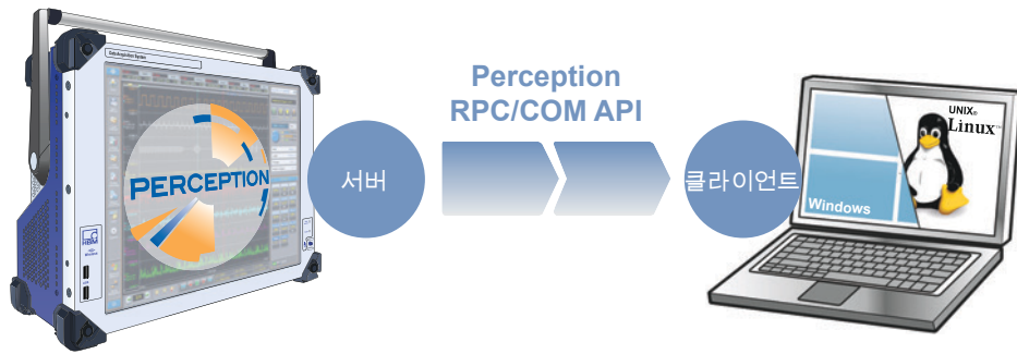
그림 1.37: 기능도 DCE/RPC
