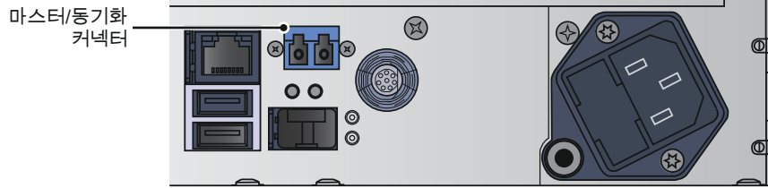
그림 1.11: 마스터/동기화 커넥터
