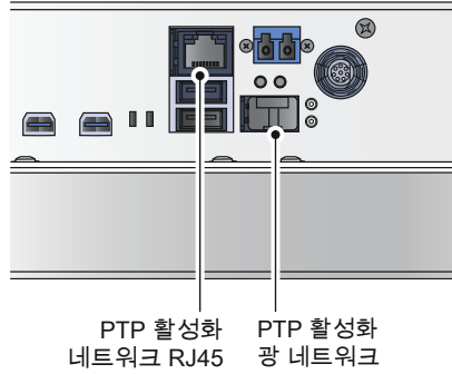
그림 1.8: 전기 및 광 1 Gbit 네트워크 인터페이스
