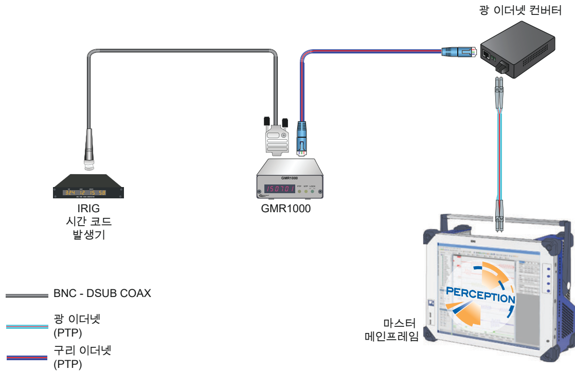
그림 1.31: 예제 설정 IRIG 시간 동기화
