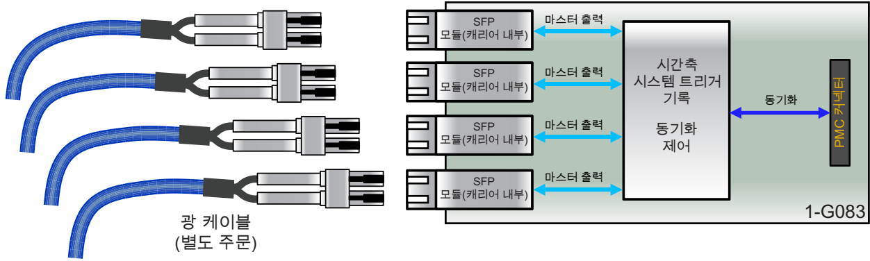
그림 1.21: 블록도 마스터 출력 카드 (G081 필요)
