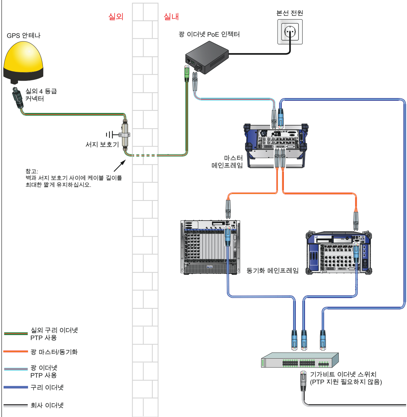
그림 1.33: 마스터/동기화 연결 동기화 메인프레임과 테더링된 메인프레임용 GPS 설정
