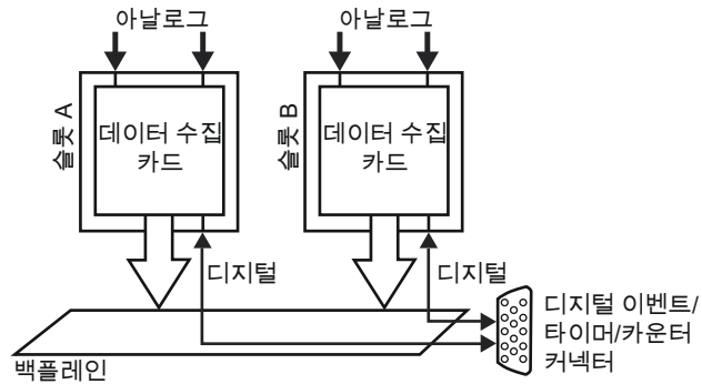
그림 1.14: 디지털 이벤트/타이머/카운터 블록도
