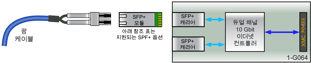
그림 1.22: 블록도 10Gbit 이더넷 카드, 광 (G081 필요)
