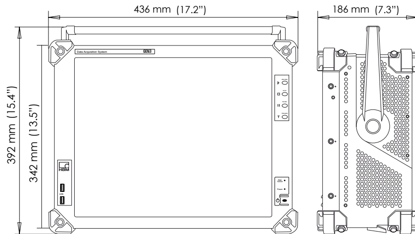
그림 1.18: GEN3iA 치수
