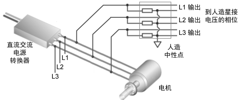
图 1.15: 人造星型连接适配器的一般用途
