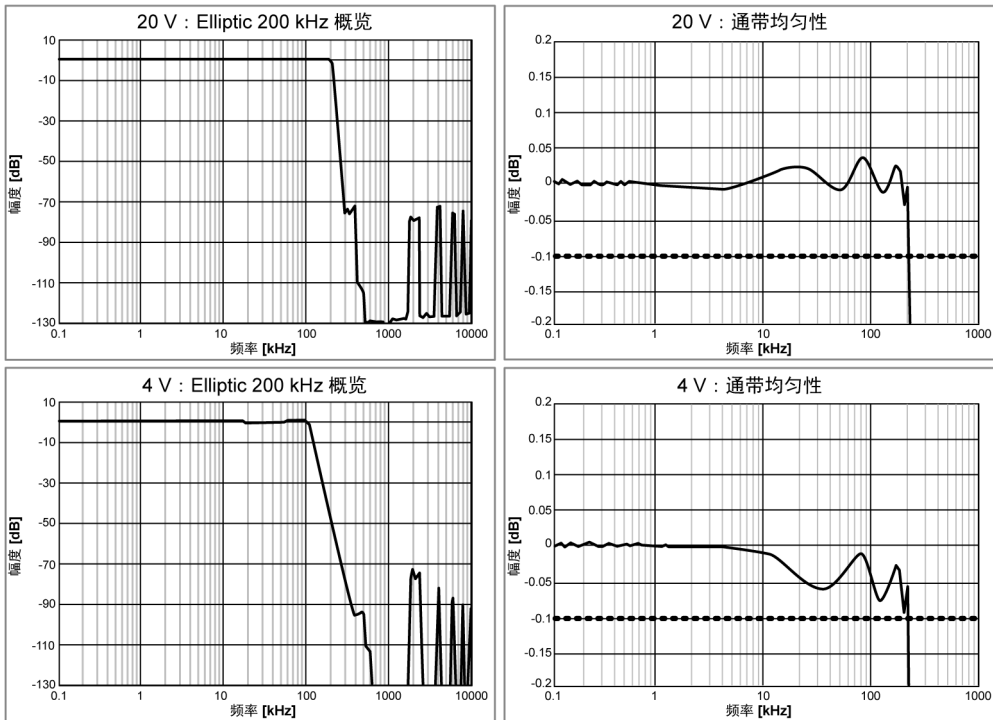
图 1.10: 典型 Elliptic IIR 200 kHz 概览和通带均匀性
