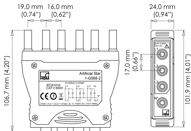
图 1.17: 人造星型连接适配器
