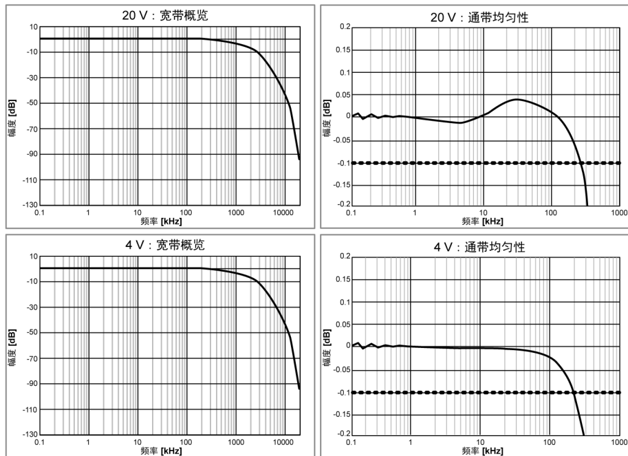
图 1.4: 典型宽带概览和通带均匀性
