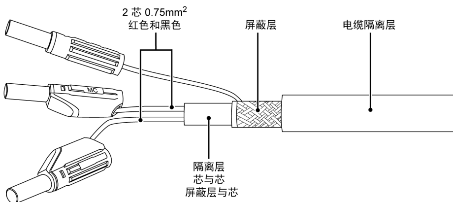
图 1.13: 屏蔽电缆设置
