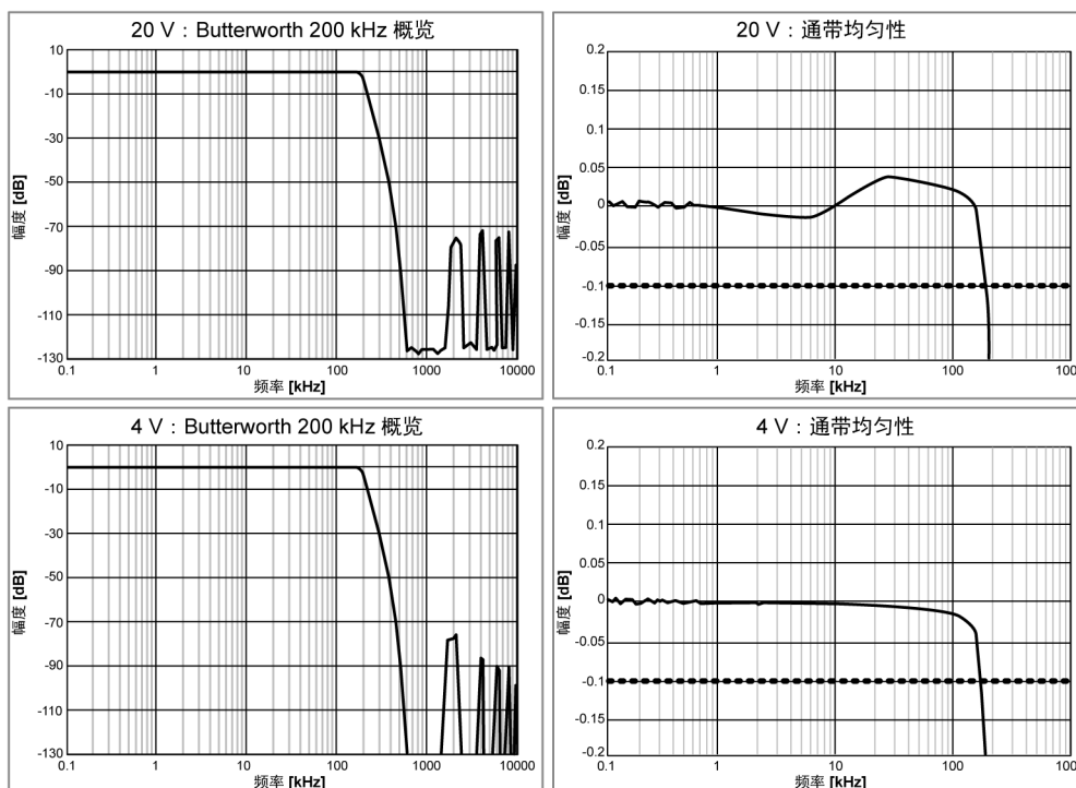
图 1.8: 典型 Butterworth IIR 200 kHz 概览和通带均匀性
