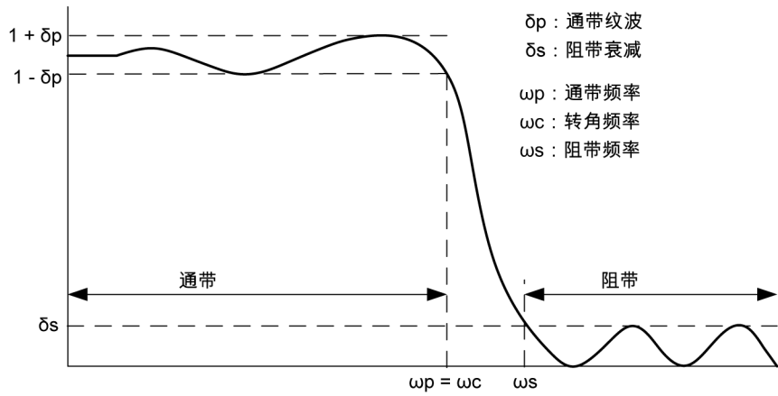
图 1.9: 数字 Elliptic IIR 滤波器
