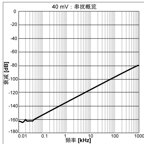
图 1.11: 典型通道到通道串扰
