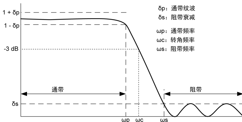
图 1.7: 数字 Butterworth IIR 滤波器
