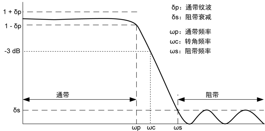
图 1.5: 数字 Bessel IIR 滤波器
