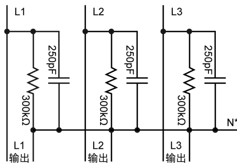
图 1.16: 电气图表
