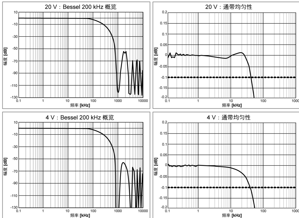
图 1.6: 典型 Bessel IIR 200 kHz 概览和通带均匀性
