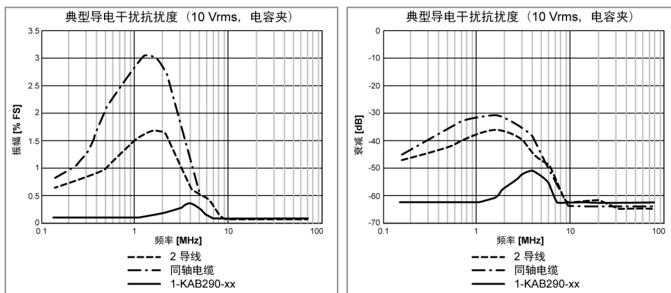
图 1.14: 典型传导抗扰度 , 使用 ± 10 V 量程测试
