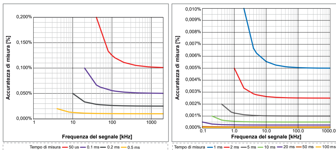
Figura 26: Incertezza di misura massima timer
