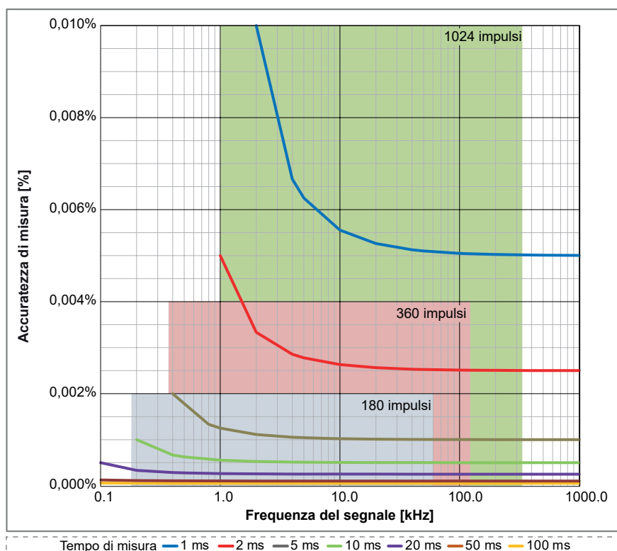
Figura 28: Campo operativo trasduttore numero di giri rispetto all'incerteza di misura e al tempo di misura
