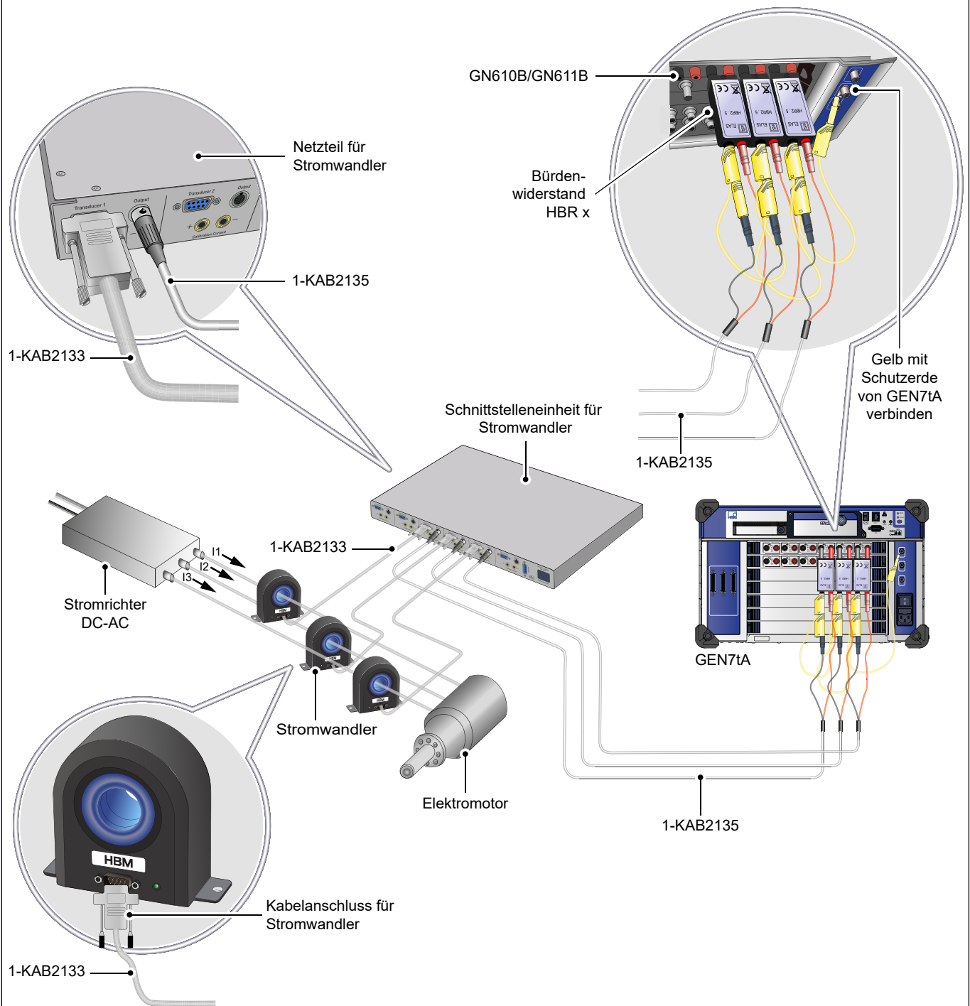
Abbildung 1.9: Anschlussdiagramm des Stromwandlers (CT)
