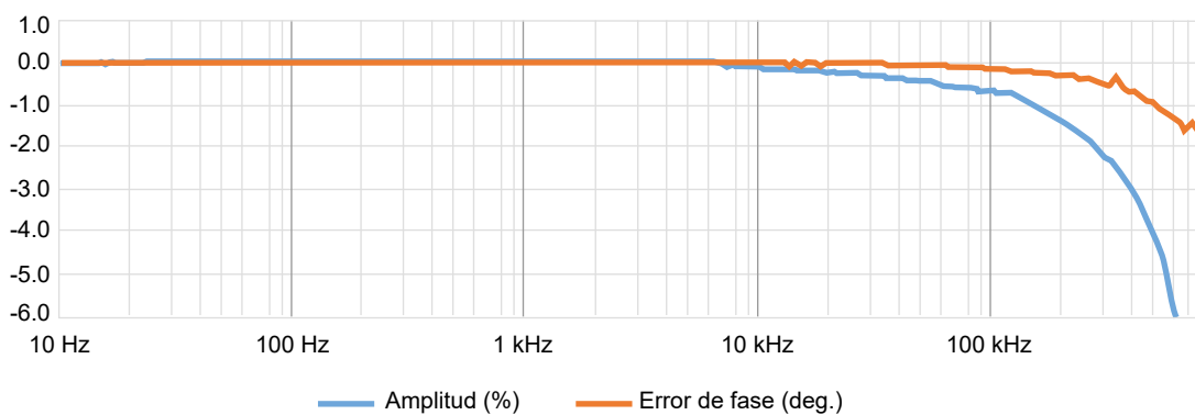
Figura 1.3: Características de frecuencia
