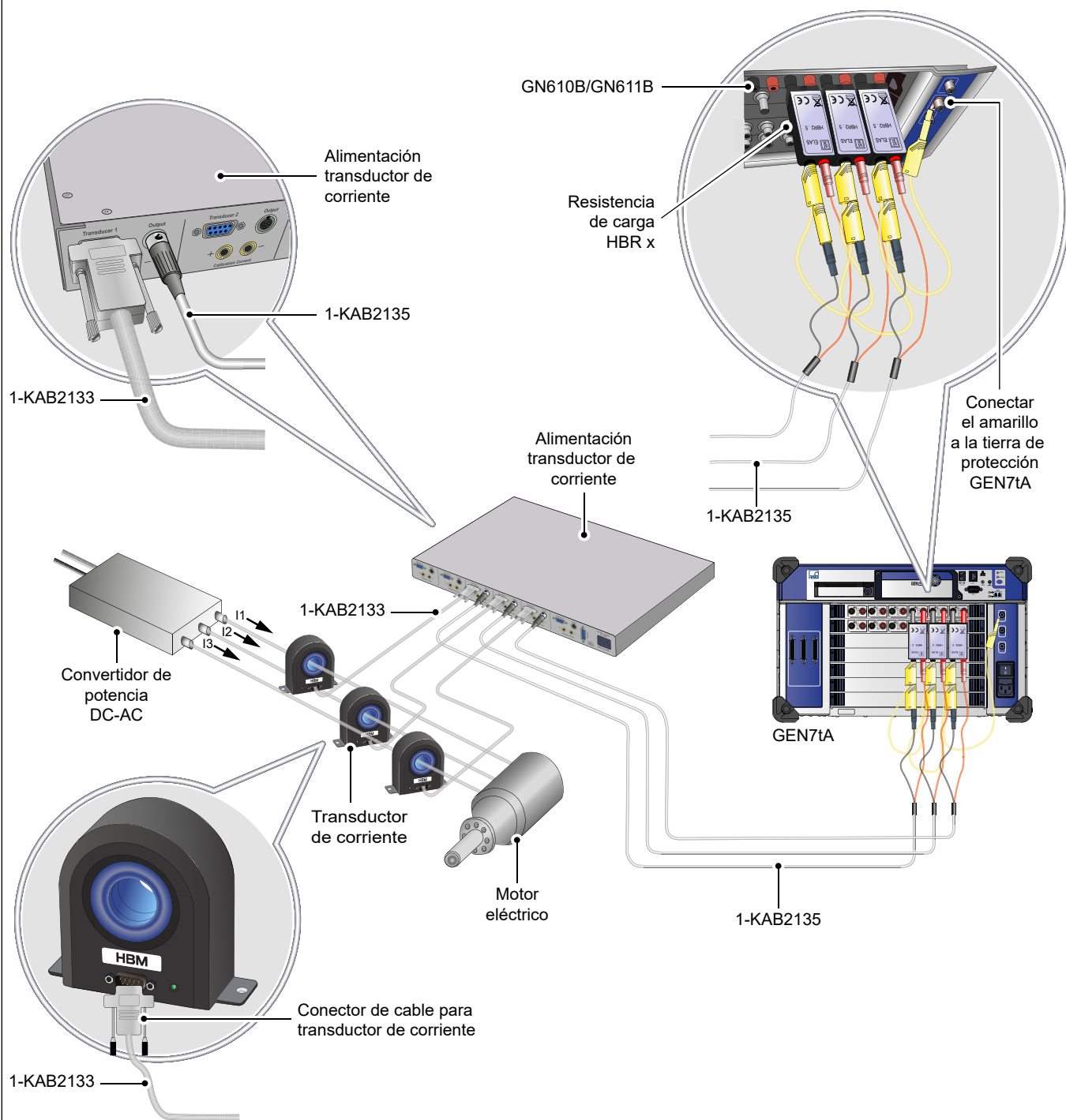
Figura 1.9: Diagrama de conexiones del transductor de corriente
