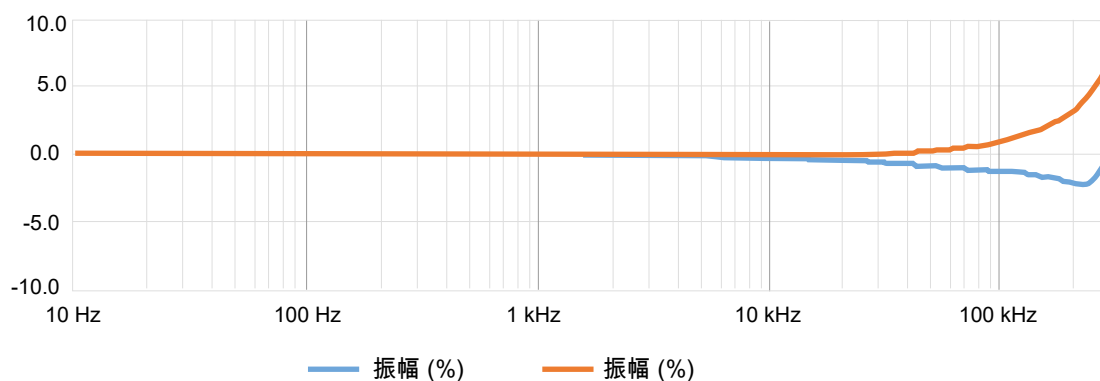
図 1.3: 周波数特性
