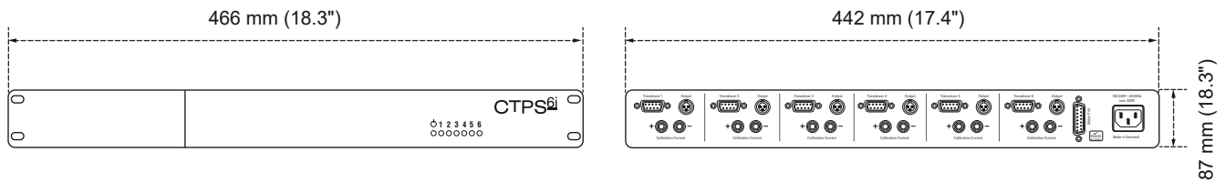
図 1.7: 寸法
