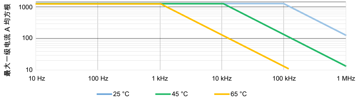
図 1.2: 周波数および周囲温度のディレーティング
