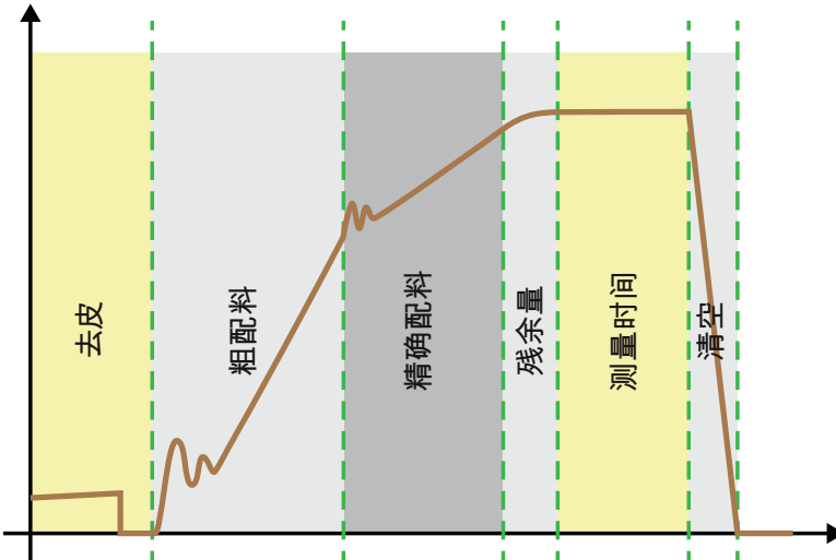
Fig. 6.2 灌装入秤
