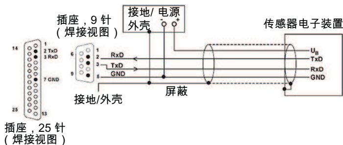
Fig. 4.6 串行接口（9 针和 25 针插座的标准分配）接线图（使用同一电缆供电）。
