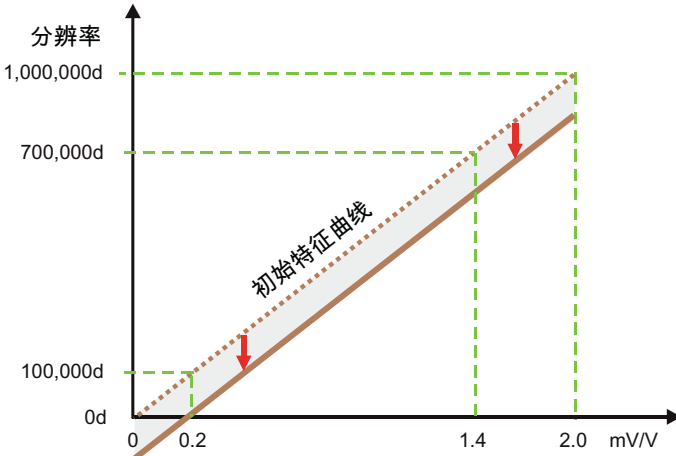
Fig. 5.1 测量操作对特征曲线的影响。
