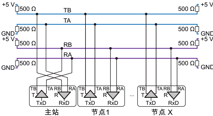
Fig. 4.8 RS-485 接口接线图
