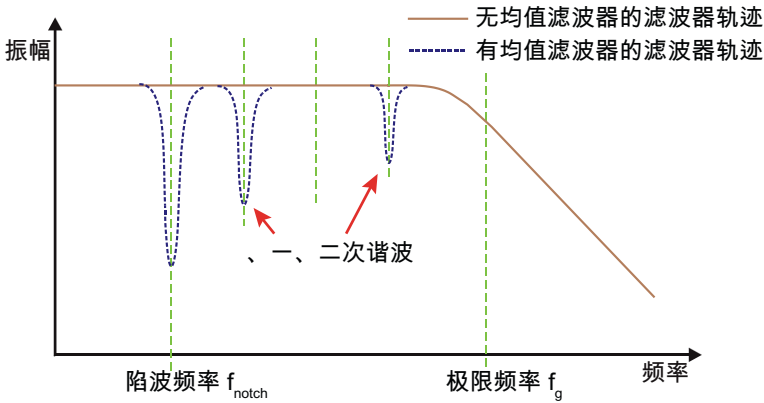
Fig. 7.12 陷波滤波器的频率响应。
