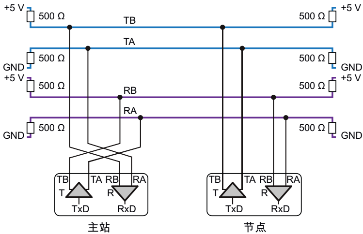
Fig. 4.7 RS-422 接口接线图
