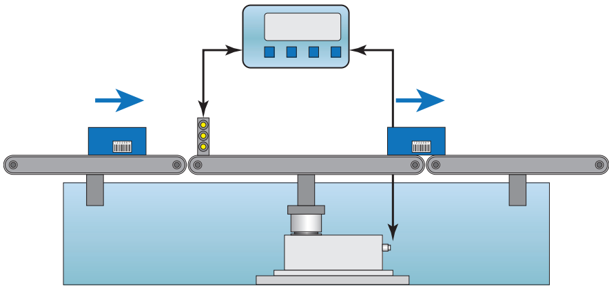
Fig. 6.4 检重秤原理
