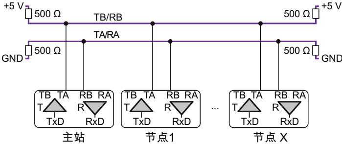
Fig. 4.9 二线制配置下的 RS-485 接口接线图
